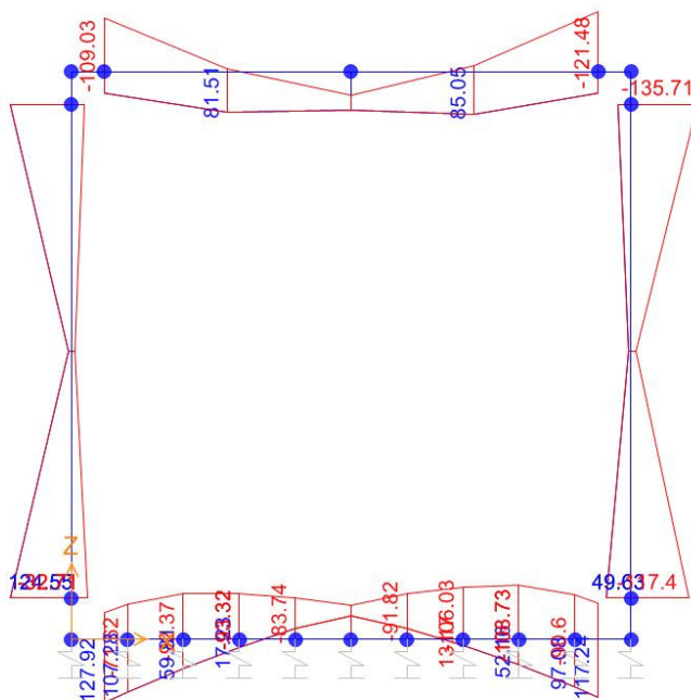
Momento Flettente
