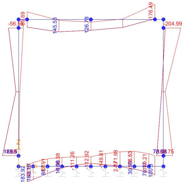
Momento Flettente
