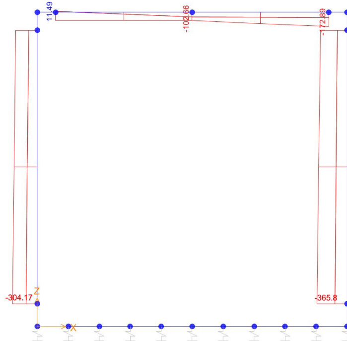
Sforzo normale
