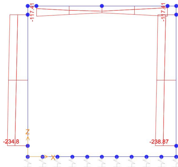
Sforzo normale
