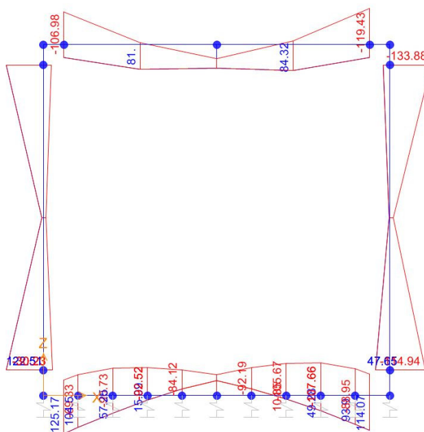
Momento Flettente
