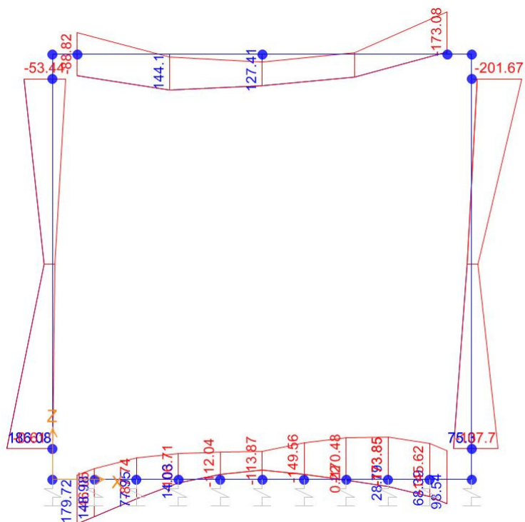
Momento Flettente
