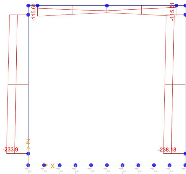
Sforzo normale
