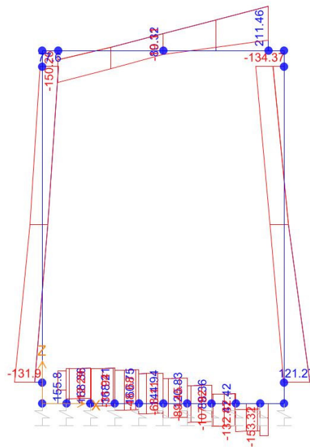
Taglio
