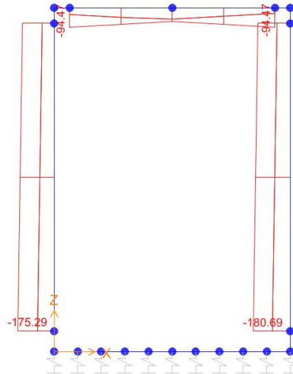
Sforzo normale
