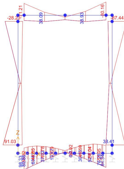
Momento Flettente
