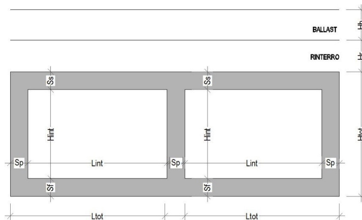
Figura 2. Sezione trasversale dello scatolare
