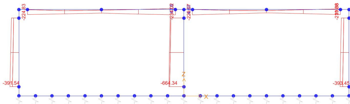
Sforzo normale
