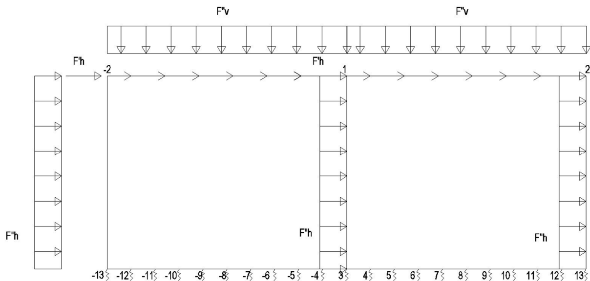
Figura 9. Forze sismiche agenti sulla struttura
