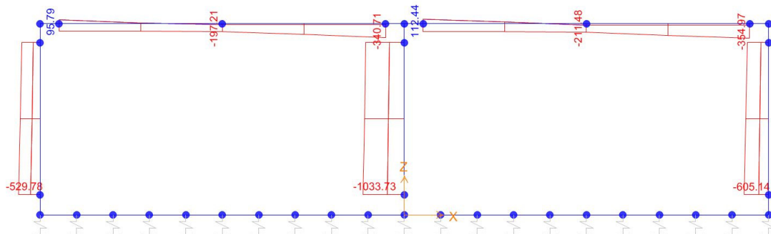
Sforzo normale
