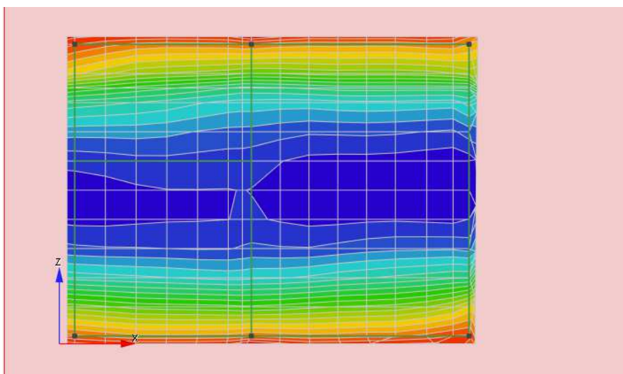
Figura 7-5 – Sollecitazioni flettenti M_{zz} SLV.
