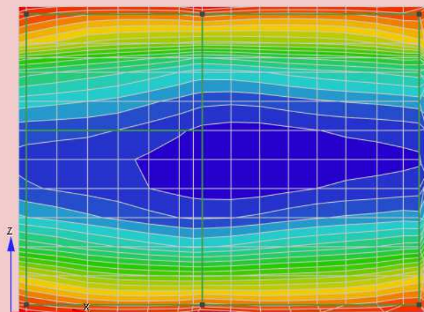
Figura 7-3 – Sollecitazioni flettenti M_{zz} SLU.
