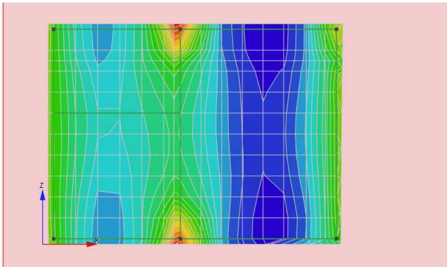
Figura 7-4 – Sollecitazioni flettenti M_{xx} SLV.
