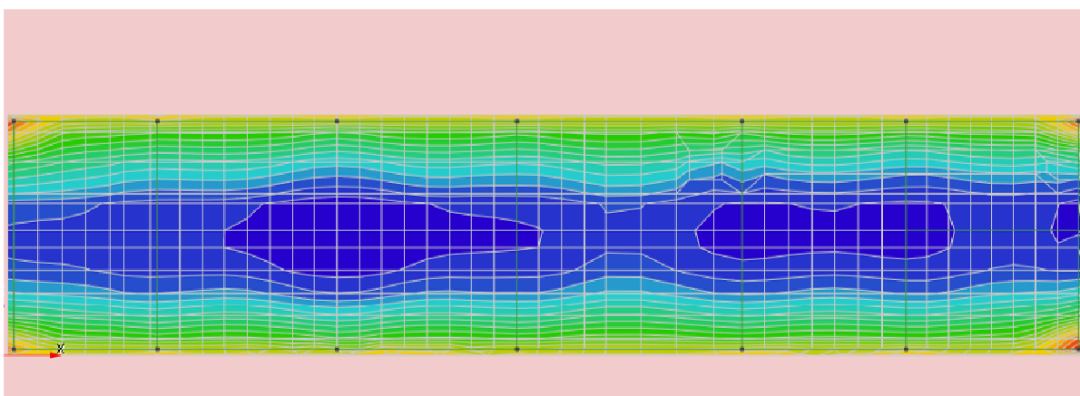
Figura 7-5 – Sollecitazioni flettenti Mzz SLV.
