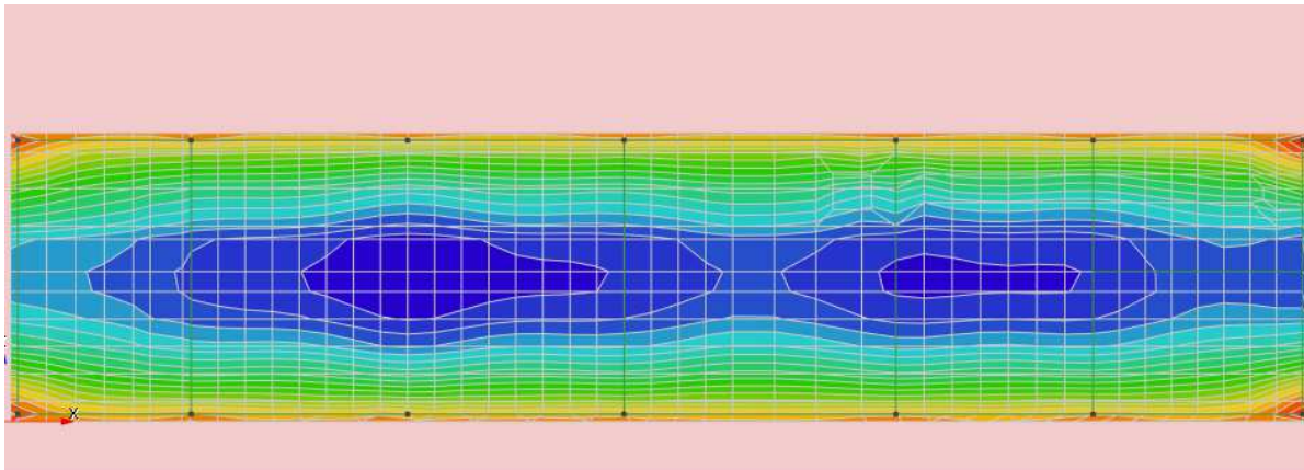
Figura 7-3 – Sollecitazioni flettenti Mzz SLU.
