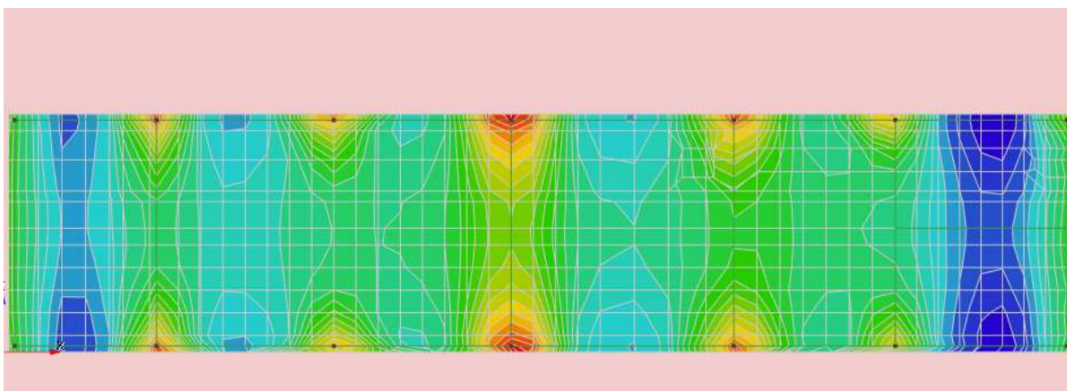
Figura 7-4 – Sollecitazioni flettenti Mxx SLV.
