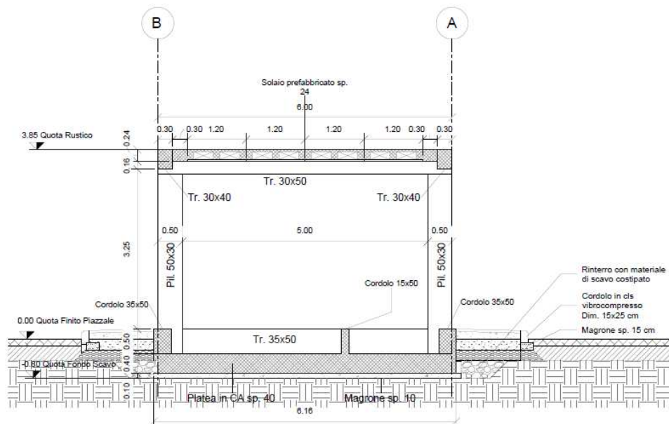
Sezione STR B-B' 1 : 50
