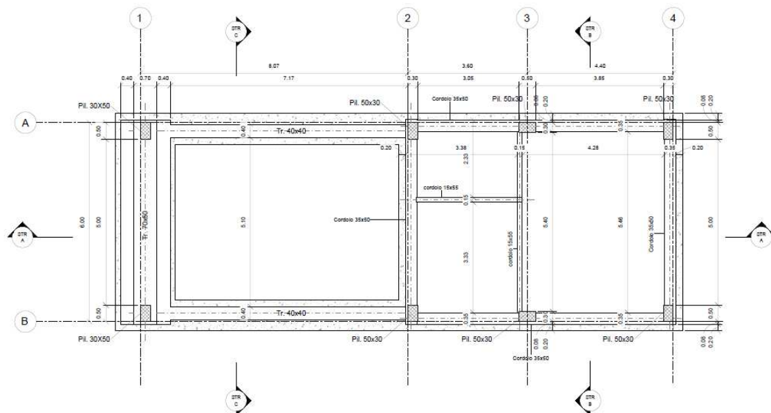
Carpenteria Fondazione 1 : 50
