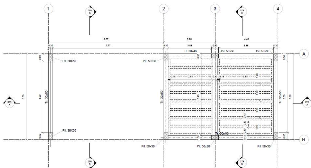
Carpenteria Copertura 1 : 50
