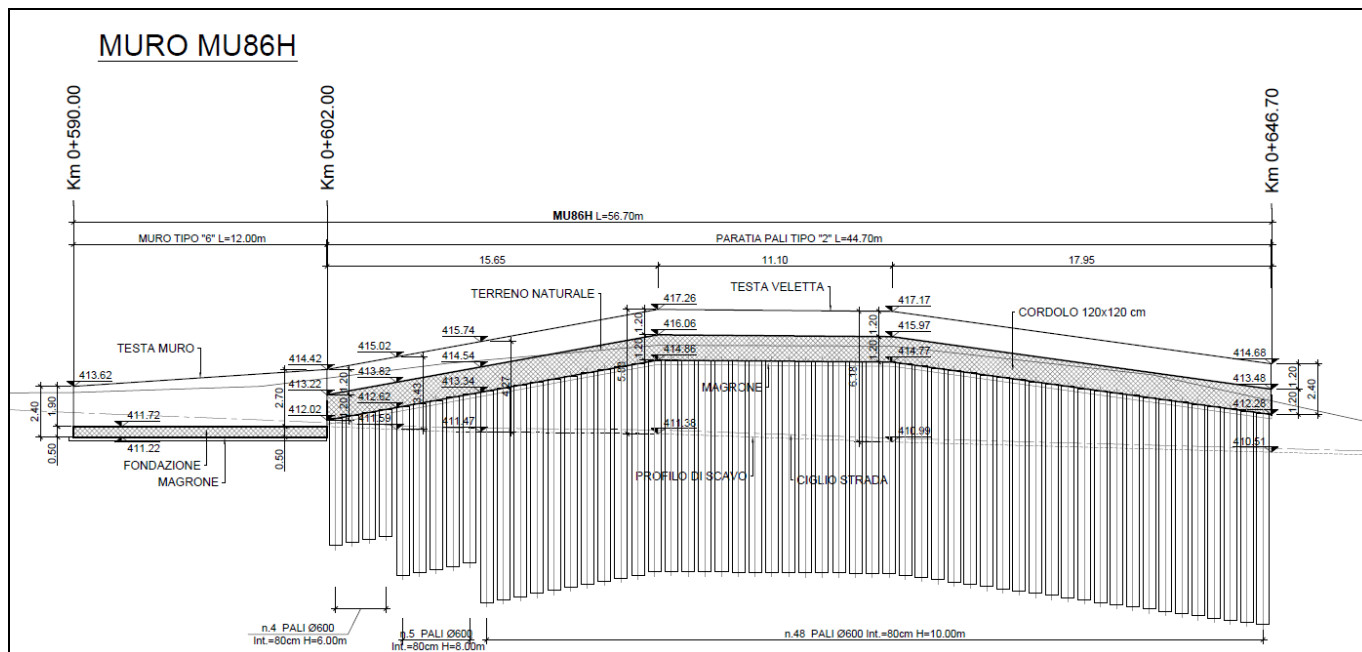
Figura 1-2 – Profilo MU86H.
