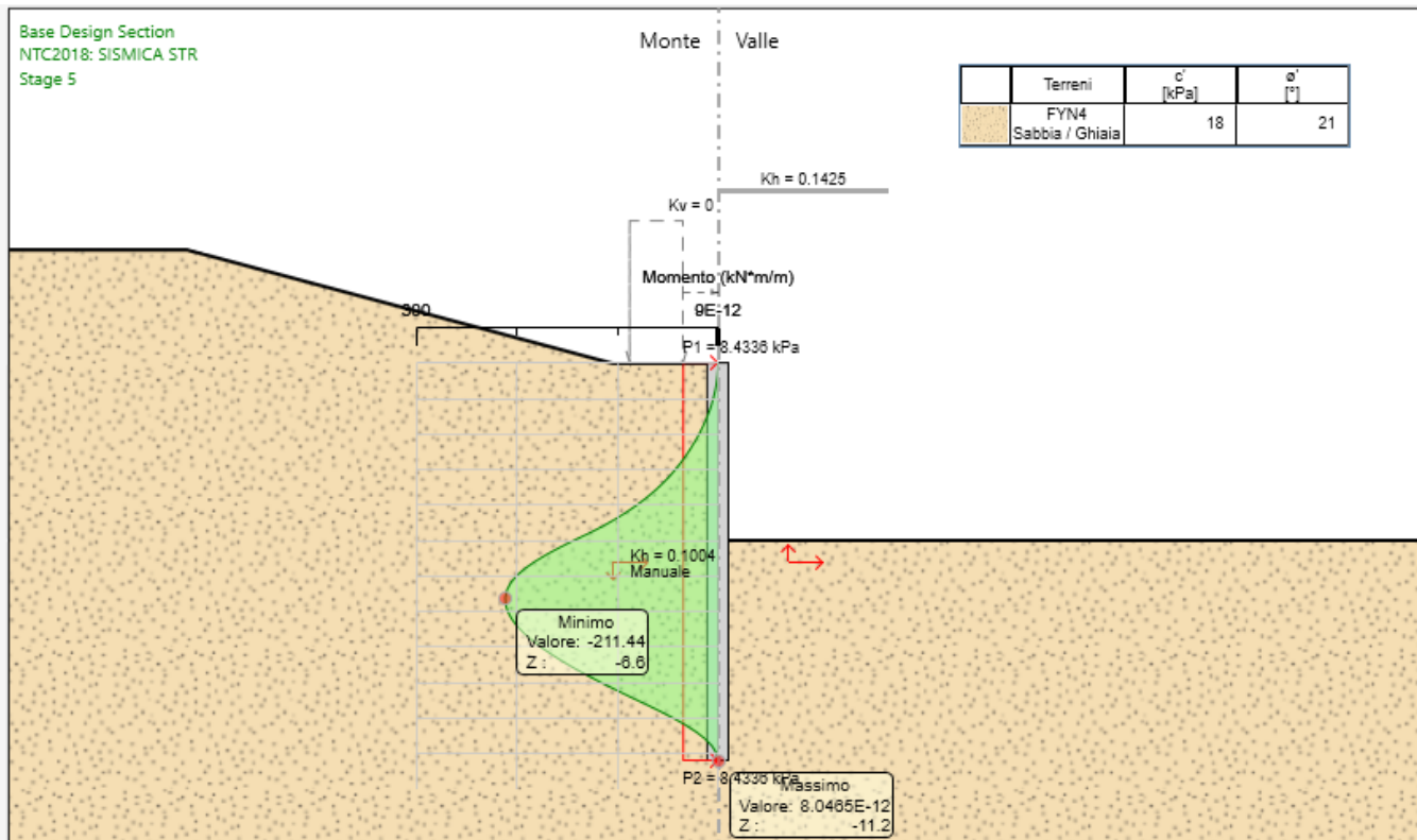
Figura 12-5 – Momento SLV.
