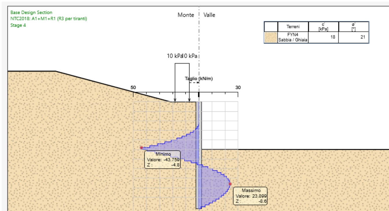
Figura 12-4 – Taglio SLU.
