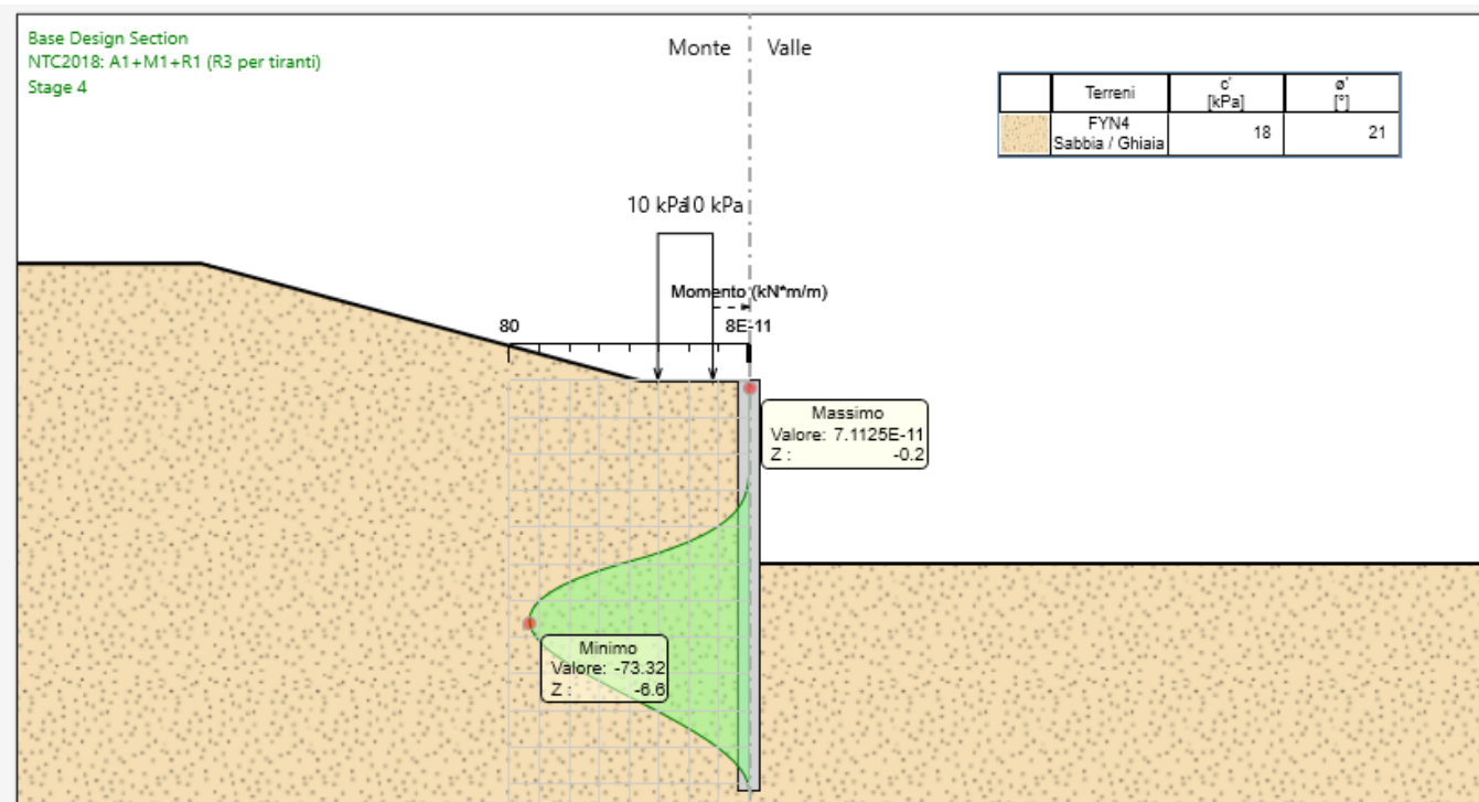
Figura 12-3 – Momento SLU.
