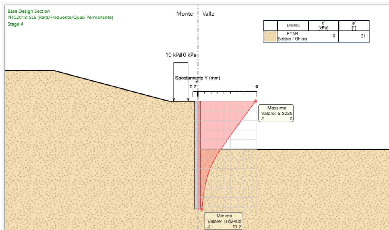
Figura 12-7 – Deformata dell'opera di sostegno nella configurazione di fondo scavo.
