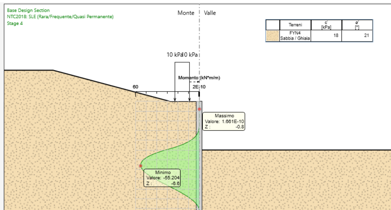
Figura 12-2 – Momento SLE.
