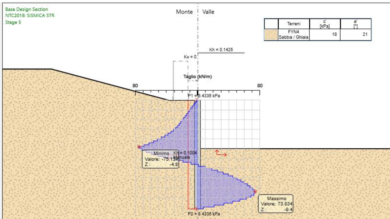
Figura 12-6 – Taglio SLV.
