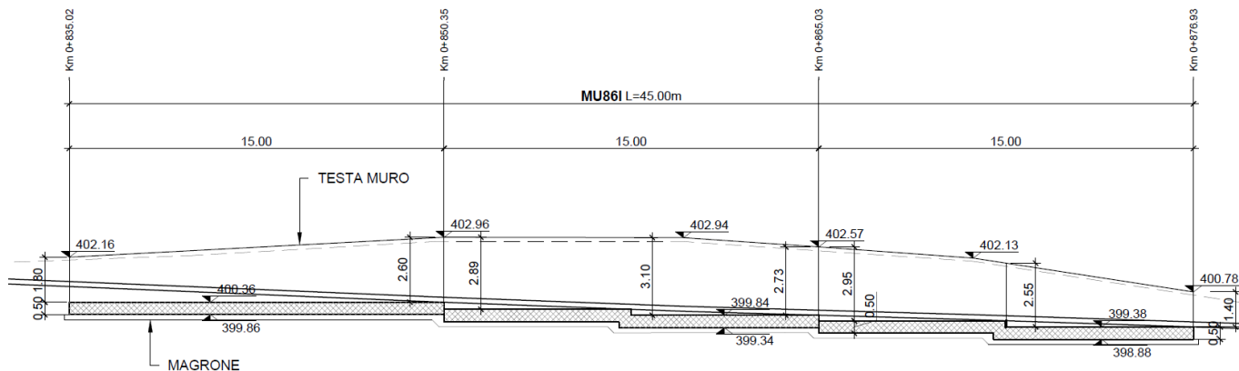
Figura 1-2 –Profilo MU861.
