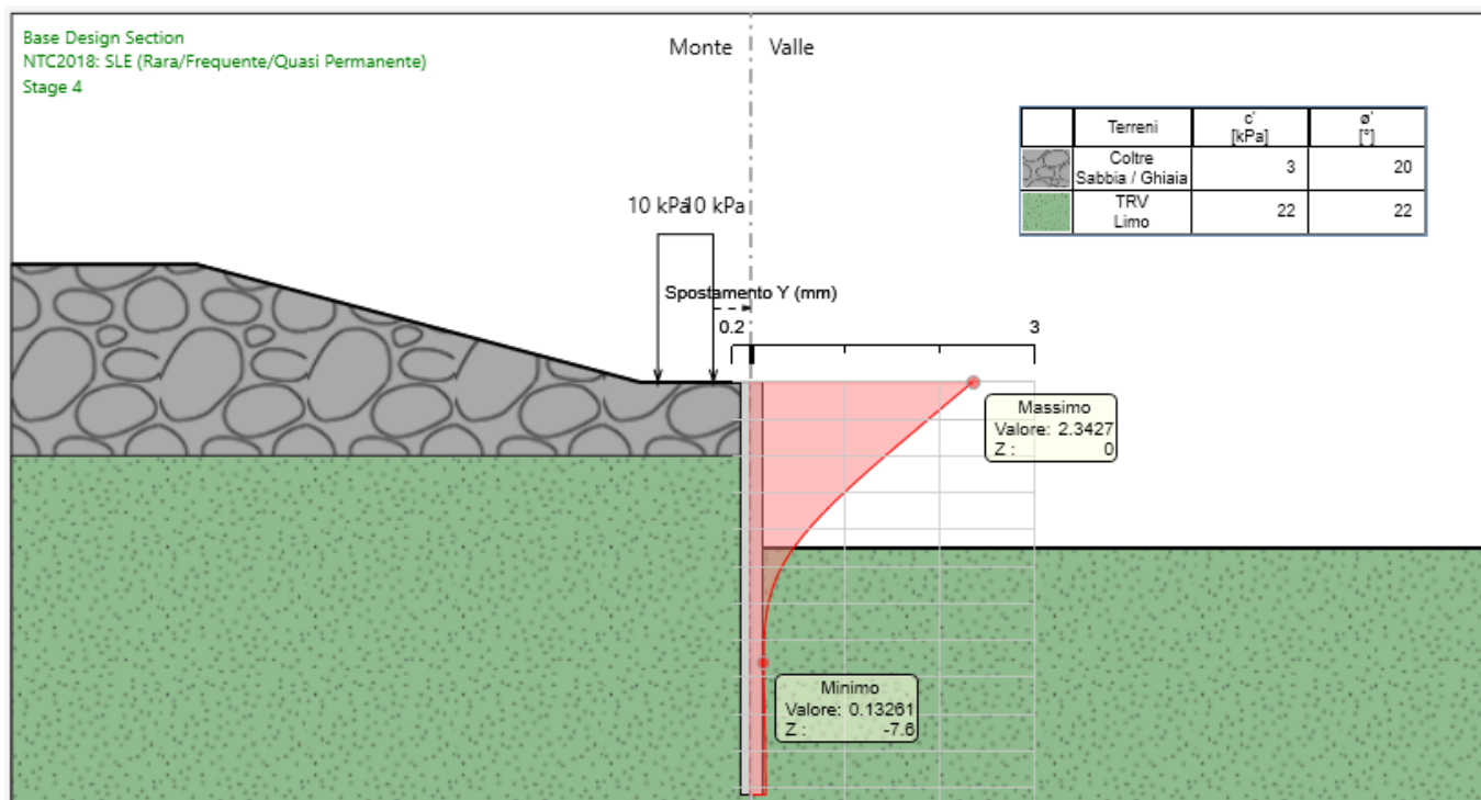
Figura 13-7 – Deformata dell'opera di sostegno nella configurazione di fondo scavo.
