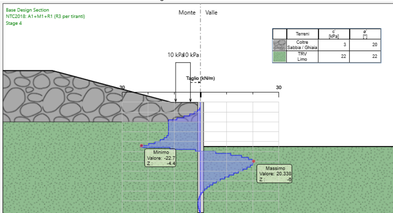
Figura 13-4 – Taglio SLU.
