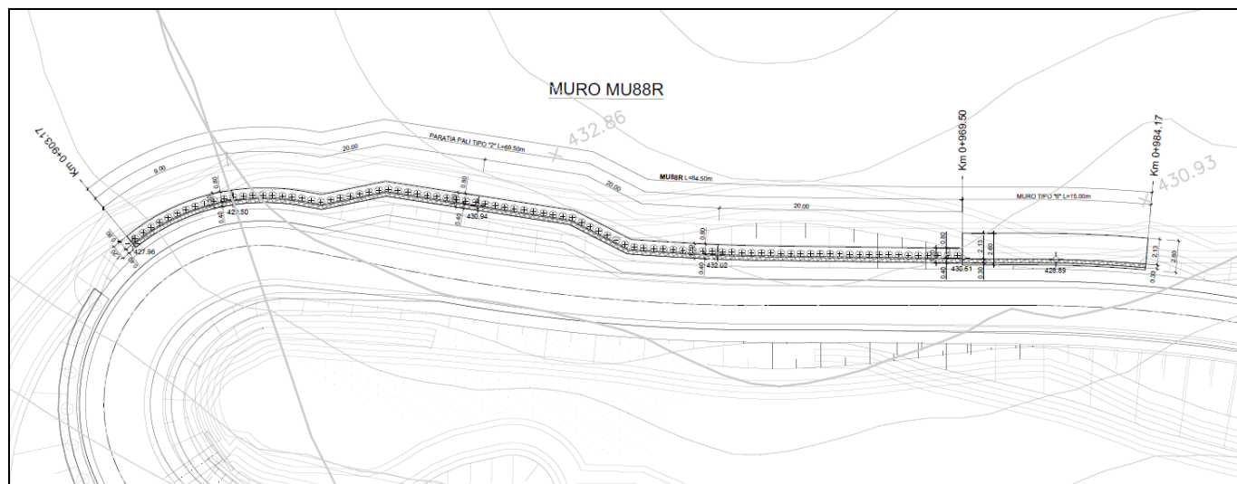
Figura 1-1 – Pianta MU88R.
