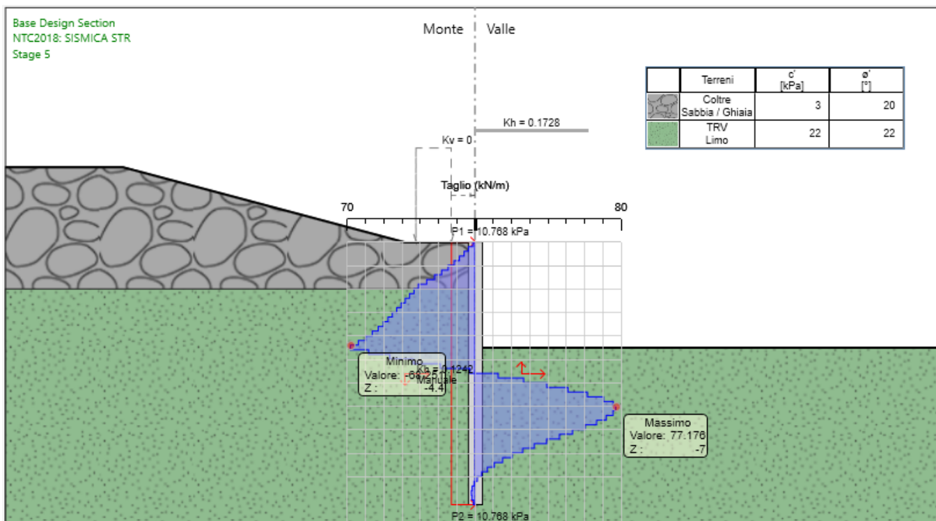
Figura 13-6 – Taglio SLV.
