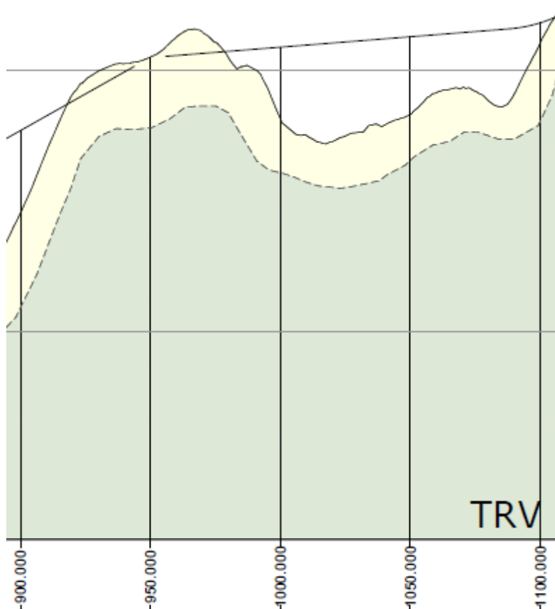
Figura 6-1 – Stralcio del profilo geotecnico.
