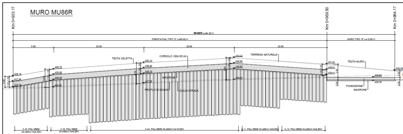
Figura 1-2 – Prospetto MU88R.
