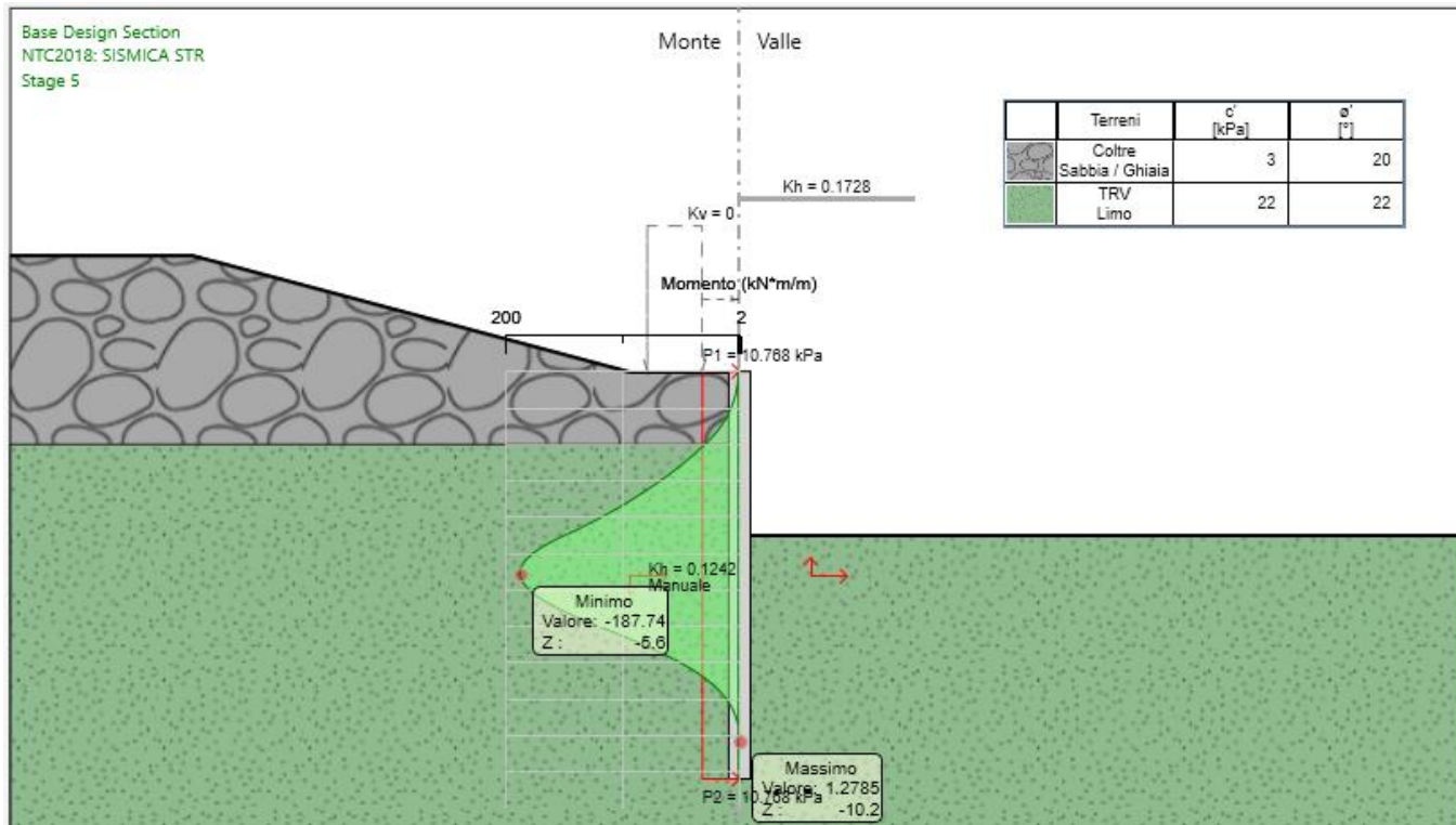
Figura 13-5 – Momento SLV.
