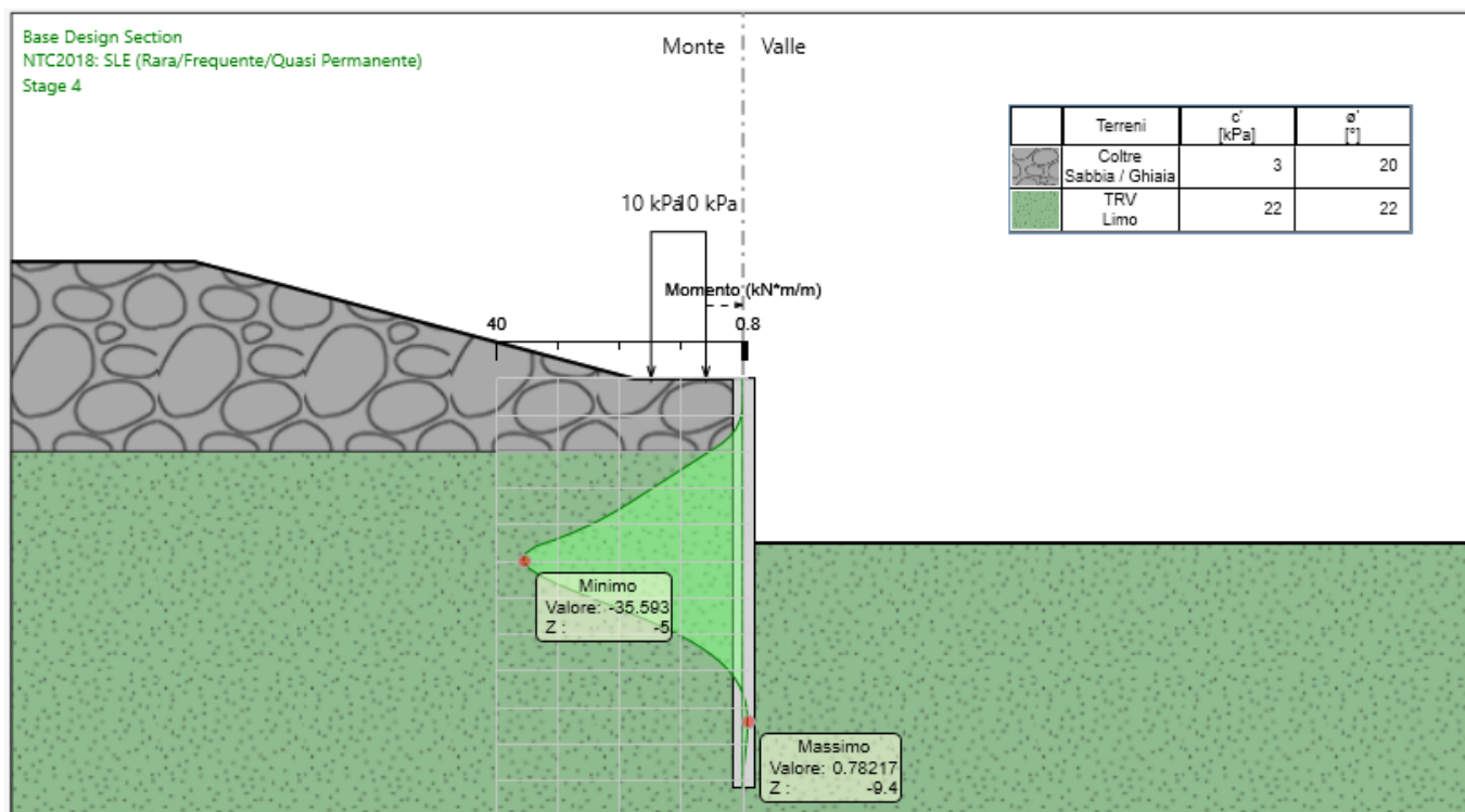
Figura 13-2 – Momento SLE.
