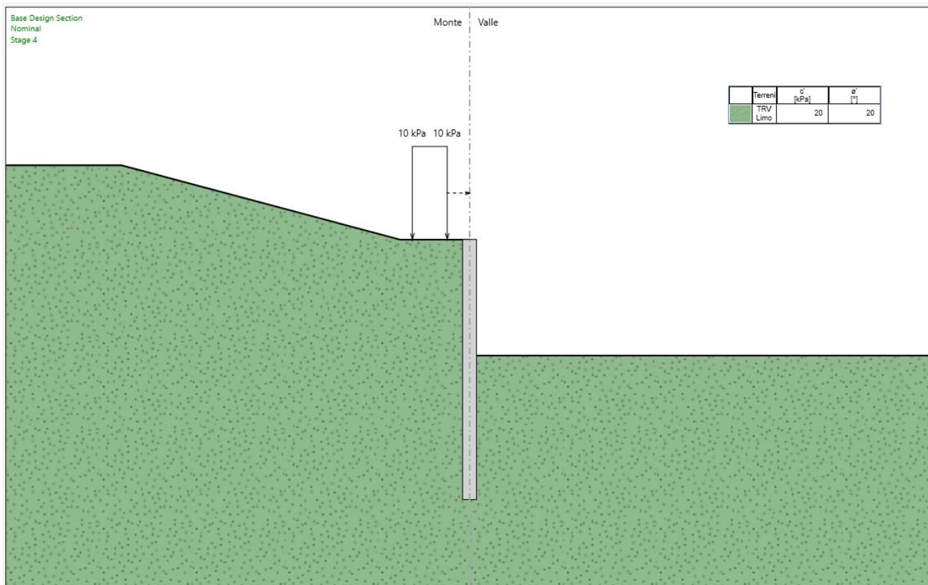
Figura 13-1. Schema di calcolo paratia
