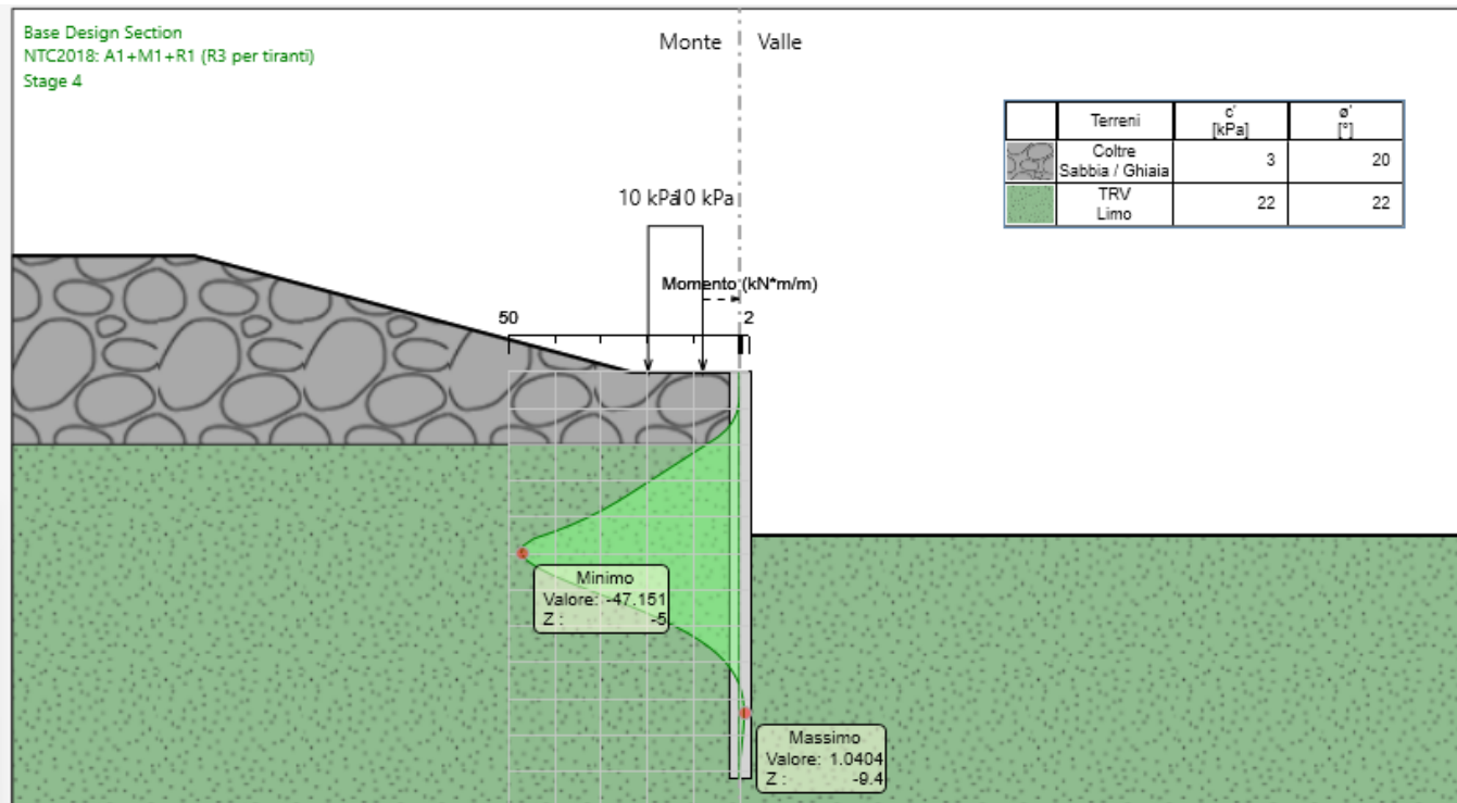
Figura 13-3 – Momento SLU.
