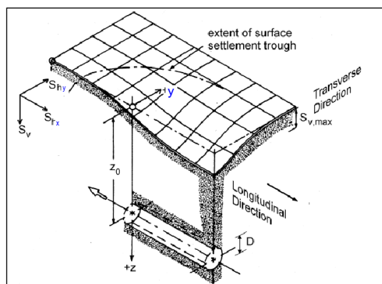
Figura 1 - Movimenti indotti in superficie dall'avanzamento di uno scavo sotterraneo (dopo Attewell et Al., 1986, Mair, Taylor 1997)
