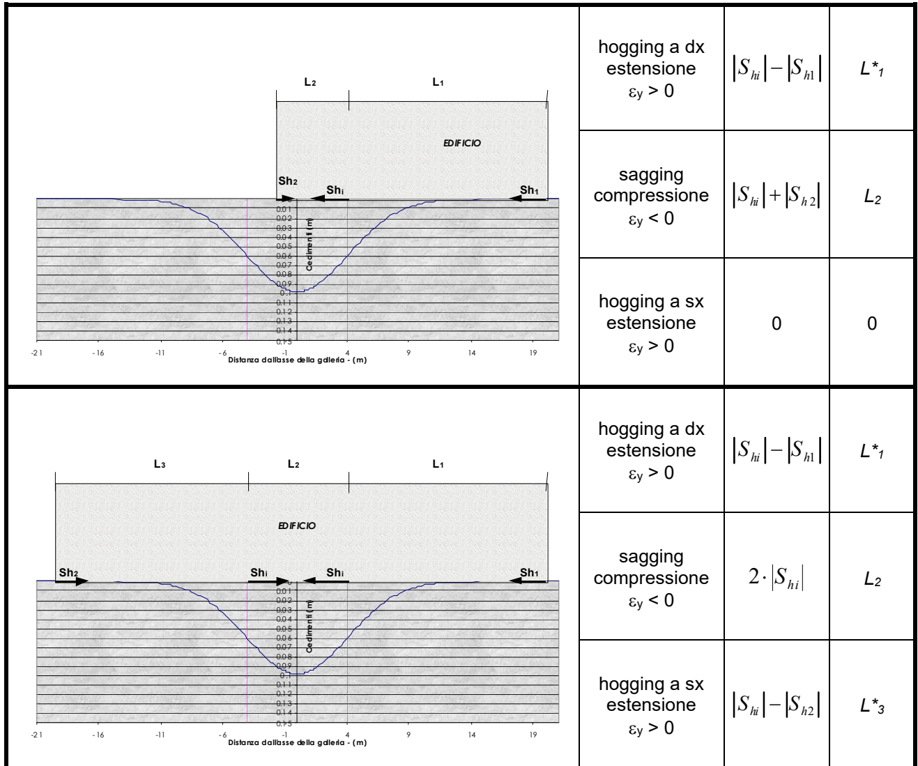
Figura 7 - Schemi di riferimento per la definizione del parametro \Delta Sh (2/3)
