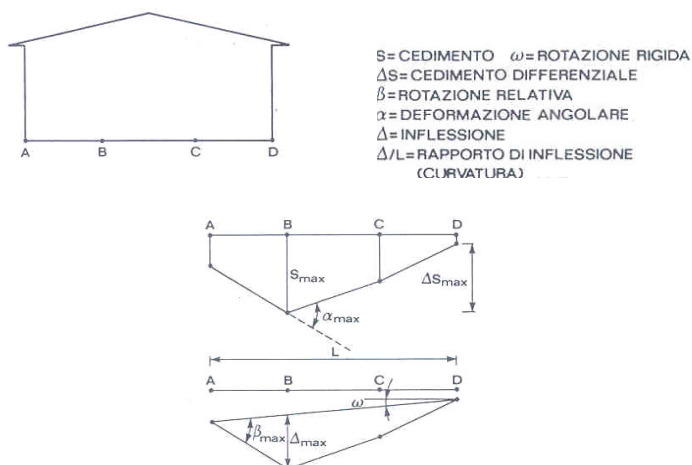
Figura 5 - Principali parametri per la definizione del danneggiamento degli edifici per fondazioni a plinti
