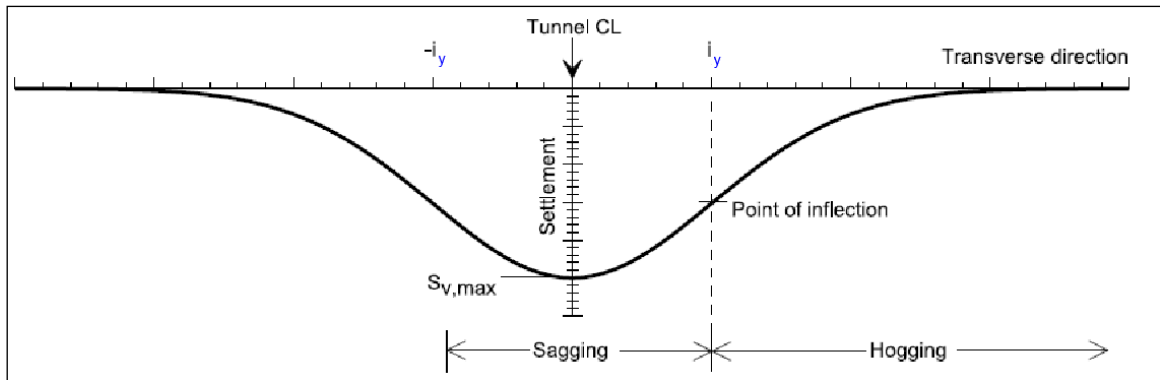
Figura 2 - Profilo trasversale di subsidenza (Mair, Taylor 1997)
