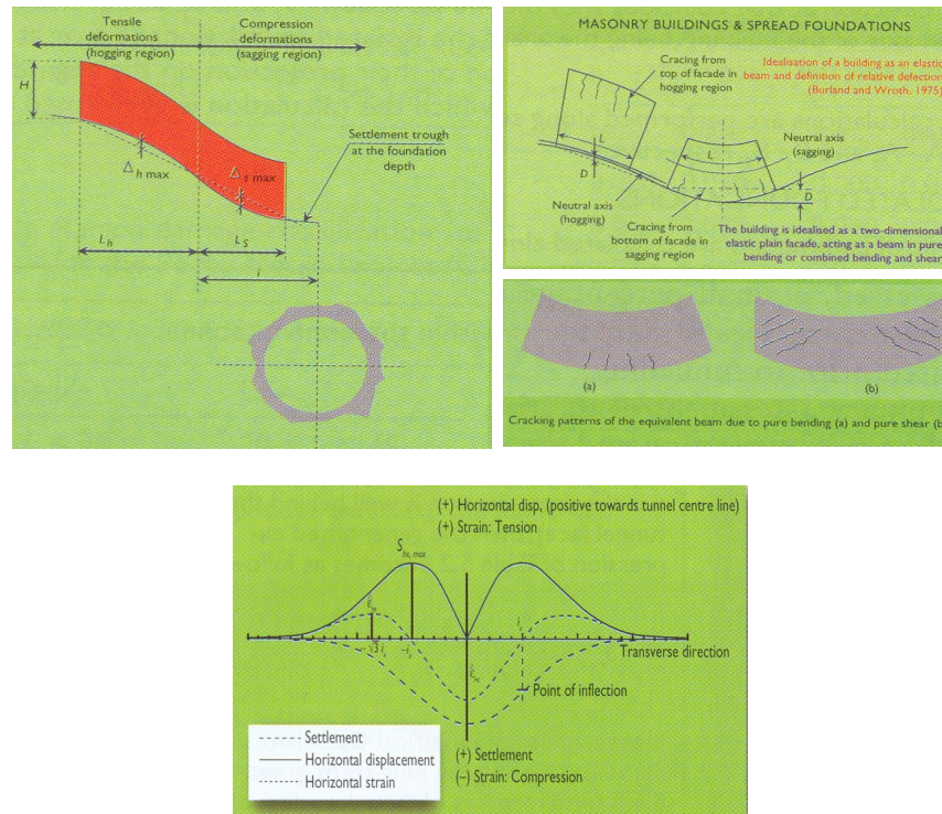
Figura 4 - Suddivisione della curva di subsidenza nelle componenti “hogging” e “sagging”
