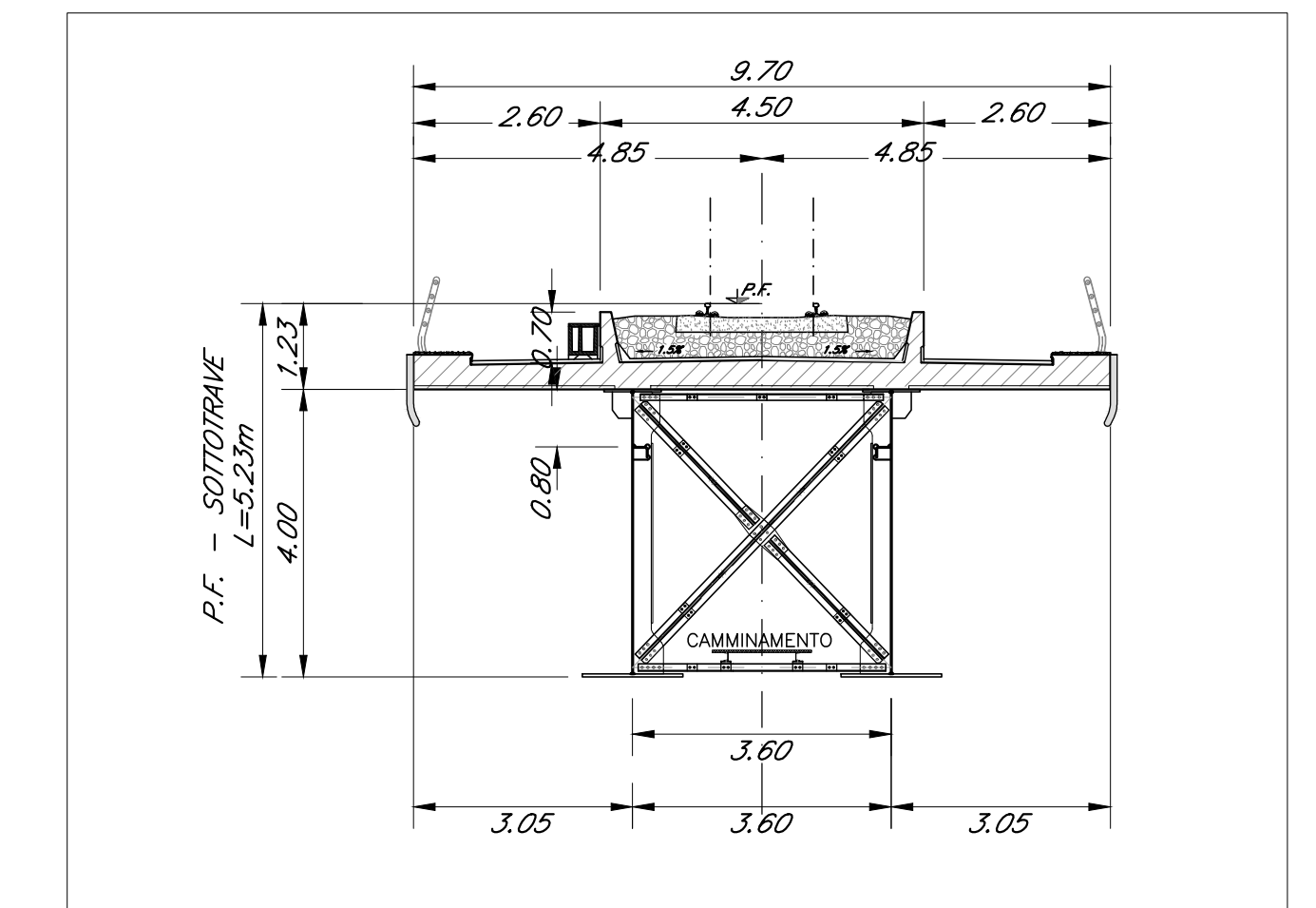
SEZIONE TIPO ACCIAIO 50M Scala 1:100
