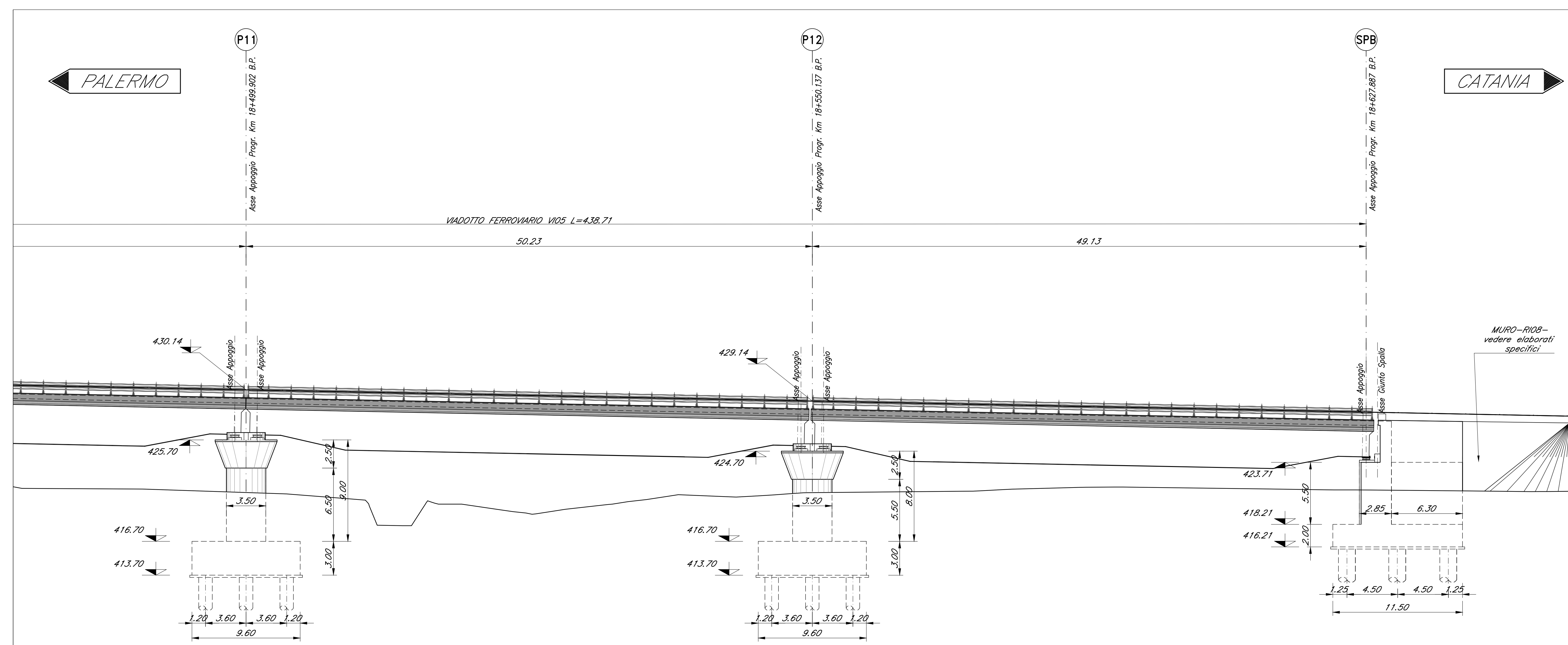
PROSPETTO BINARIO PARI Scala 1:200
