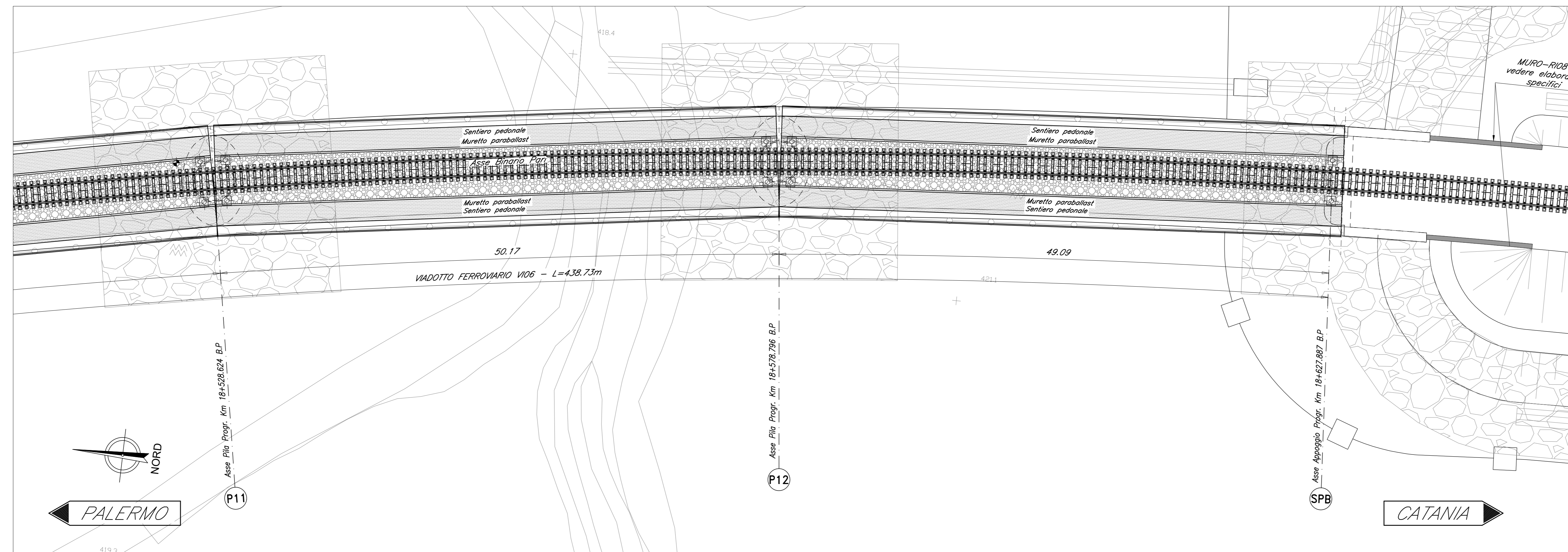
PROSPETTO BINARIO PARI Scala 1:200
