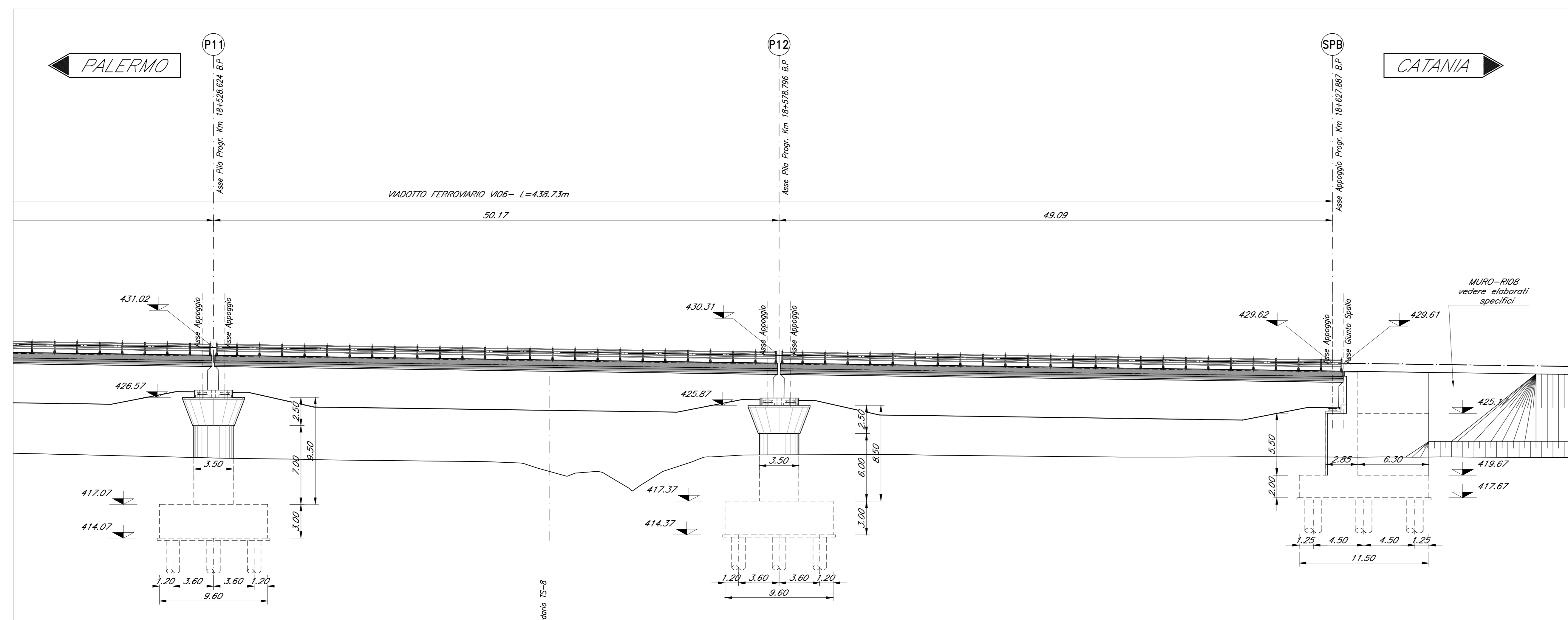
PROSPETTO BINARIO PARI Scala 1:200
