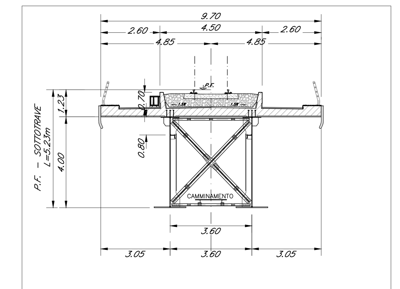
SEZIONE TIPO ACCIAIO 50M Scala 1:100
