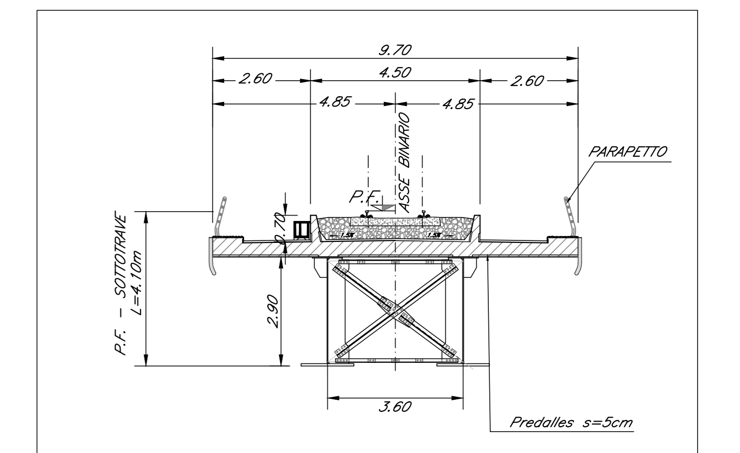
SEZIONE TIPO ACCIAIO 40M Scala 1:100
