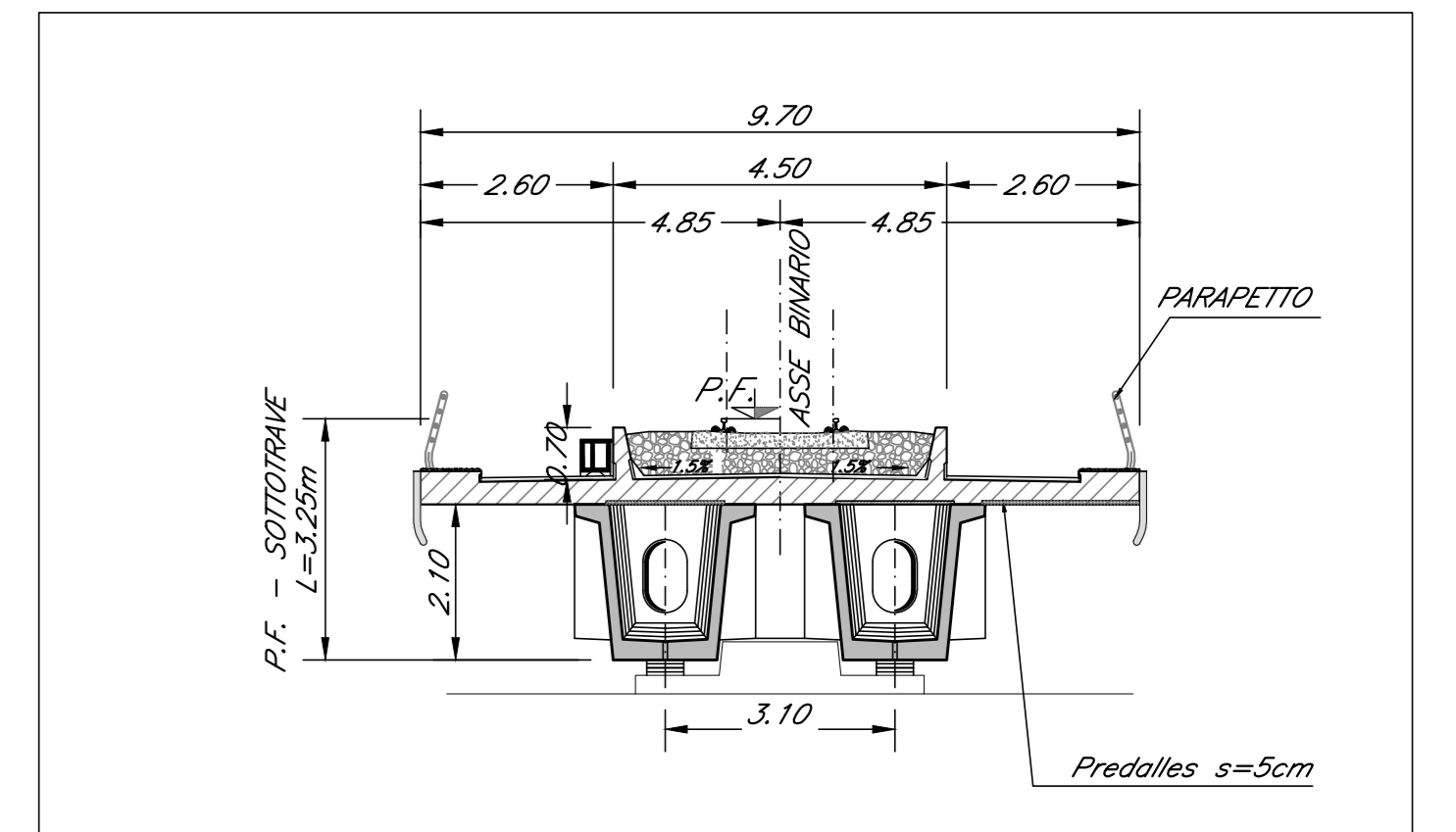
SEZIONE TIPO C.A.P. 25M Scala 1:100
