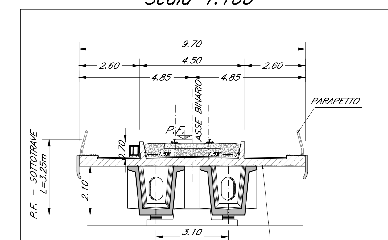
SEZIONE TIPO CAP 25M Scala 1:100
