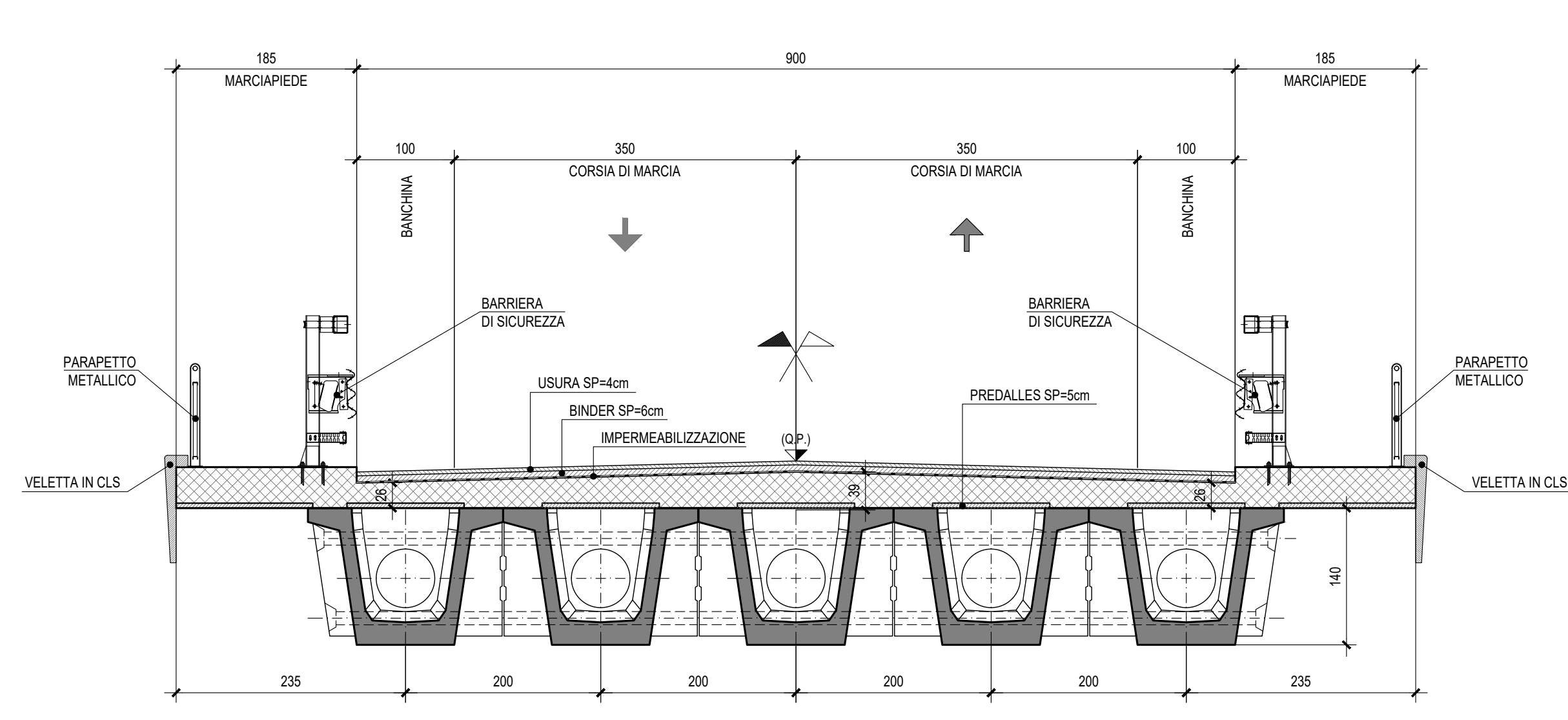
SEZIONE TRASVERSALE - Scala 1:50
