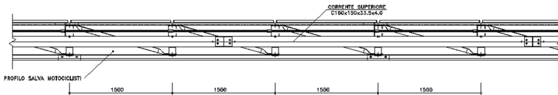
Vista laterale e dall'alto barriera ANAS H4 BLSM
