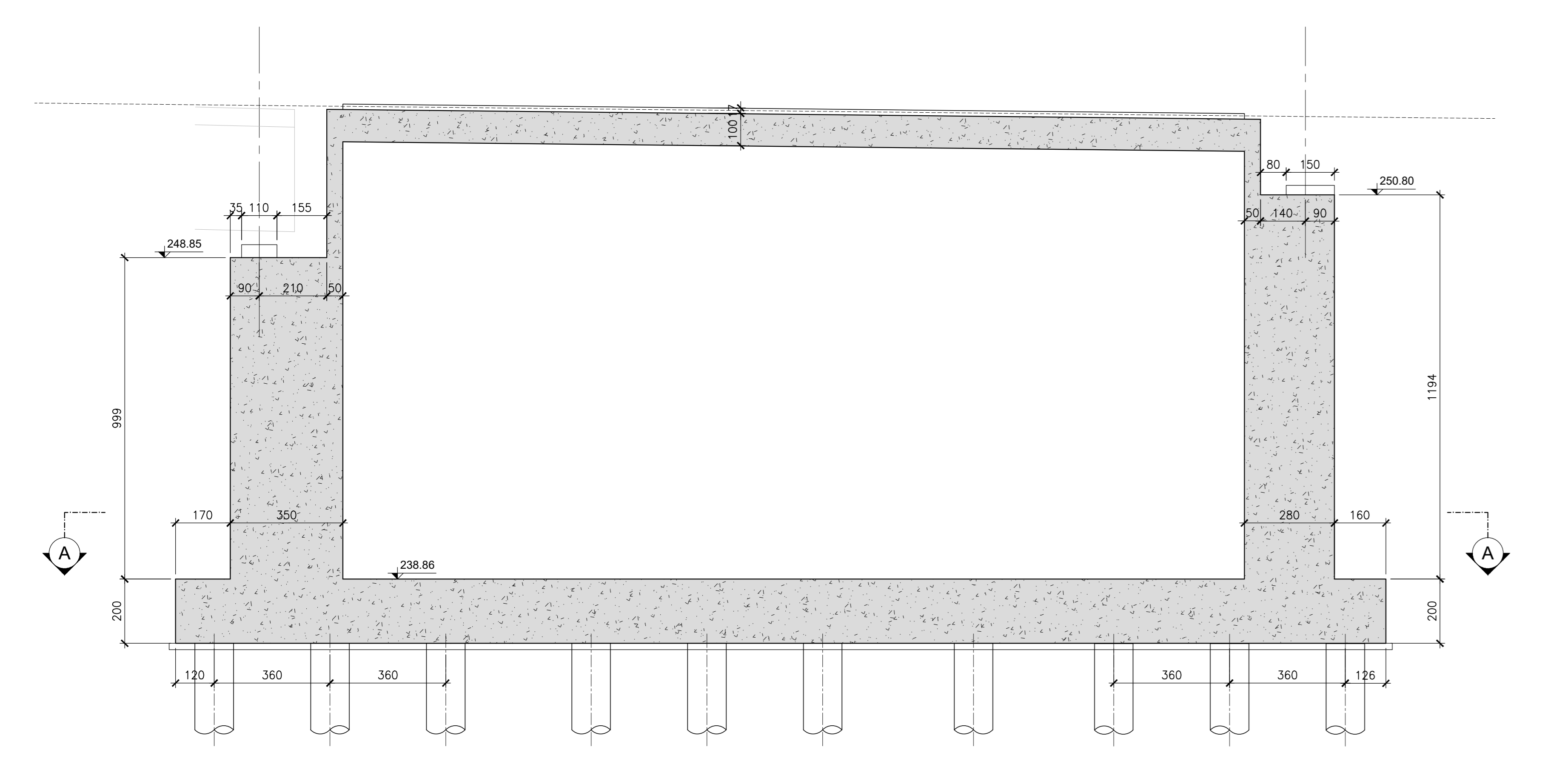
SEZIONE LONGITUDINALE D-D SCALA 1:100
