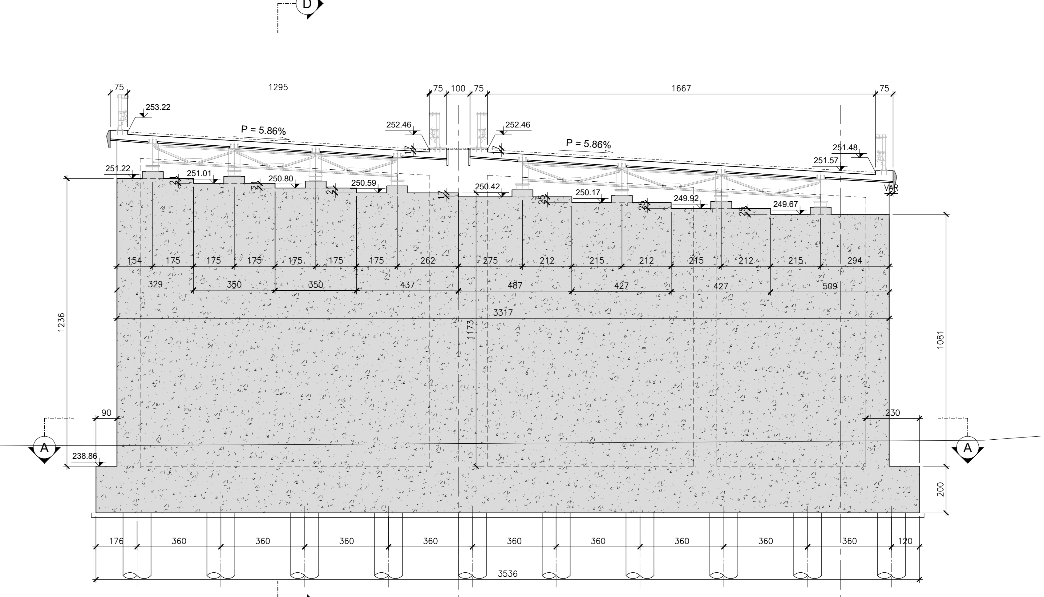
SEZIONE TRASVERSALE F-F (ASSE APPOGGIO) SCALA 1:100
