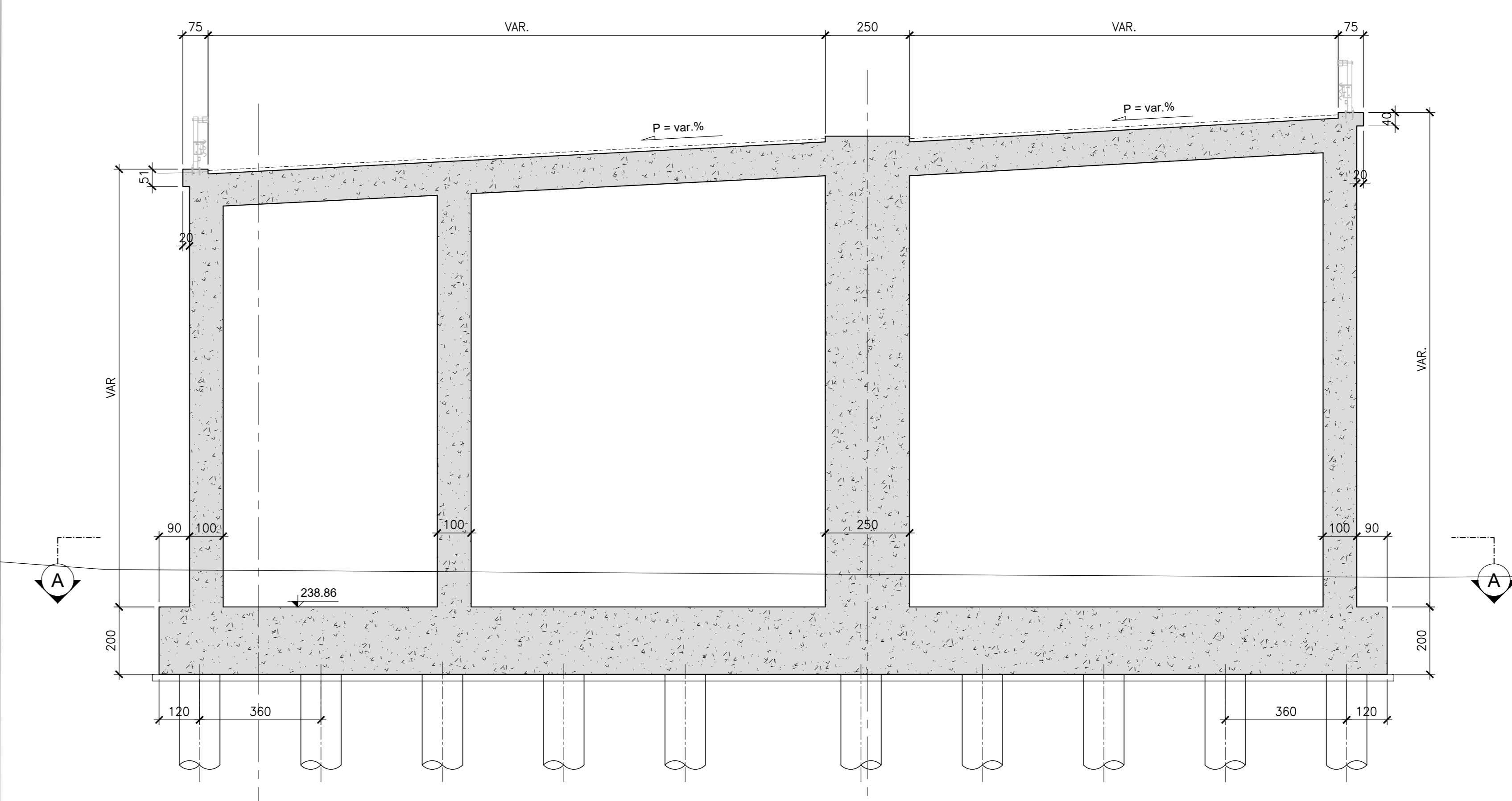
SEZIONE TRASVERSALE SCALA 1:100
