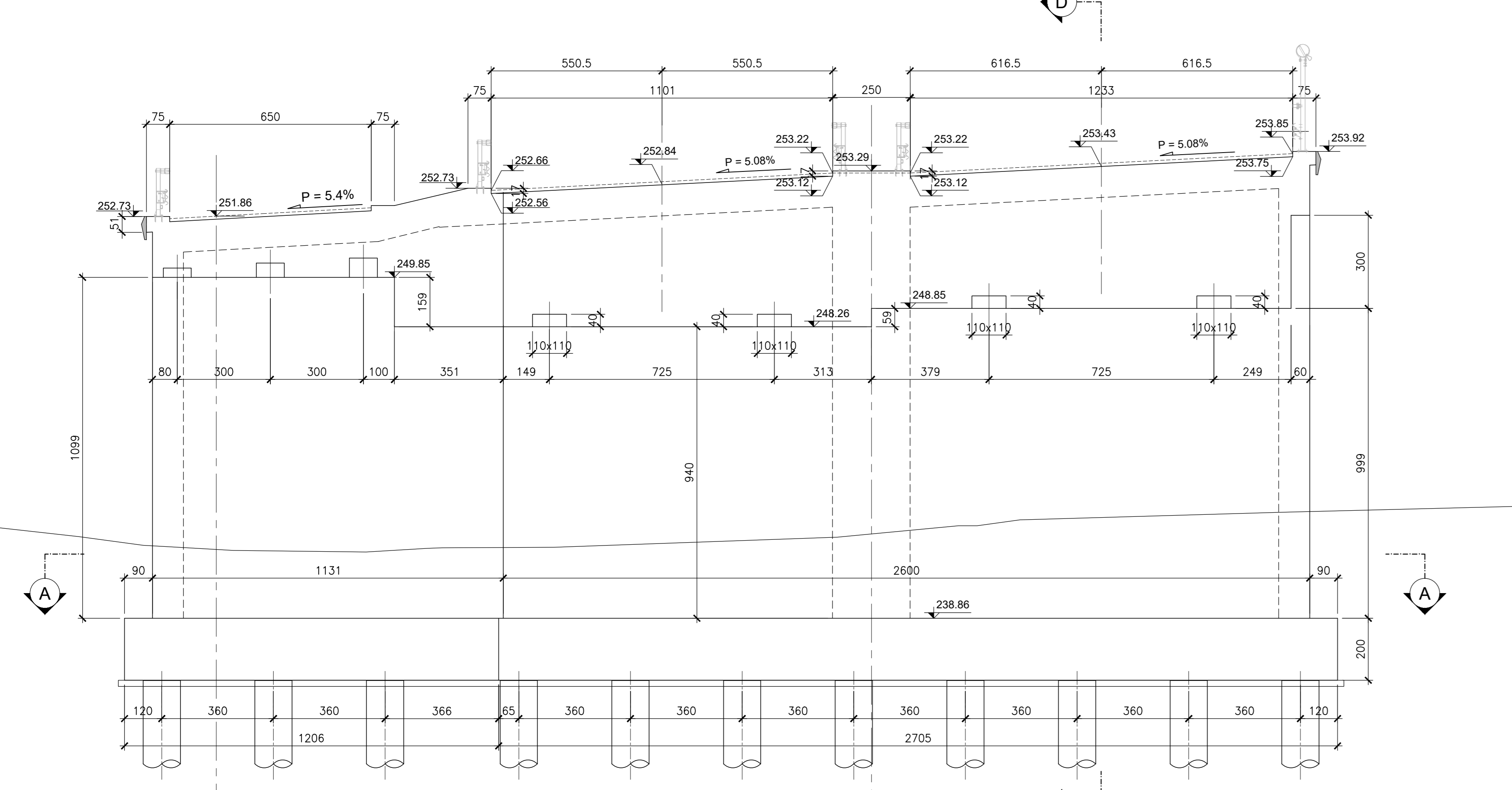
PROSPETTO FRONTALE B-B SCALA 1:100
