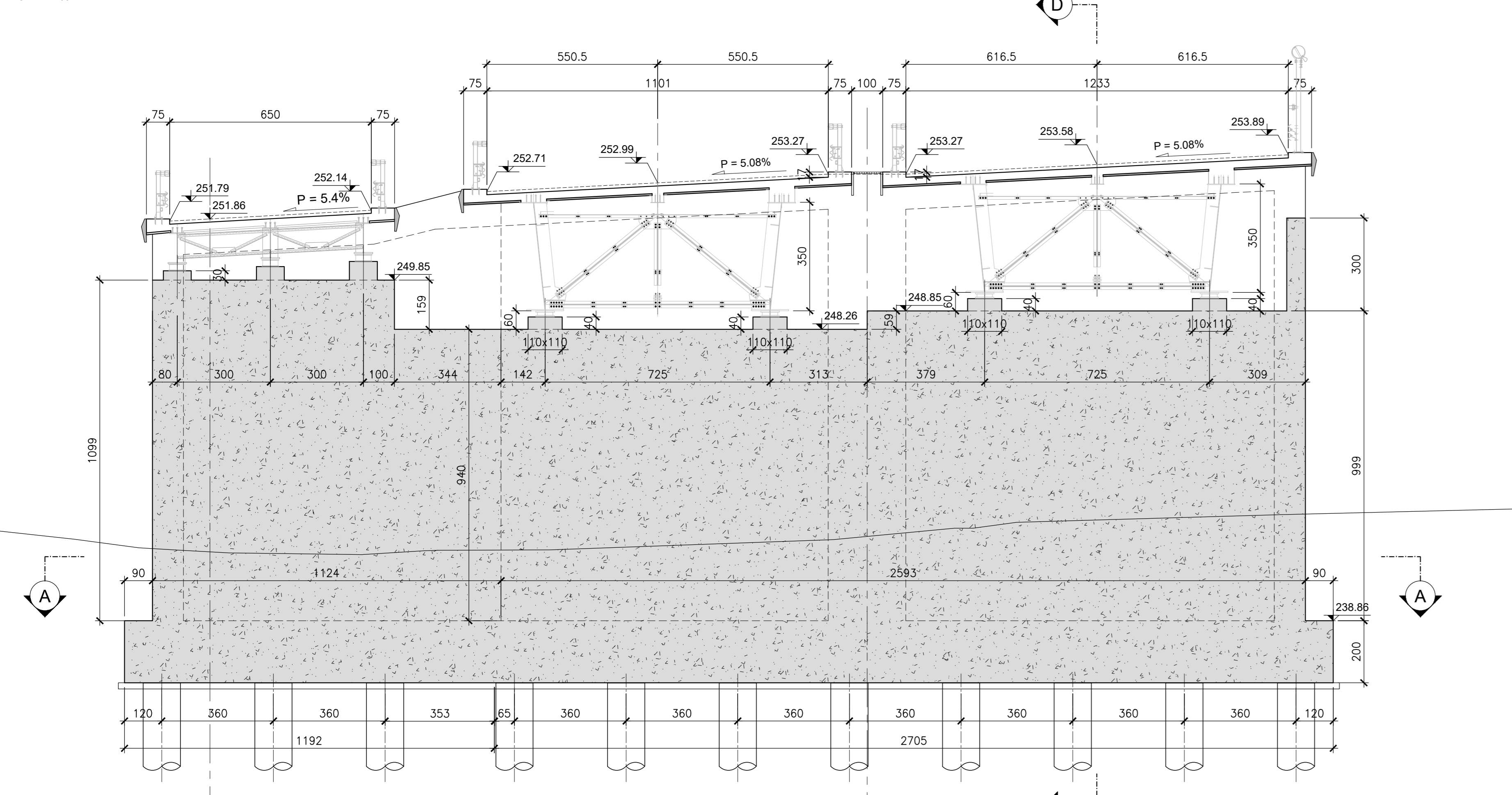
SEZIONE TRASVERSALE E-E (ASSE APPOGGIO) SCALA 1:100
