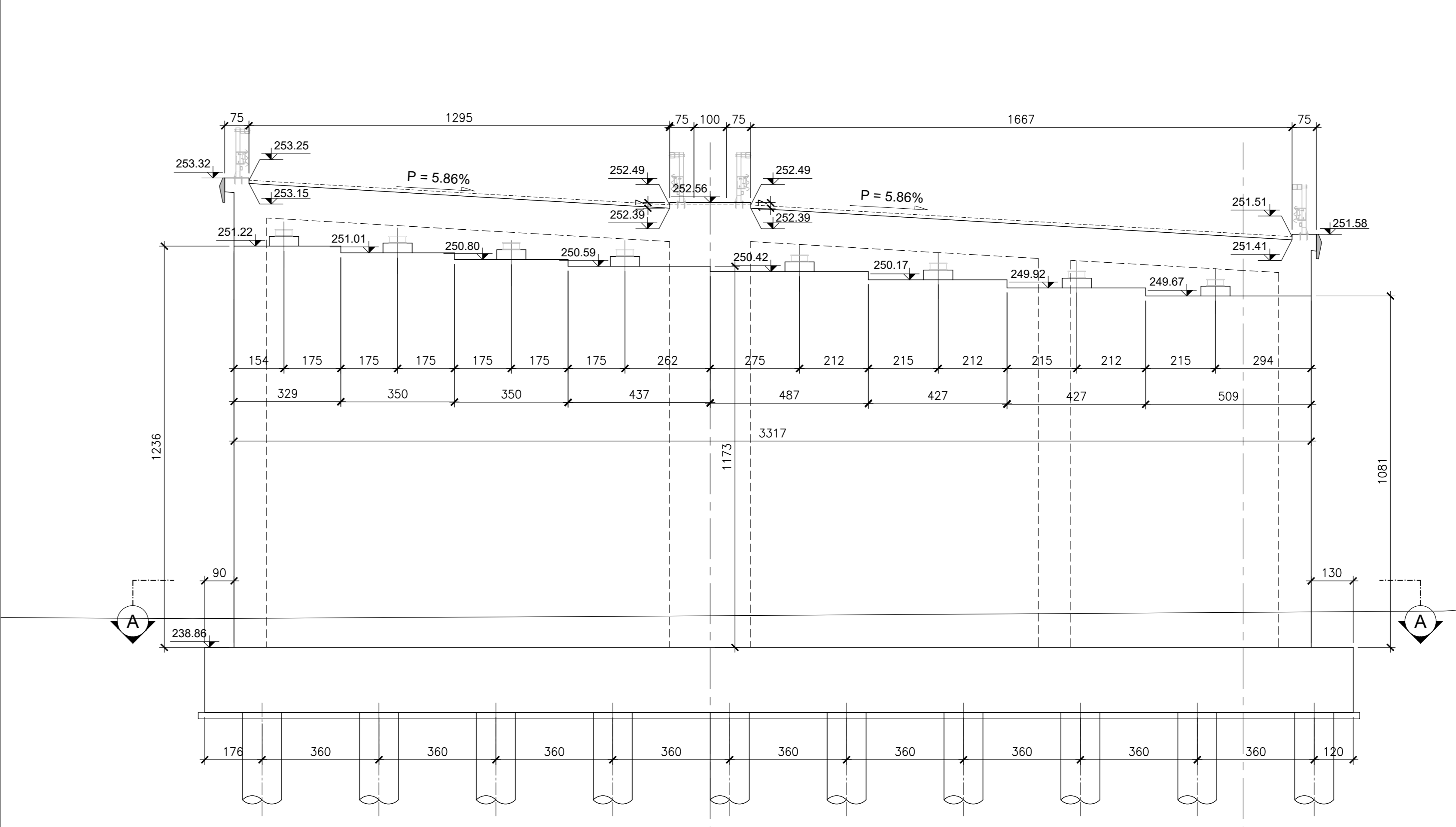
PROSPETTO FRONTALE C-C SCALA 1:100
