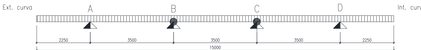
Figura 1 – Schema di riferimento per il calcolo dell'azioni g_1 sulle travi principali
