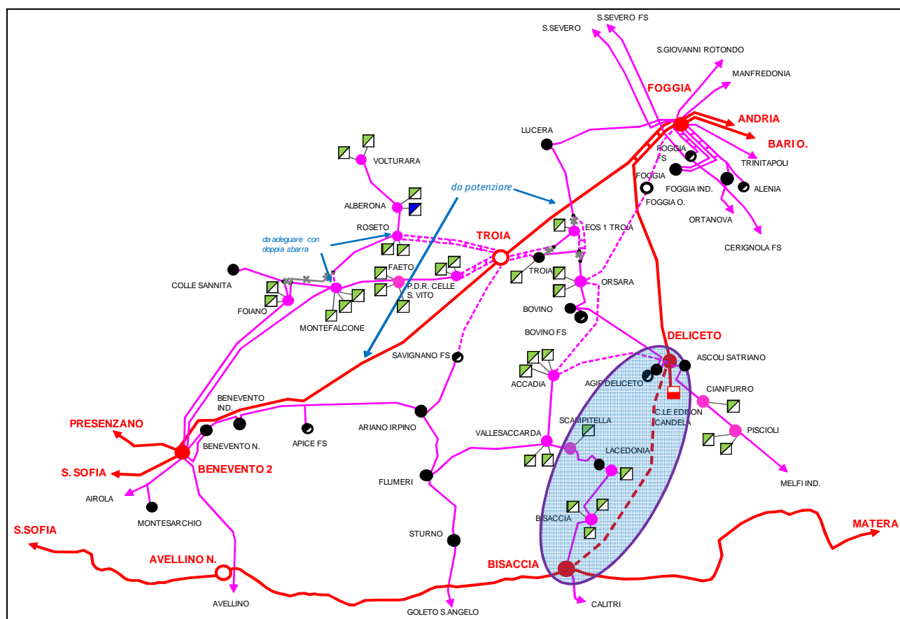
Figura 1 – Elettrodotto 380 kV “Deliceto - Bisaccia”
