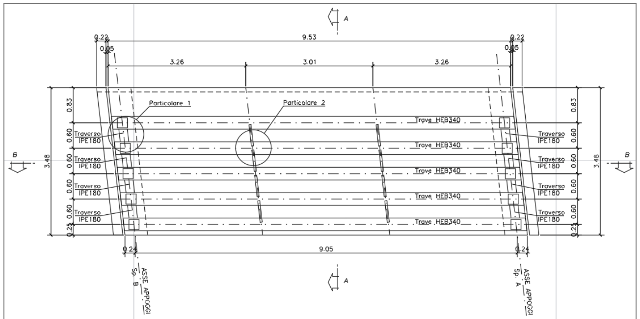
Figura 2-4 Carpenteria
