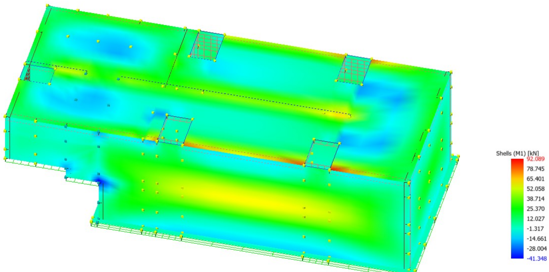
Diagramma del momento flettente M1 allo SLU
