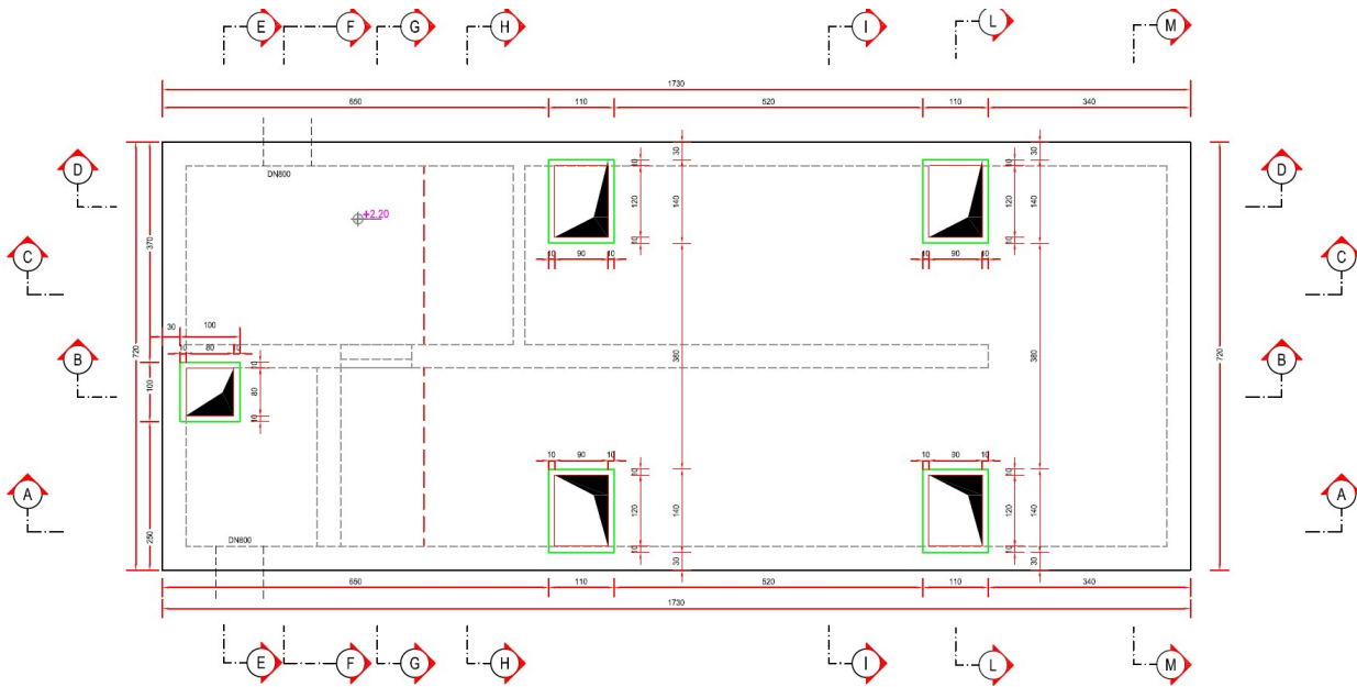
I.1 PIANA DELLA COPERTURA
