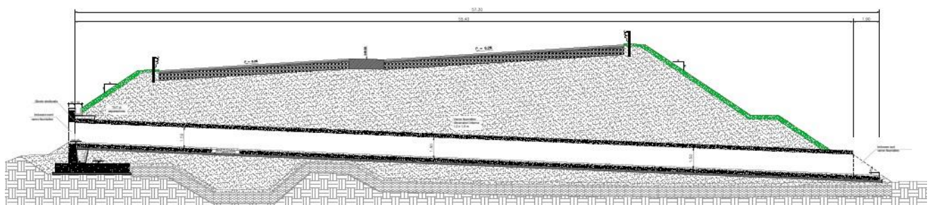
I.2 Sezione longitudinale - Sottopasso faunistico
