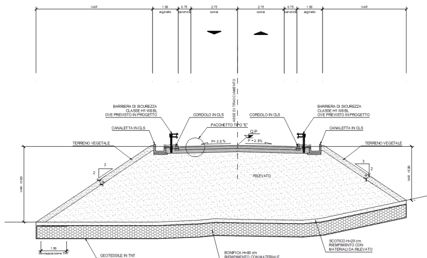
Sezione tipologica Via Cadorna
