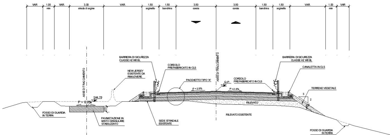
Sezione tipologia rampa di svincolo bidirezionale
