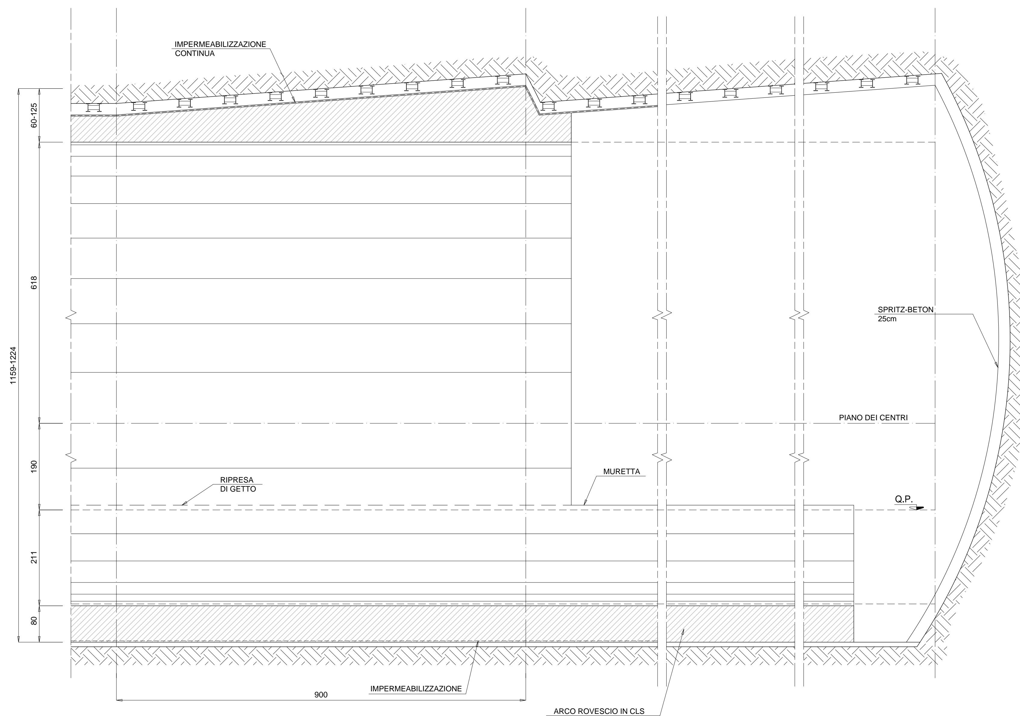
SEZIONE LONGITUDINALE TIPO RACCORDO B2 - C2VP-1 scala 1:50
