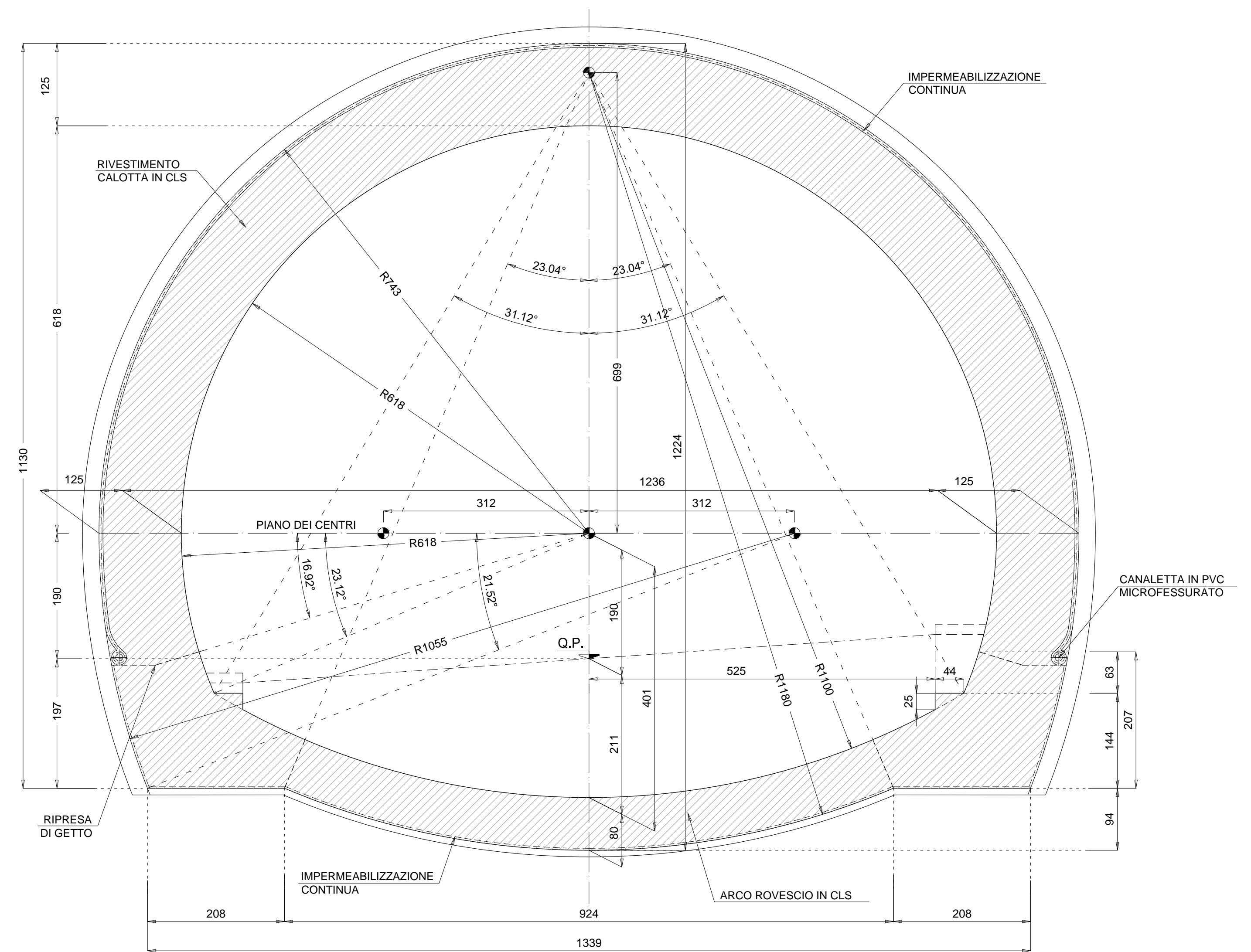
SEZIONE TRASVERSALE (MAX) TIPO RACCORDO B2 - C2VP-1 scala 1:50
