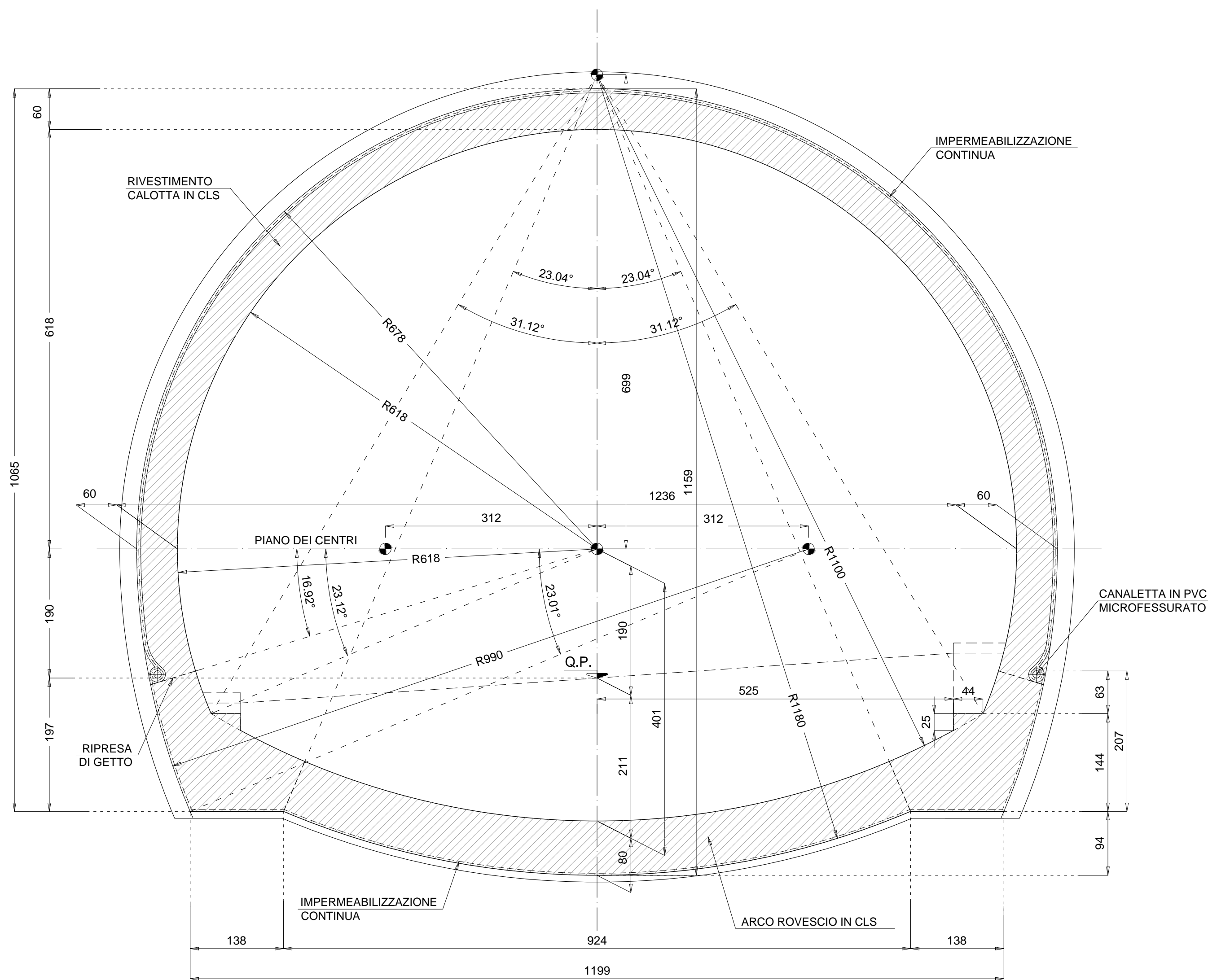
SEZIONE TRASVERSALE (MIN) TIPO RACCORDO B2 - C2VP-1 scala 1:50
