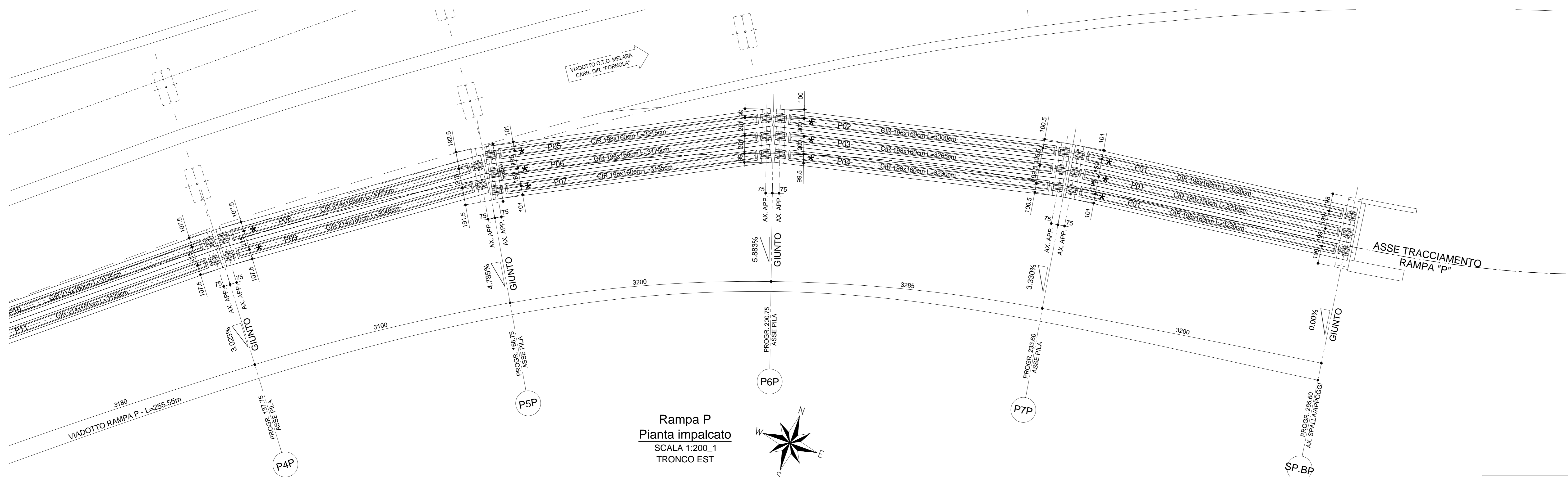
Rampa P Pianta impalcato SCALA 1:200_1 TRONCO OVEST
