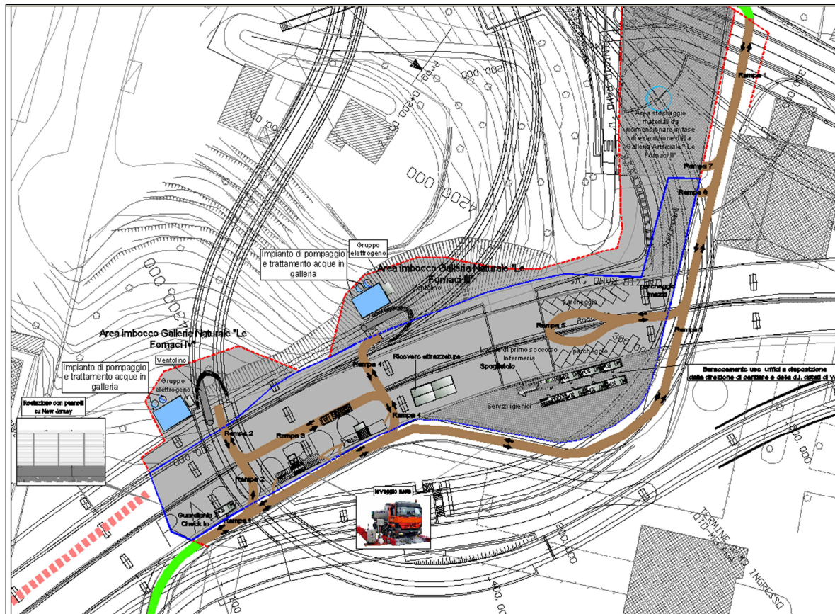
Viabilità interna al cantiere Melara
