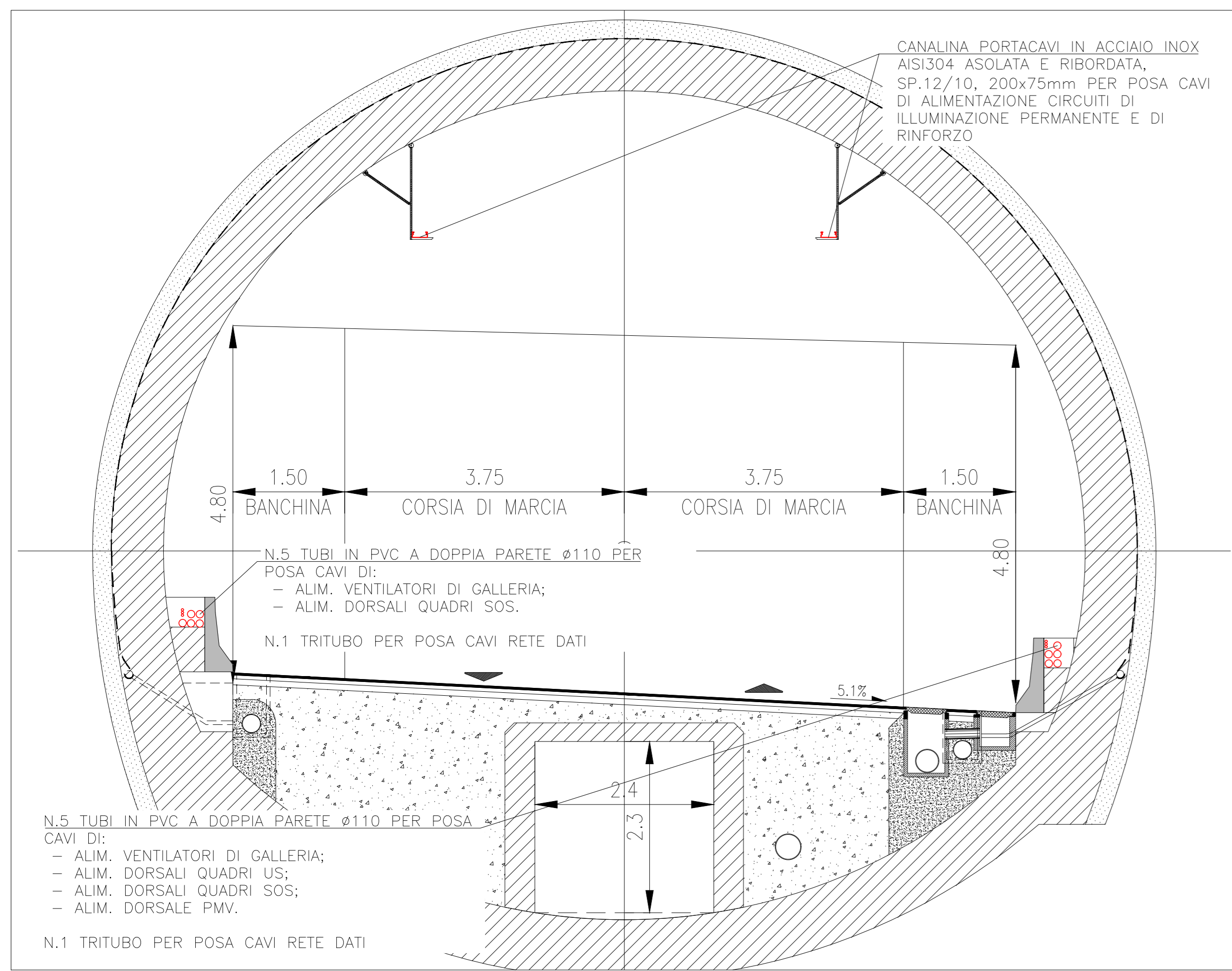
SEZIONE TIPICA VIE CAVI IN GALLERIA – IN DELLA SEZIONE W8 (1:50)
