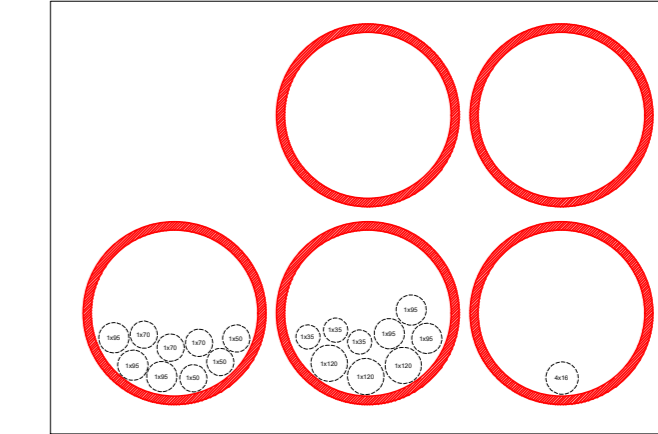
DETTAGLIO RIEMPIMENTO BANCO TUBI LATO SX
