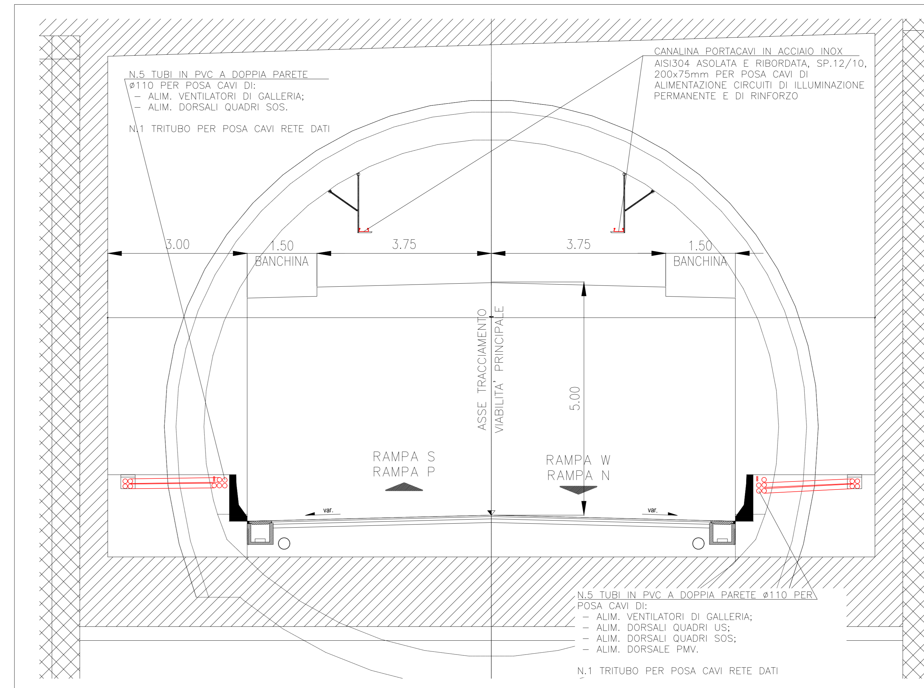
SEZIONE TIPICA VIE CAVI IN GALLERIA – IN DELLA SEZIONE W1 (1:50)
