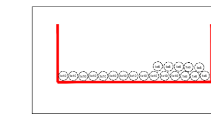
DETTAGLIO RIEMPIMENTO PASSERELLE IN VOLTA LATI DX/SX
