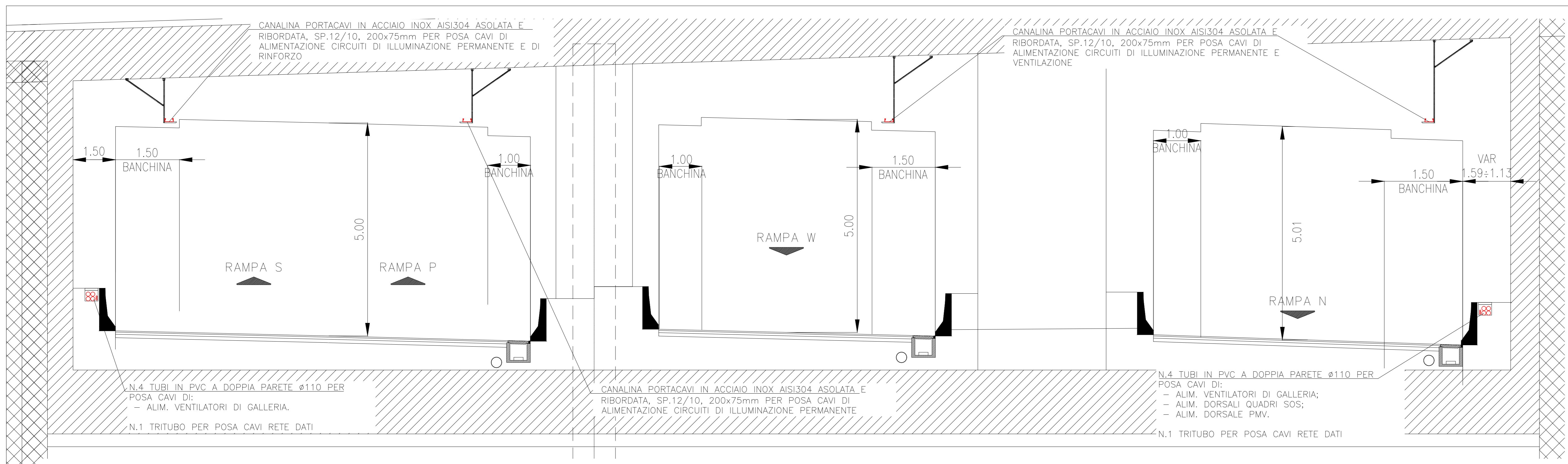
SEZIONE TIPICA VIE CAVI IN GALLERIA – IN DELLA SEZIONE W10 (1:50)
