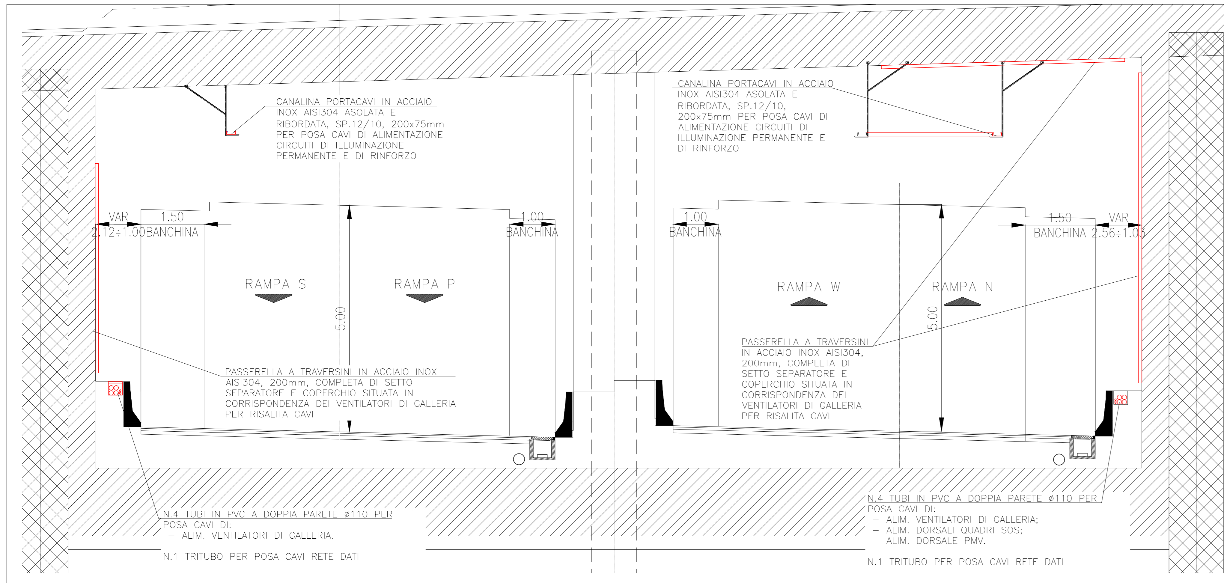
SEZIONE TIPICA VIE CAVI IN GALLERIA – IN DELLA SEZIONE W8 (1:50)
