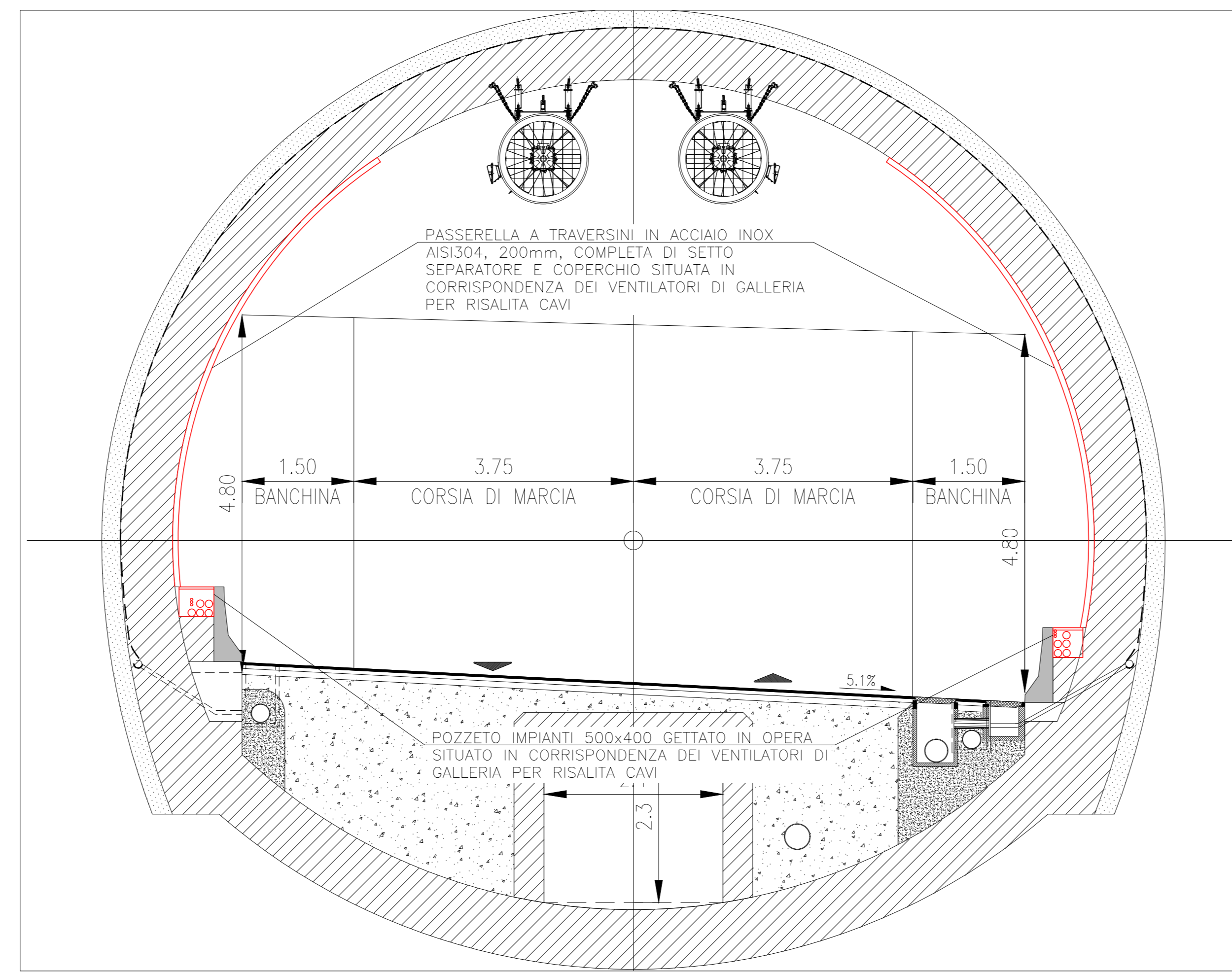
SEZIONE TIPICA VIE CAVI IN GALLERIA – IN DELLA SEZIONE W1 (1:50)
