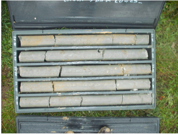
SONDAGGIO S1 CASSETTA N. 5 da mt. 20.00 a mt. 25.00
