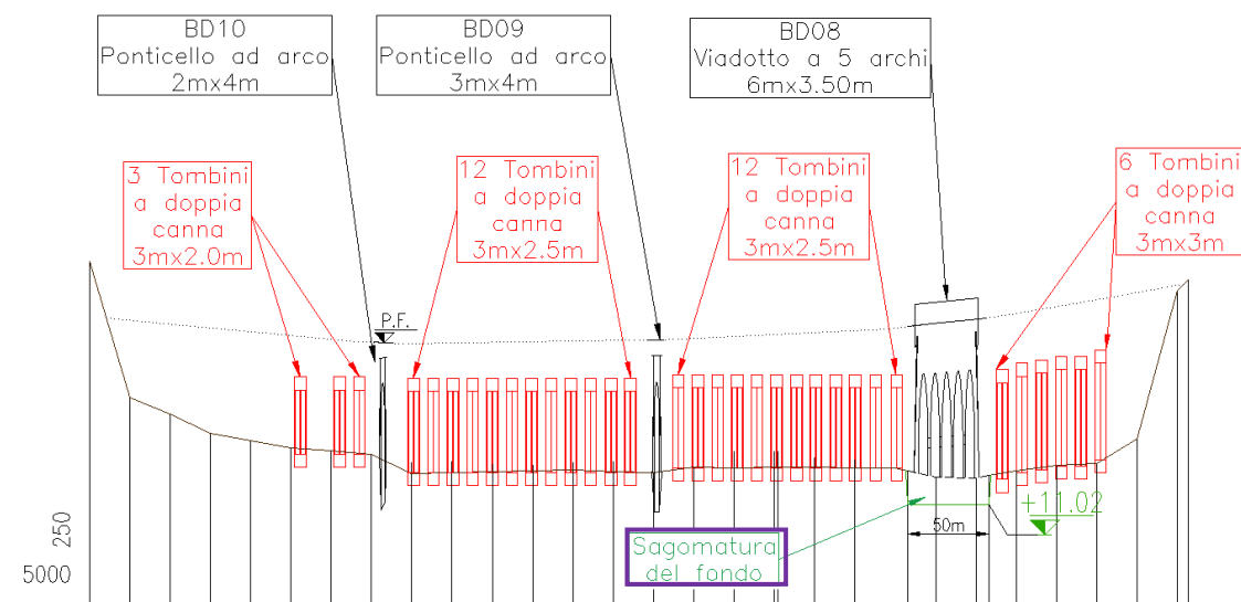
Figura 28: ipotesi progettuale: Sezione trasversale ubicata a monte della linea Barletta-Canosa
