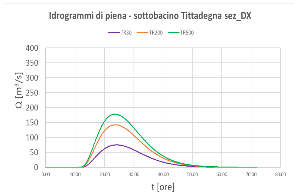
Figura 10: Idrogrammi di Piena – SEZDX
