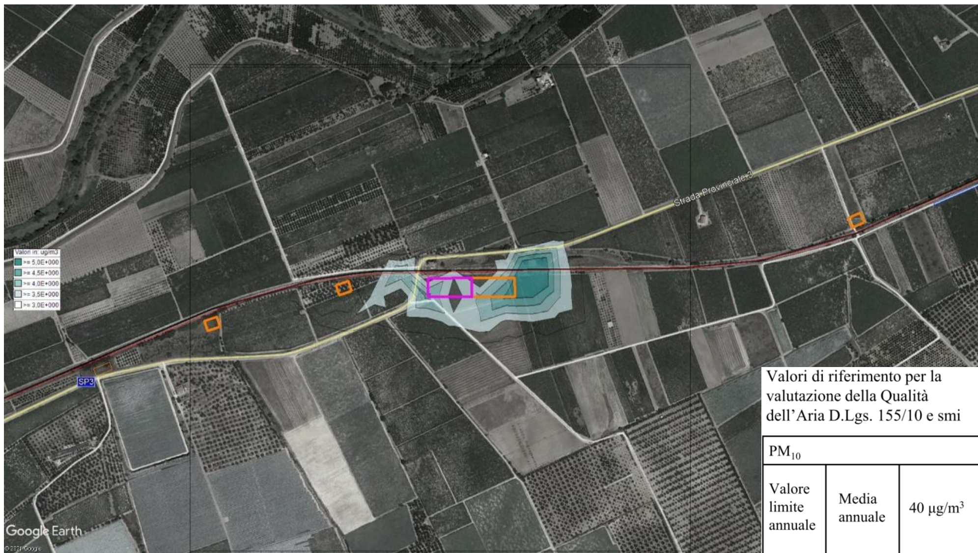
Concentrazioni di PM 10 dovute alle emissioni dei mezzi d'opera dell'area 1B
