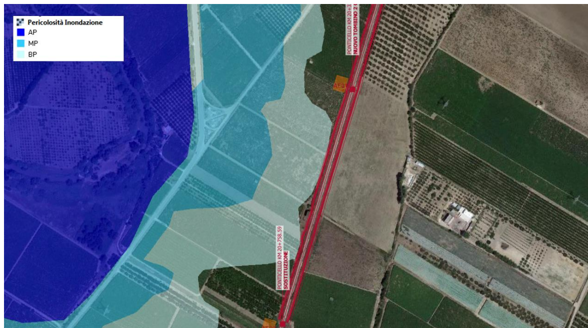
Figura 4-17: Pericolosità idraulica. - AdB della Regione Puglia, prog km 20+420÷ 20+650
