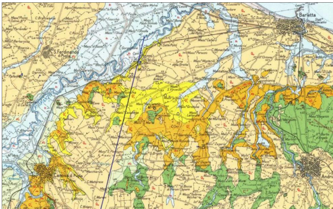
Figura 4-12 – Stralcio ingrandito della Carta Geologica d'Italia - foglio 176 Barletta - scala 1: 100.000.
