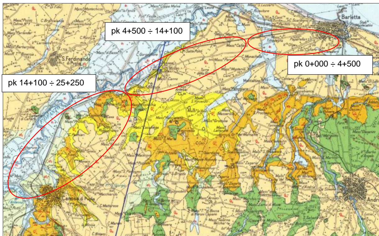
Figura 4-13 – Stralcio, non in scala, della Carta Geologica d'Italia 1:100.000
