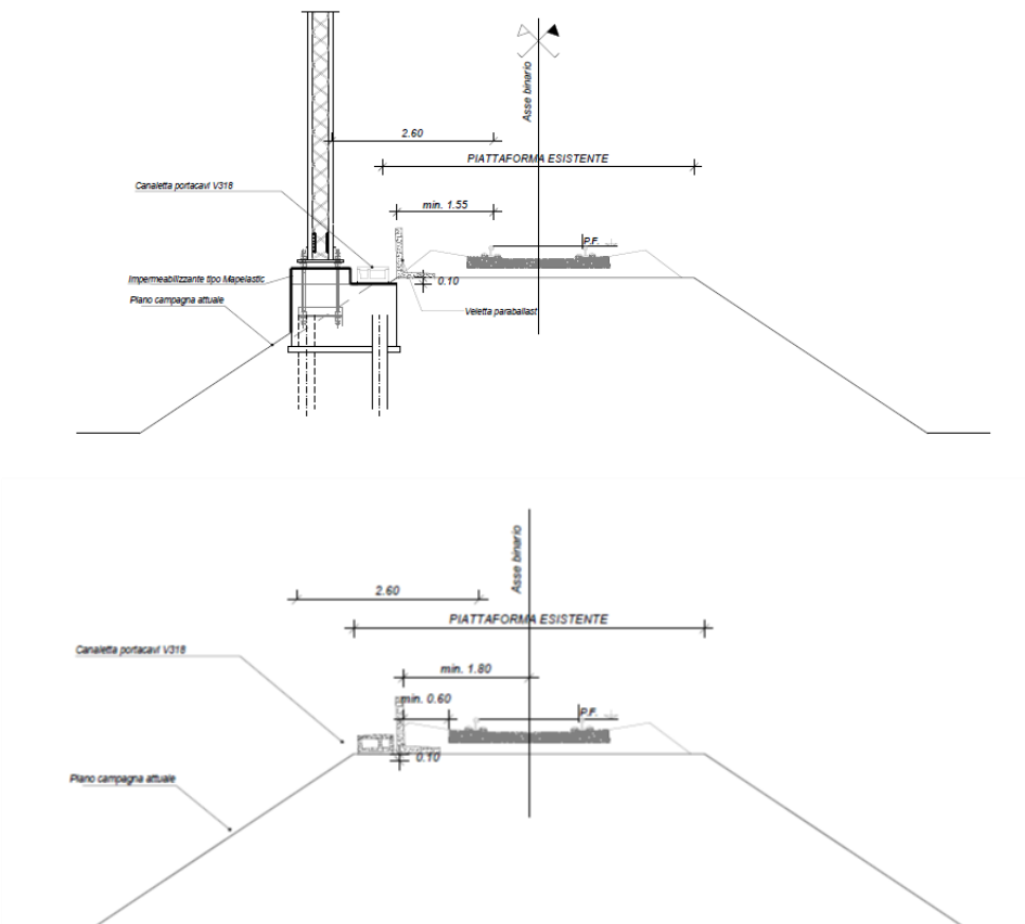
Figura 4-5 – sezioni tipologiche in corrispondenza della zona del Torrente Tittadegna
