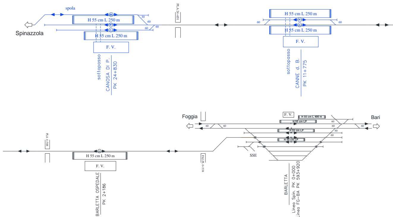
Figura 4-2 – Layout funzionale di progetto (in blu le nuove realizzazioni a Canosa e Canne d.B.)
