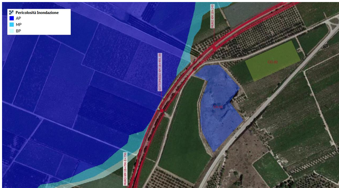
Figura 4-15: Pericolosità idraulica. - AdB della Regione Puglia, prog km 18+330 ÷ 18+640
