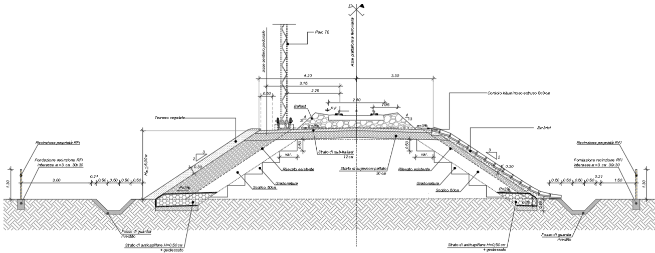
Figura 4-4 – sezione tipologica in rilevato
