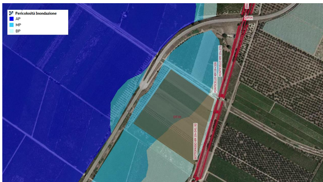
Figura 4-16: Pericolosità idraulica. - AdB della Regione Puglia, prog km 19+150 ÷ 19+550
