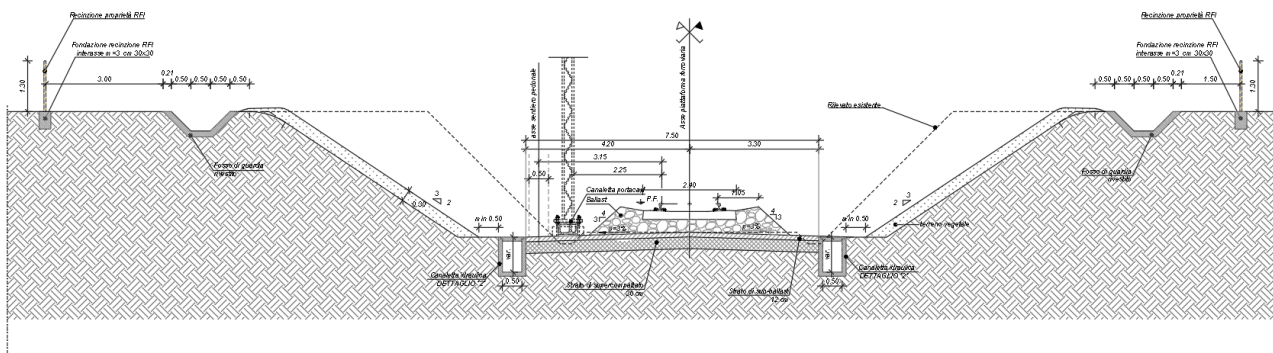
Figura 4-3 – sezione tipologica in trincea
