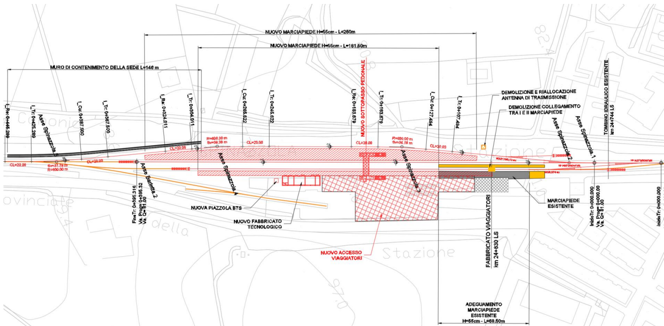
Figura 4-6 – Planimetria di Progetto - Modifica al PRG di Canosa di Puglia
