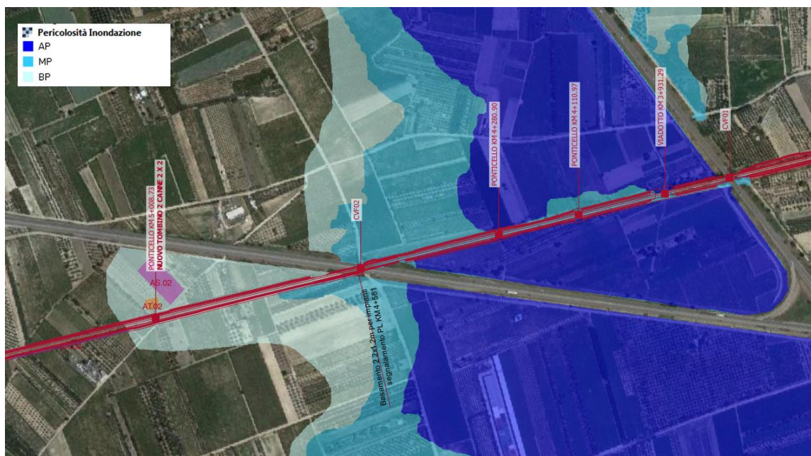
Figura 4-14: Pericolosità idraulica. - AdB della Regione Puglia, prog km 3+800 ÷ 5+100
