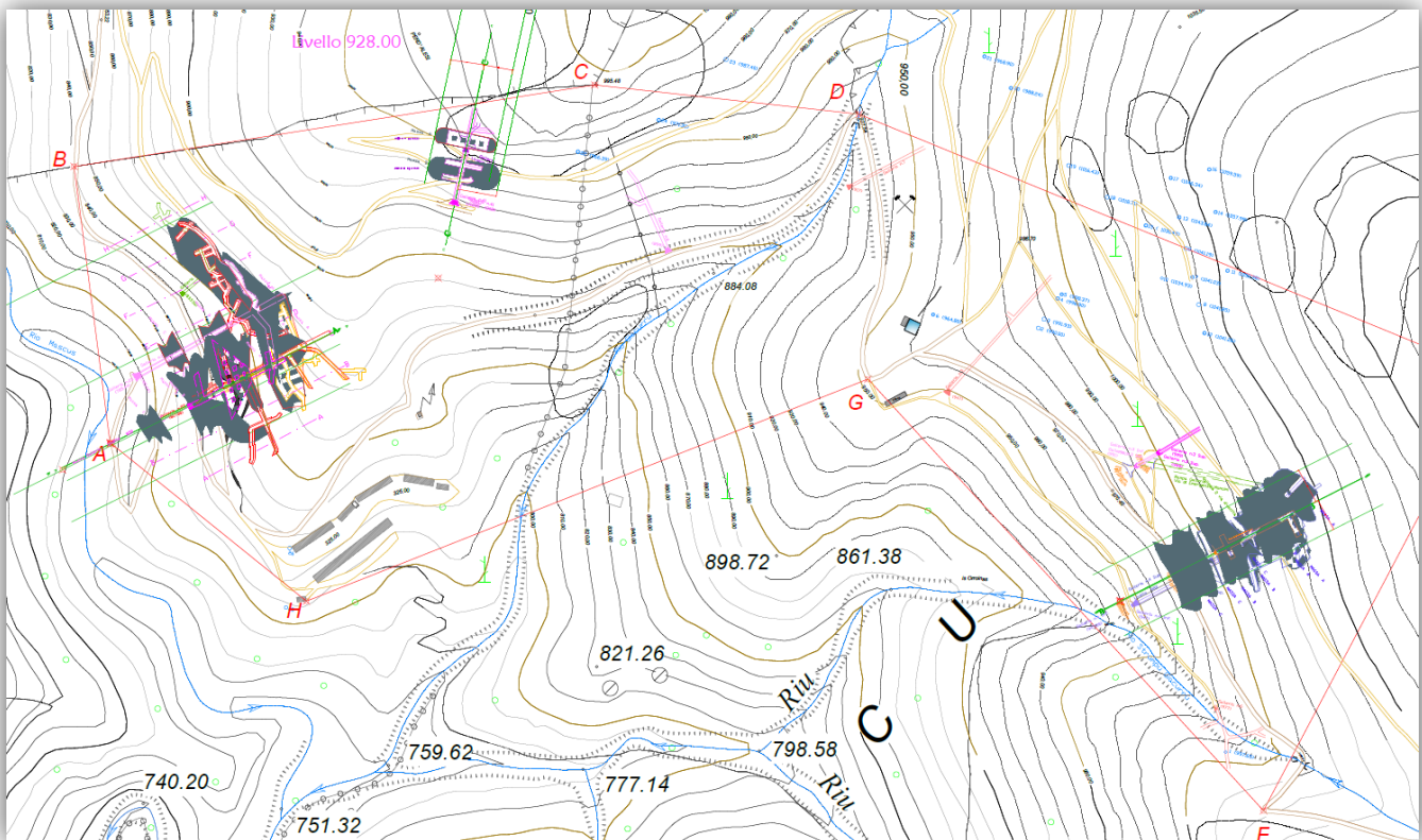
Tav. 4.0- Planimetria e Sezioni VALUTAZIONE GIACIMENTO
