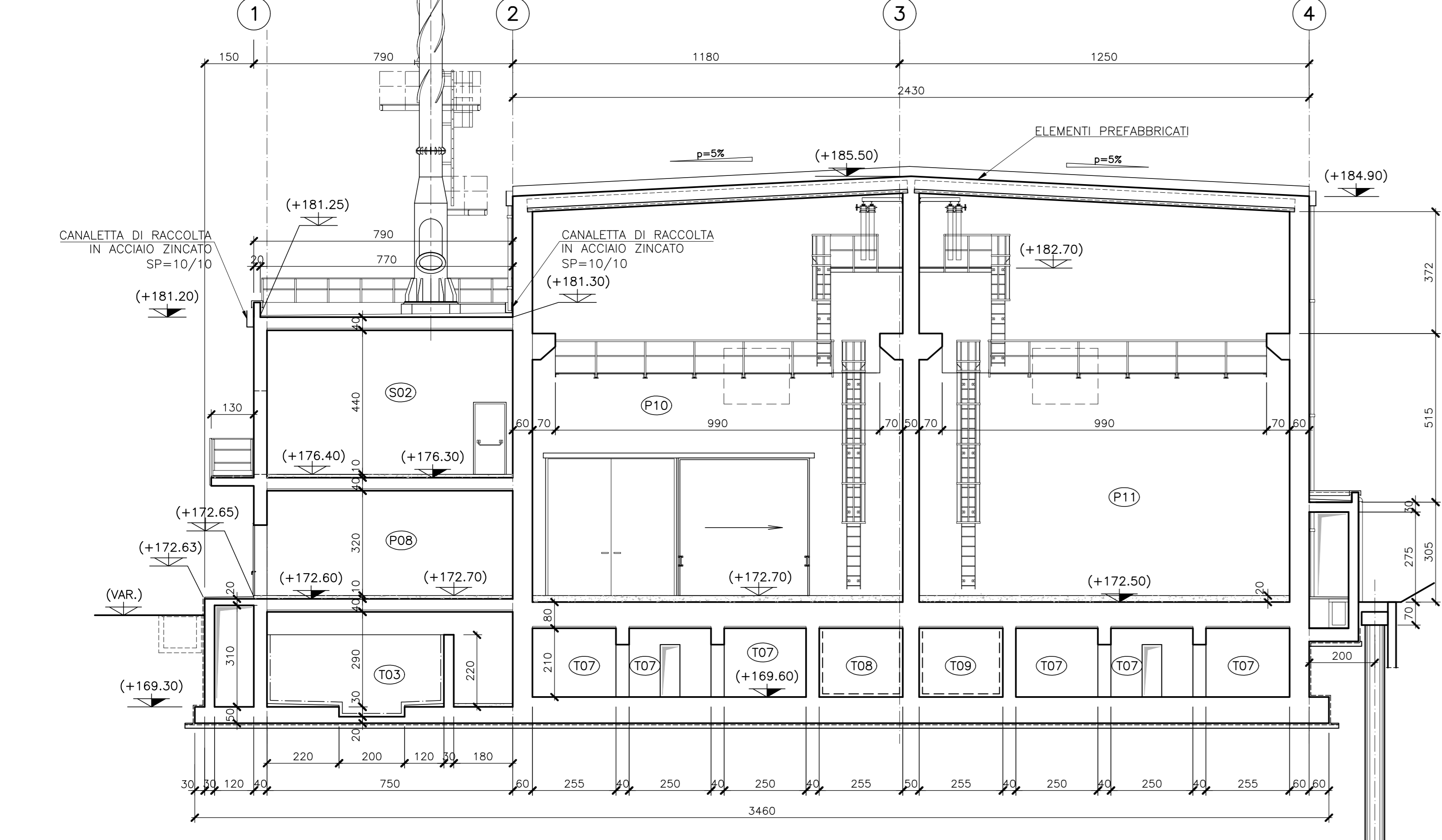
SEZIONE C-C SCALA 1:100
