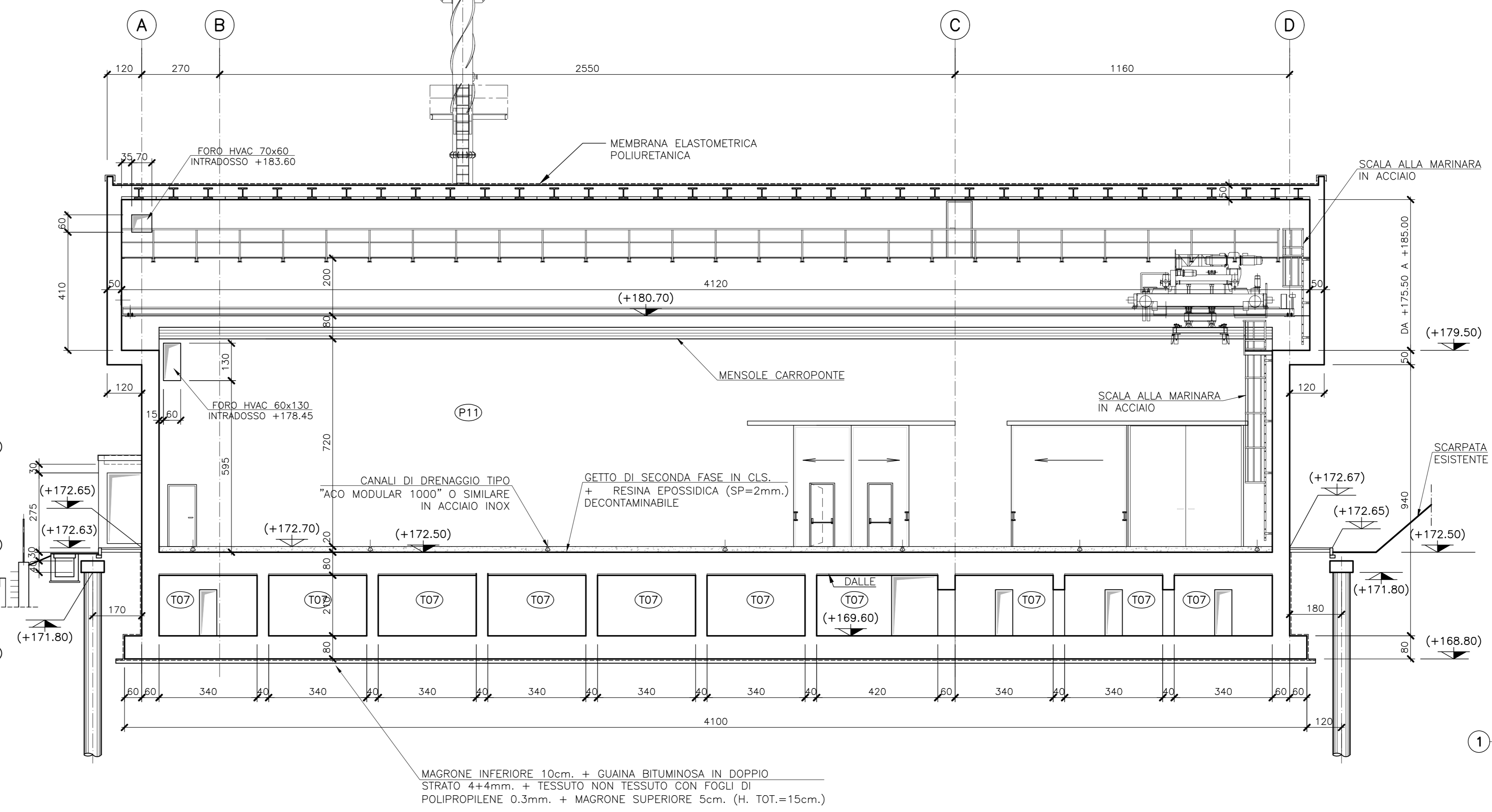
SEZIONE B-B SCALA 1:100
