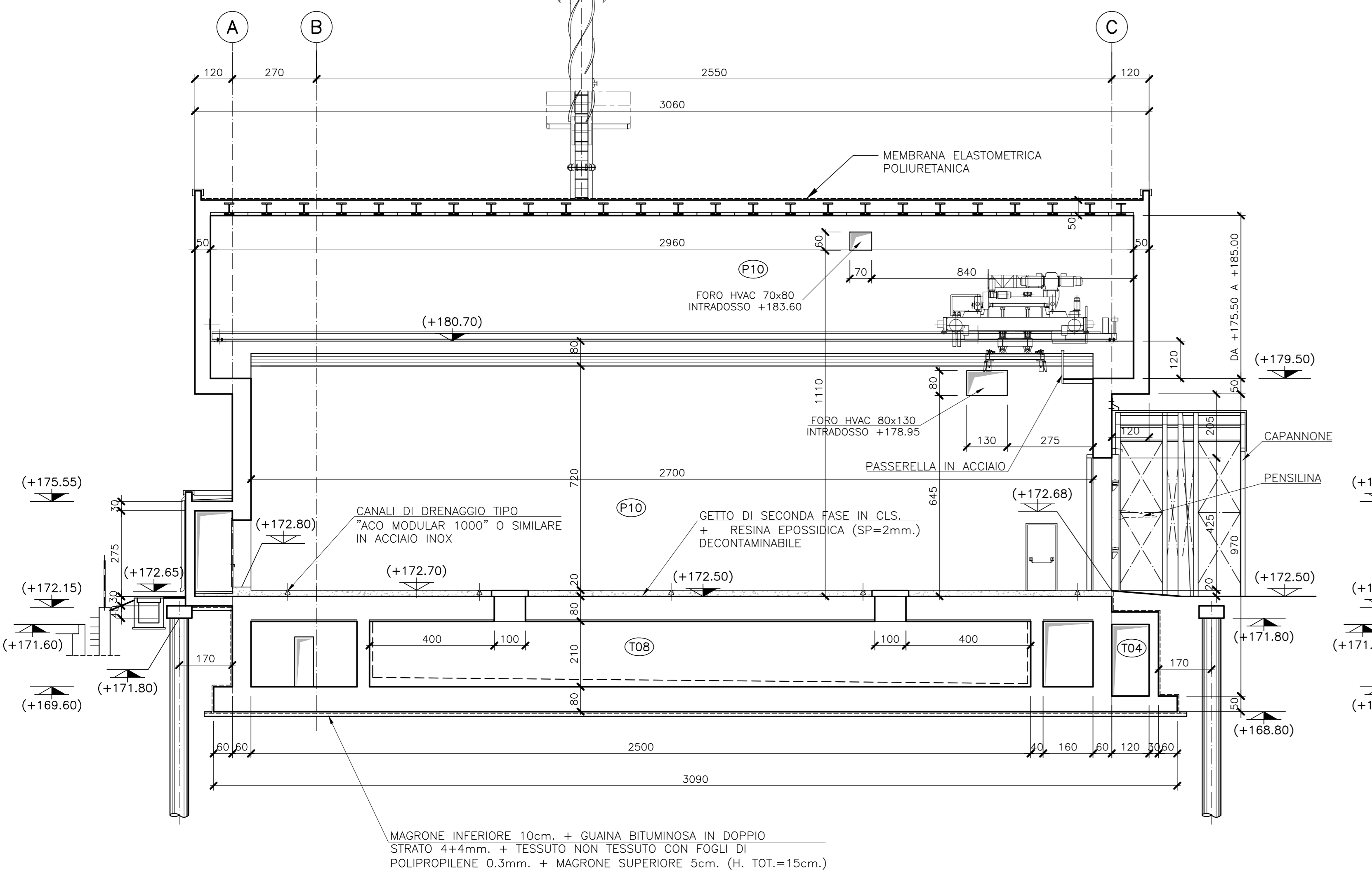
SEZIONE A-A SCALA 1:100
