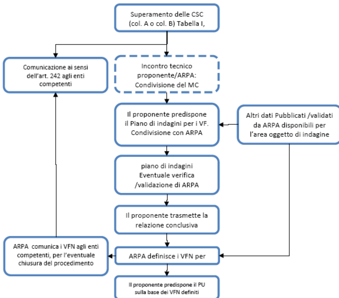
Figura 1. Schema logico per la determinazione dei valori di fondo
