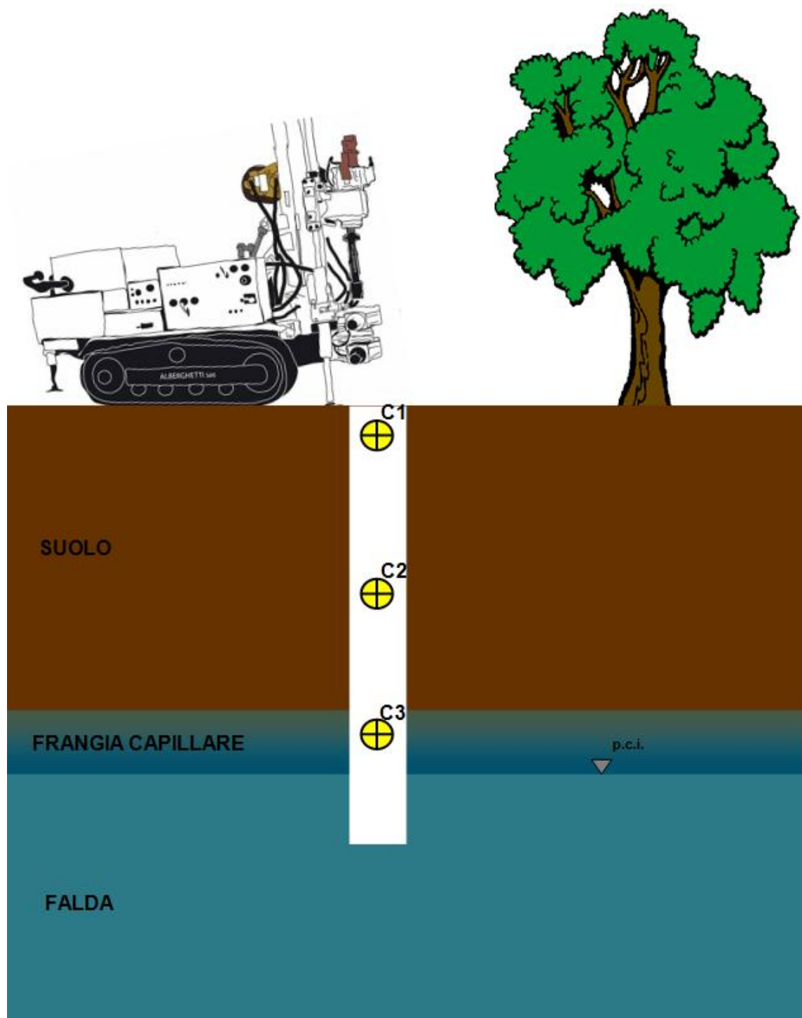
Figura 11. Schema di campionamento in presenza di falda
