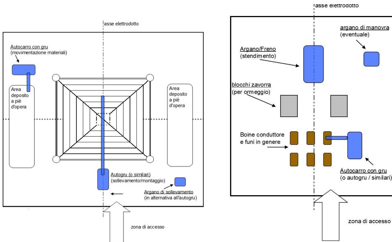
3 - Planimetria dell'Area Sostegno (montaggio sostegno) - Planimetria dell'Area di linea - Tipologico
