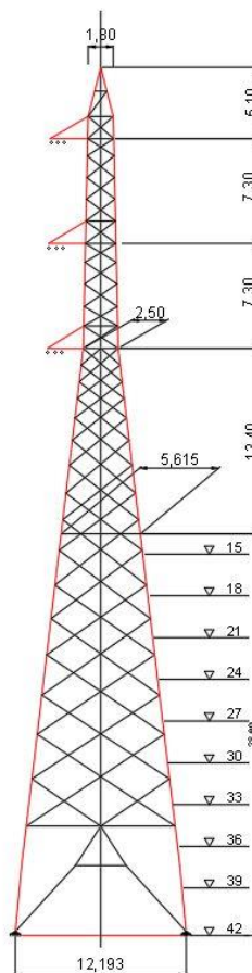
Schema sostegno a semplice terna tipo "EP"
