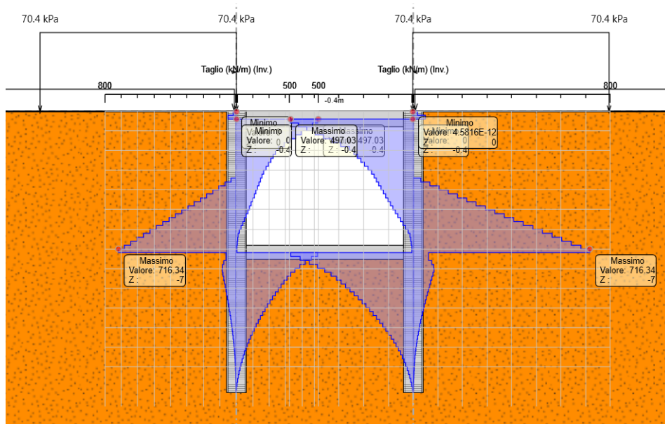
Figura 12 Involuppo taglio
