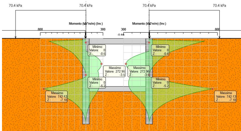
Figura 19 Involuppo momento flettente
