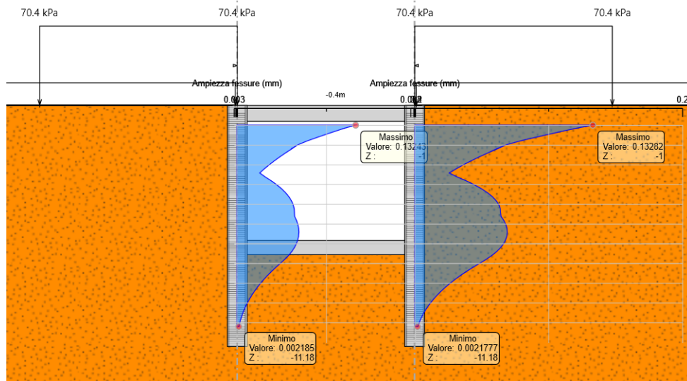
Figura 24 Verifica a fessurazione SLE
