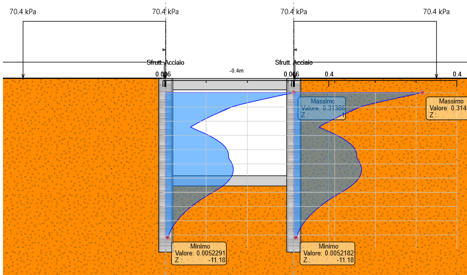
Figura 23 Verifica tensioni di esercizio nell'acciaio
