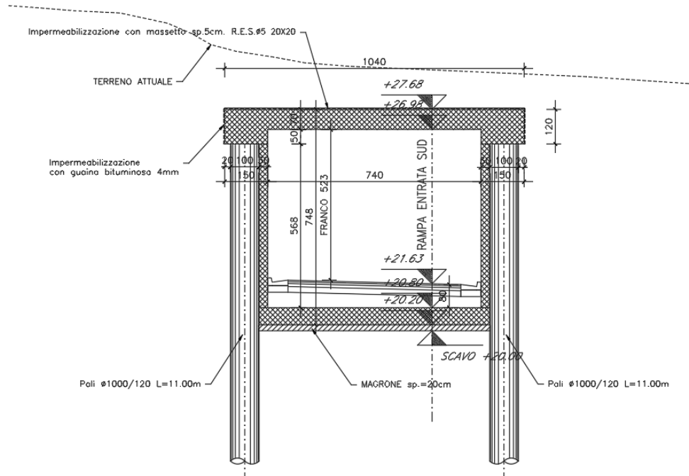
Figura 5 – Sezione Galleria artificiale non carrabile
