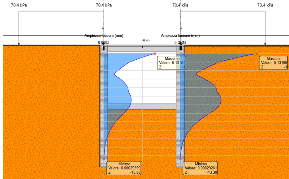
Figura 16 Verifica a fessurazione SLE
