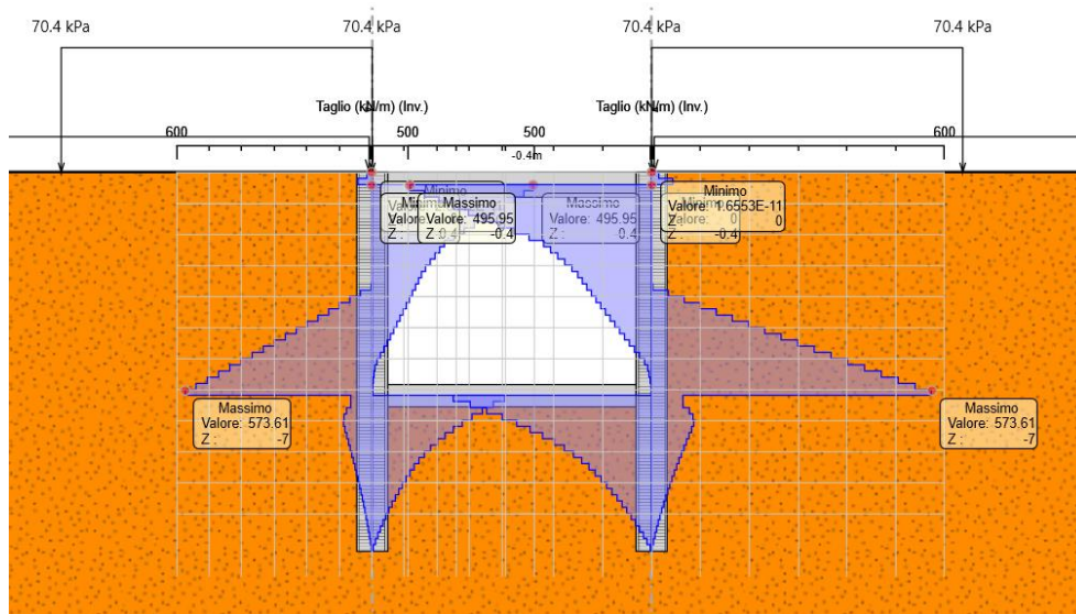
Figura 20 Inviluppo taglio
