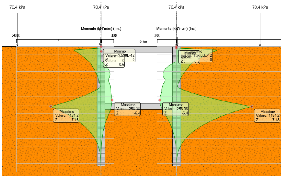
Figura 11 Inviluppo momento flettente
