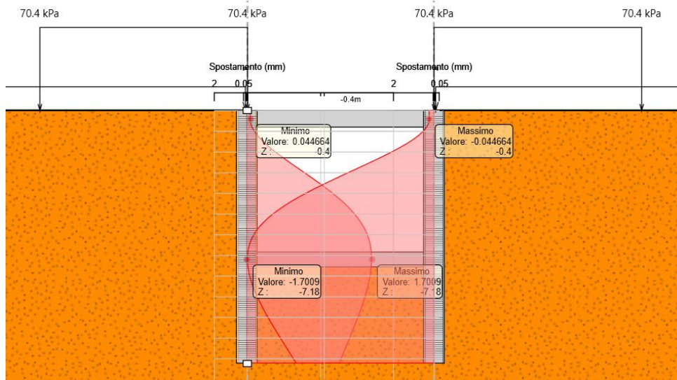
Figura 18 Involuppo spostamenti allo SLE. |u_{max}|=1.70 mm
