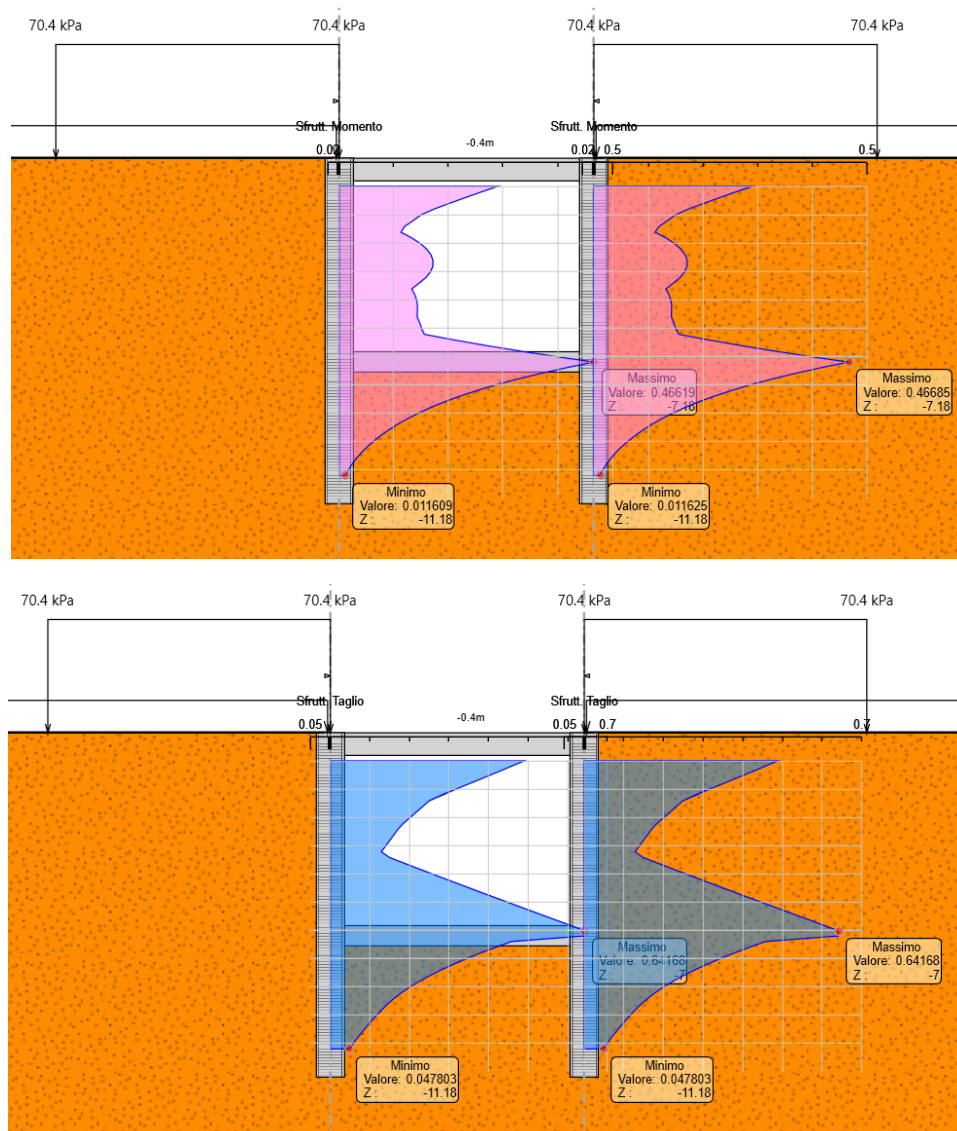
Figura 21 Verifica strutturale palo SLU
