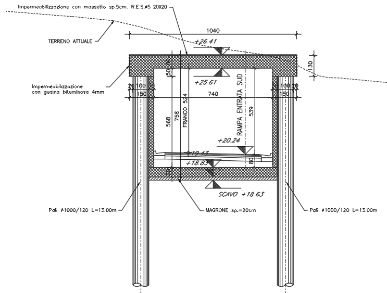
Figura 4 – Sezione Galleria artificiale carrabile
