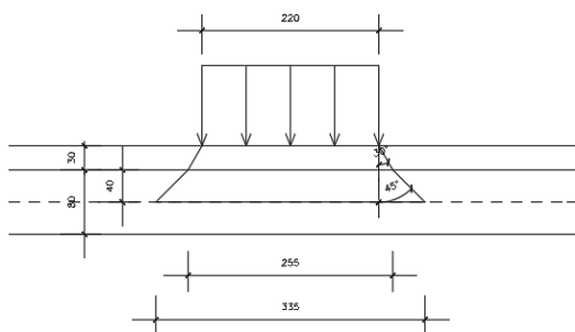
Figura 6 – Schema diffusione carichi stradali (galleria carrabile)
