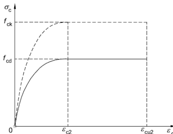
Figura 7 - Legame costitutivo di progetto del calcestruzzo
