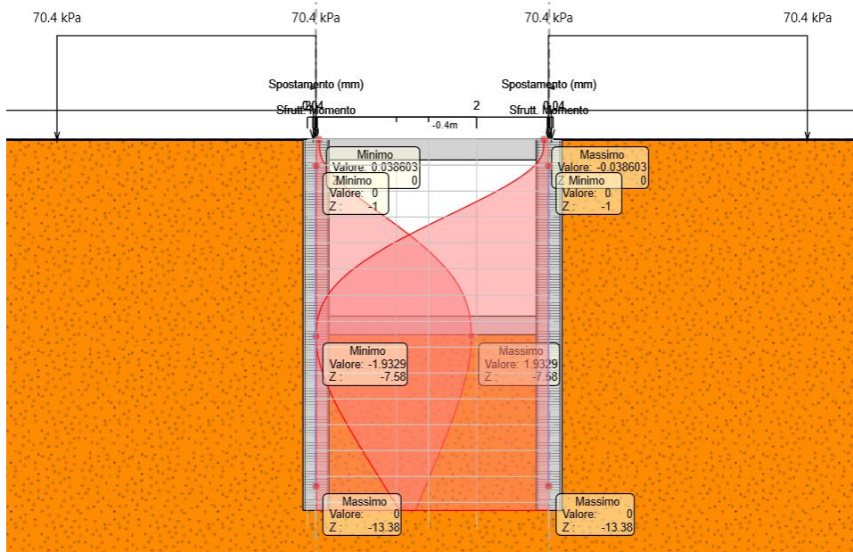
Figura 10 Inviluppo spostamenti allo SLE. |u_{max}|=1.93\text{mm}
