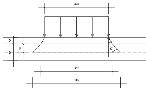
Figura 6 – Schema diffusione carichi stradali (galleria carrabile)
