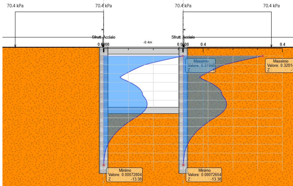
Figura 15 Verifica tensioni di esercizio nell'acciaio
