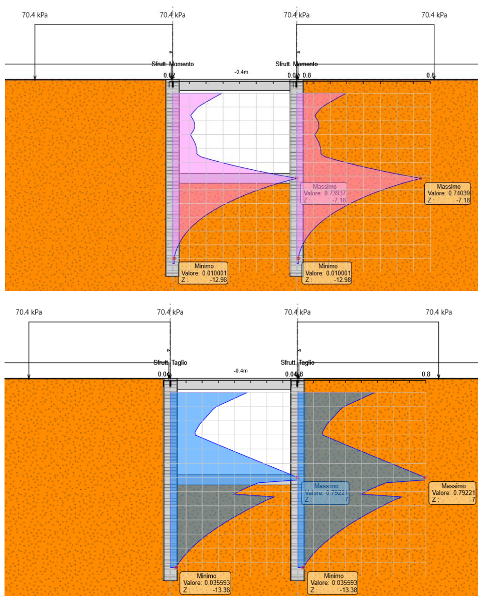
Figura 13 Verifica strutturale palo SLU
