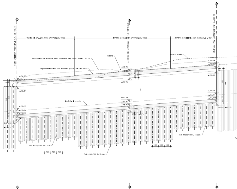
Figura 3 – Pianta e sezione longitudinale
