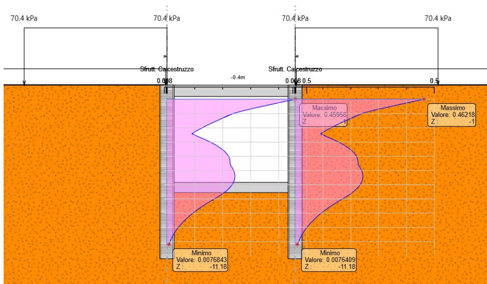
Figura 22 Verifica tensioni di esercizio nel calcestruzzo
