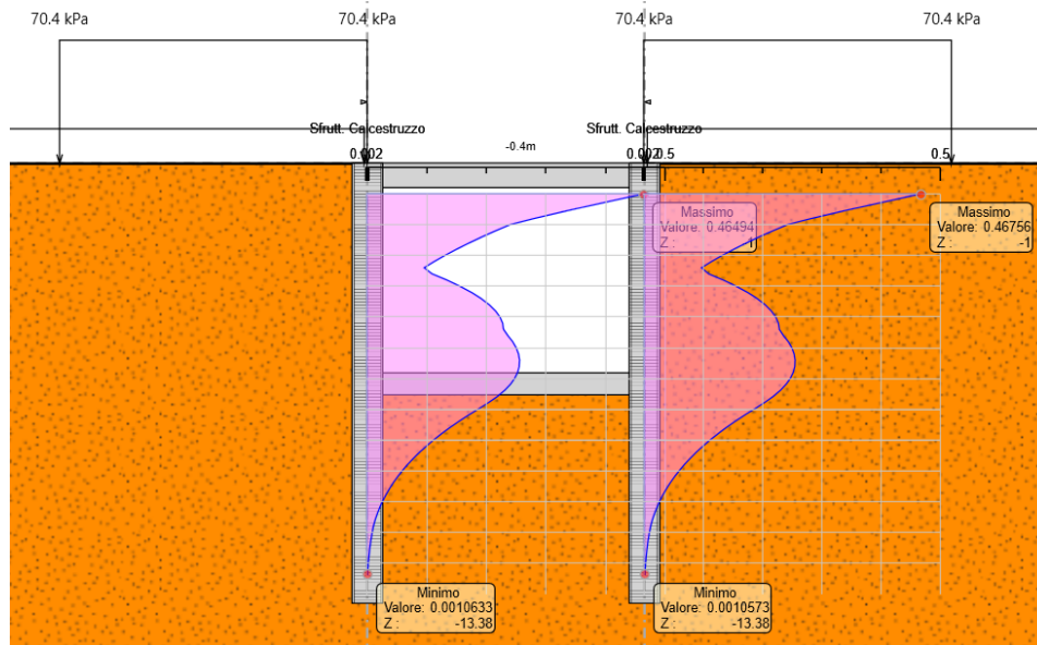
Figura 14 Verifica tensioni di esercizio nel calcestruzzo
