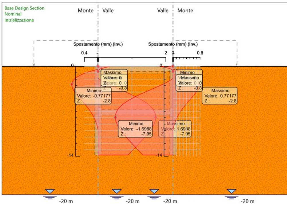
Figura 7 Involuppo spostamenti allo SLE. |umax|=1.79 mm
