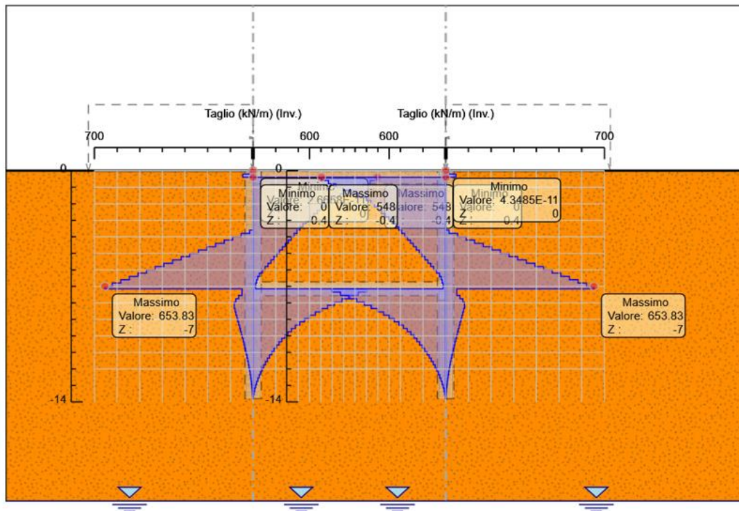
Figura 9 Involuppo taglio SLU-SLV
