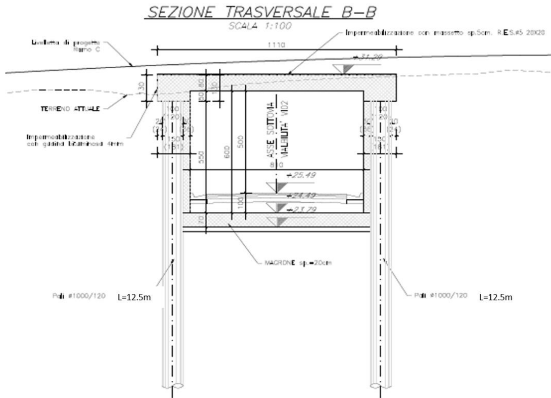
Figura 3 – Sezione Sottovia
