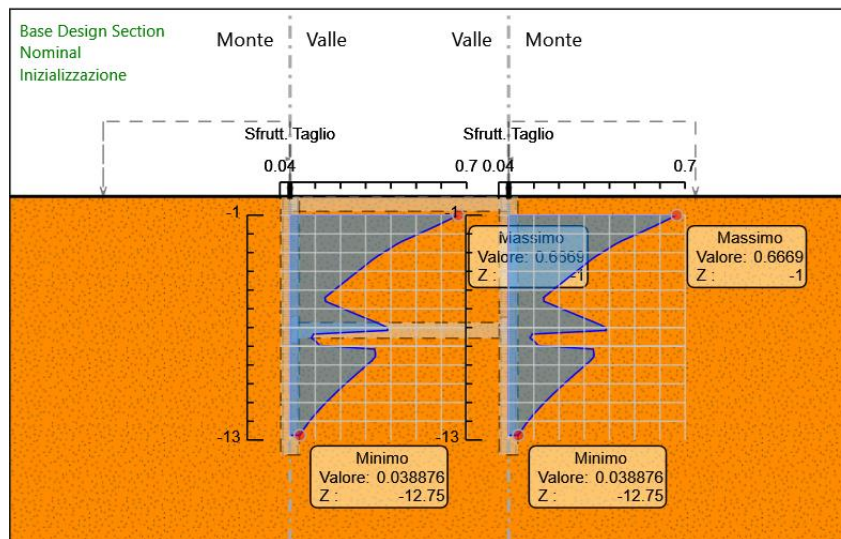
Figura 11 Verifica strutturale palo- tasso di sfruttamento taglio
