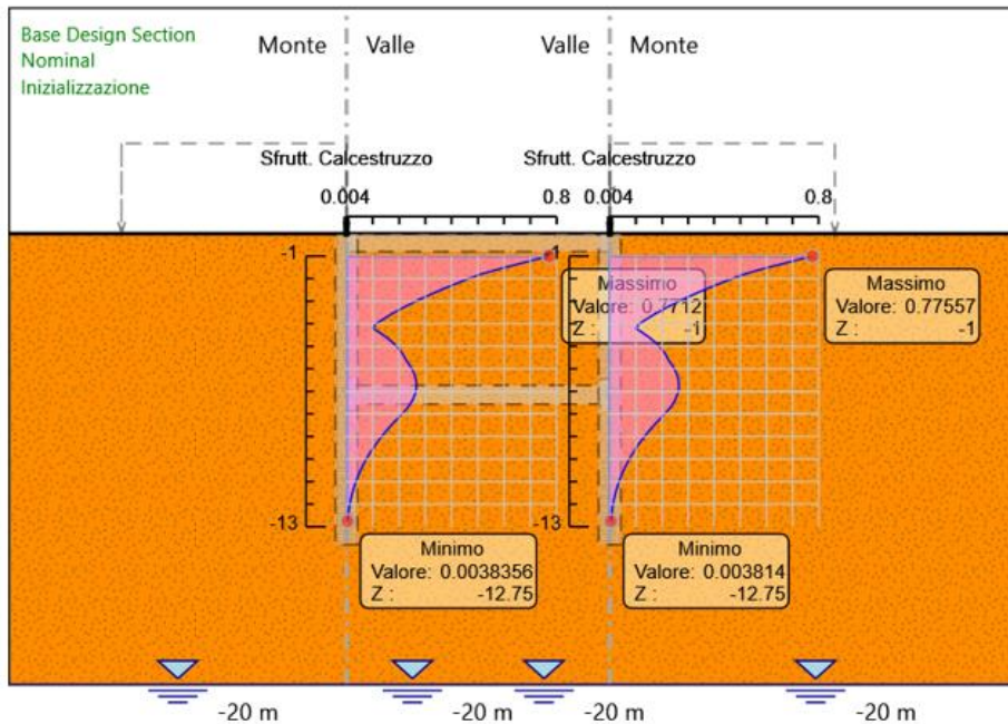
Figura 12: Verifica tensioni di esercizio- tasso di sfruttamento del calcestruzzo
