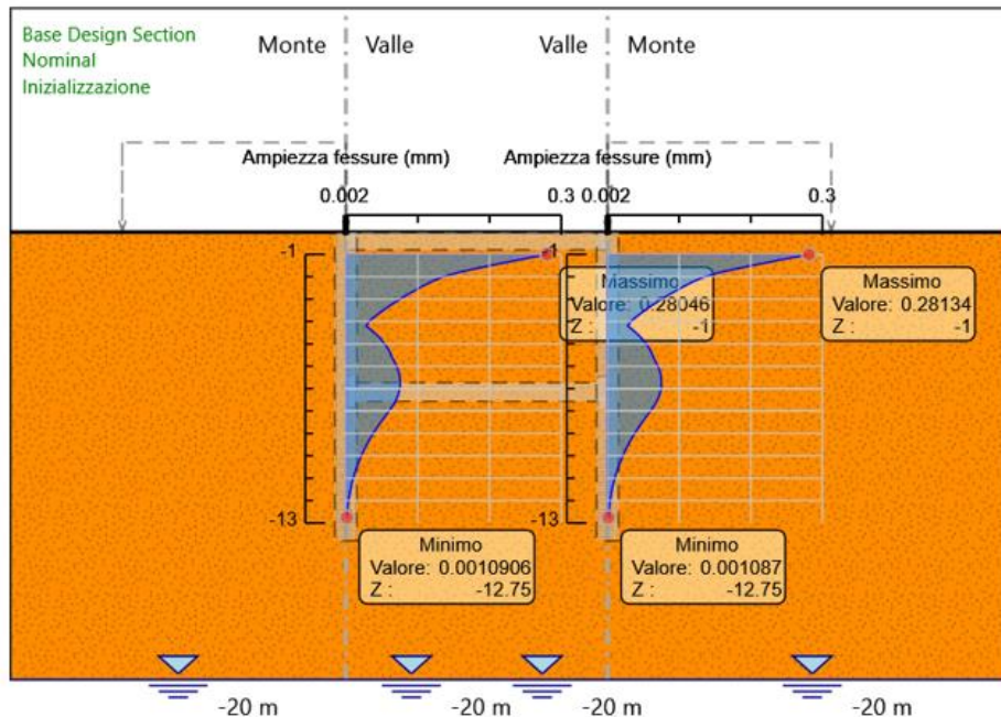
Figura 14: Verifica a fessurazione SLE
