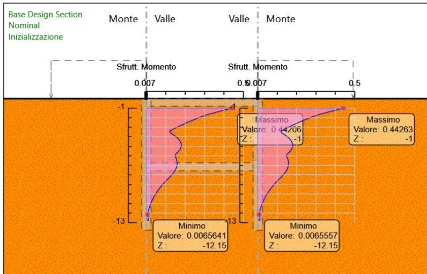
Figura 10: Verifica strutturale palo- tasso di sfruttamento momento
