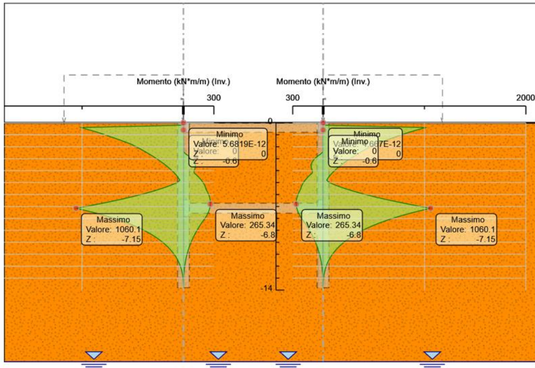
Figura 8 Involuppo momento flettente SLU-SLV
