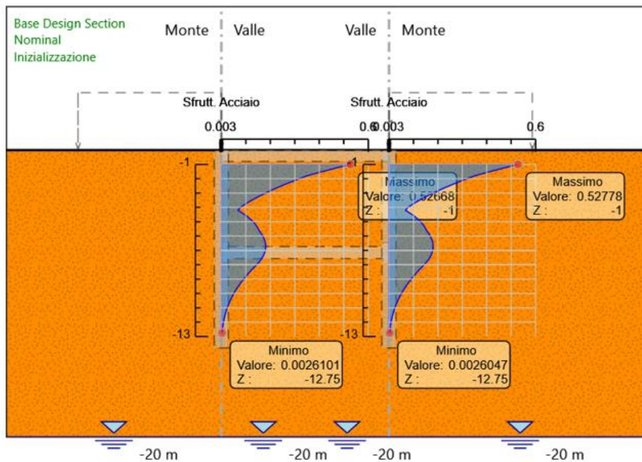
Figura 13: Verifica tensioni di esercizio- tasso di sfruttamento dell'acciaio
