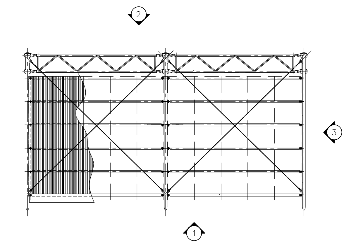
PIANTA CHIAVE
