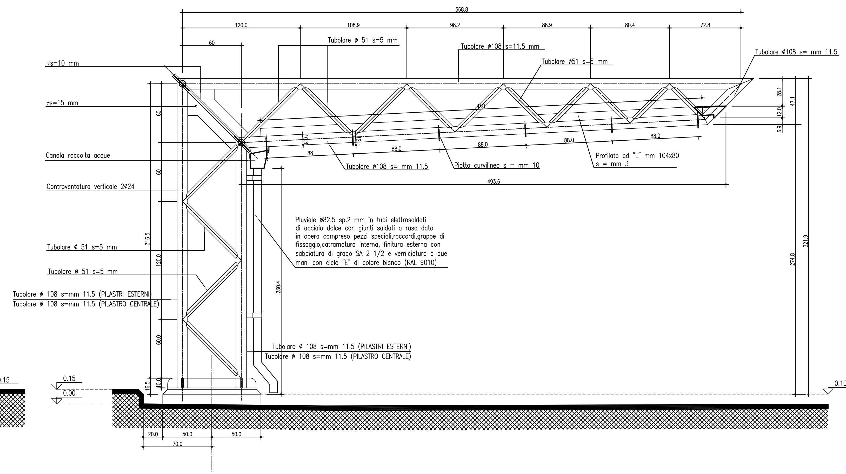
PROSPETTO "3" Rapp. 1:20
