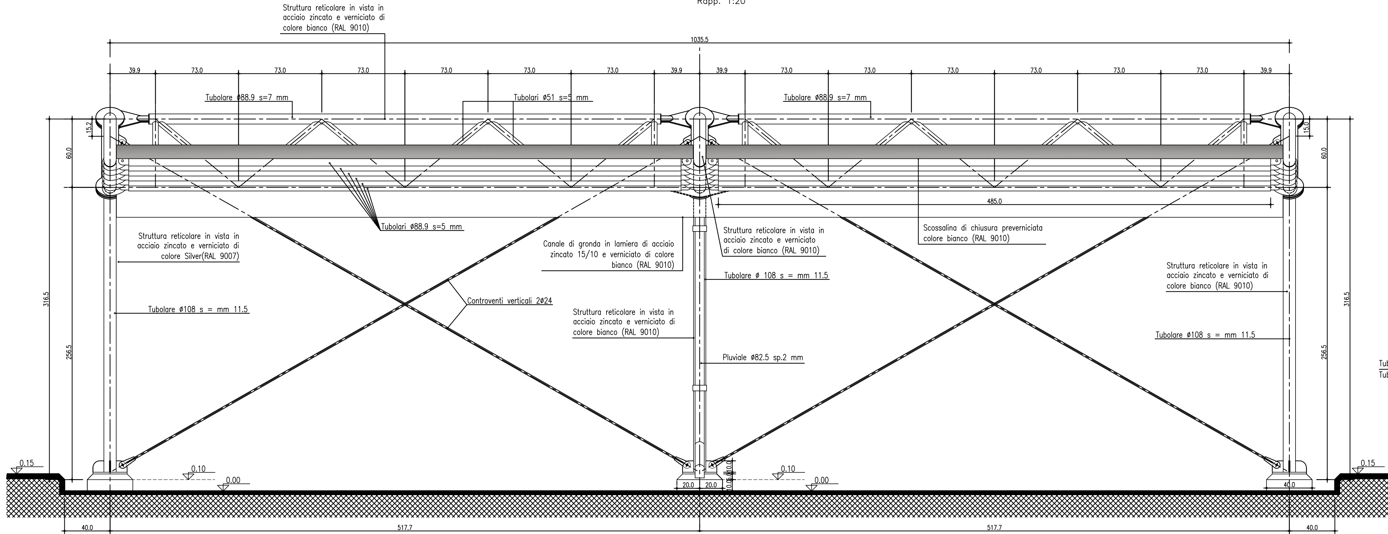
PROSPETTO "1" Rapp. 1:20
