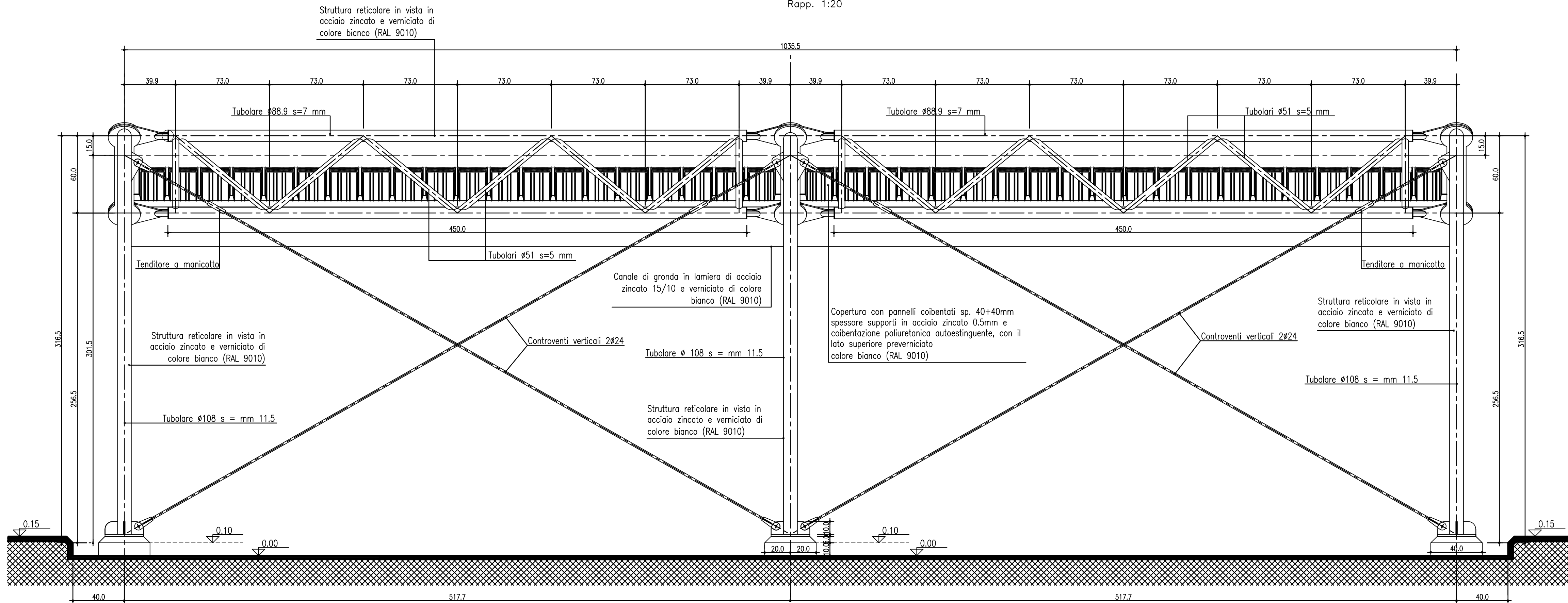
PROSPETTO "2" Rapp. 1:20
