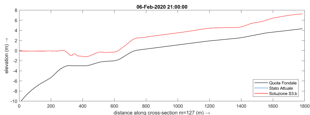
FIGURA 4-13. CONFRONTO DEI LIVELLI IDRICI OTTENUTI NEL TRATTO TERMINALE E ALLA FOCE DEL BISAGNO PER L'EVENTO DI PIENA CON TEMPO DI RITORNO 200 ANNI CON PORTATA AL COLMO Q_{\text{RES}} = 750 \text{ m}^3/\text{s} . STATO ATTUALE (BLU), SOLUZIONE S3.B (ROSSO).
