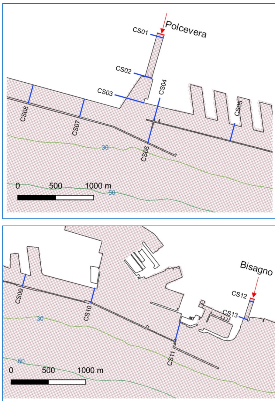
FIGURA 3-9. UBICAZIONE DELLE SEZIONI DI CONTROLLO PER L'ESTRAZIONE DEI RISULTATI IN CORRISPONDENZA DELLA FOCE DEL POLCEVERA E DEL BISAGNO.
