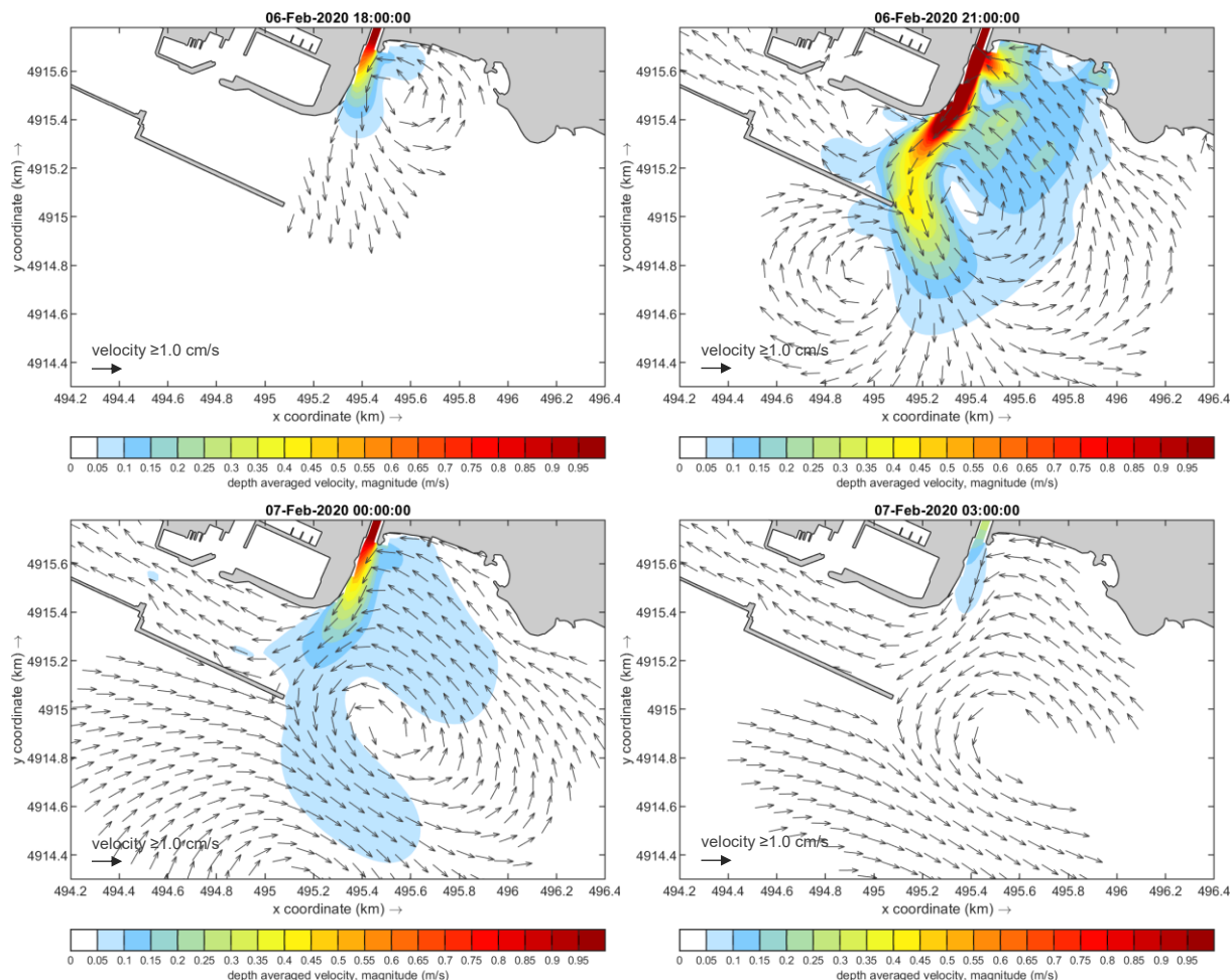
FIGURA 3-18. DETTAGLIO DEI RISULTATI OTTENUTI ALLA FOCE DEL TORRENTE BISAGNO PER L'EVENTO DI PIENA CON TEMPO DI RITORNO 10 ANNI CON PORTATA AL COLMO Q = 416 \text{ m}^3/\text{s} . CAMPO DI VELOCITÀ PER LE ORE 18:00, 21:00 (COLMO DI PIENA), 24:00 E 03:00 (CODA DELLA PIENA).
