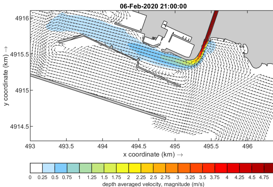
FIGURA 4-10. SOLUZIONE S3 IN FASE B). RISULTATI OTTENUTI ALLA FOCE DEL TORRENTE BISAGNO PER L'EVENTO DI PIENA CON TEMPO DI RITORNO 200 ANNI CON PORTATA AL COLMO Q_{RES} = 750 \text{ M}^3/\text{S} . CAMPO DI VELOCITÀ ALLE ORE 21:00 (COLMO DI PIENA).
