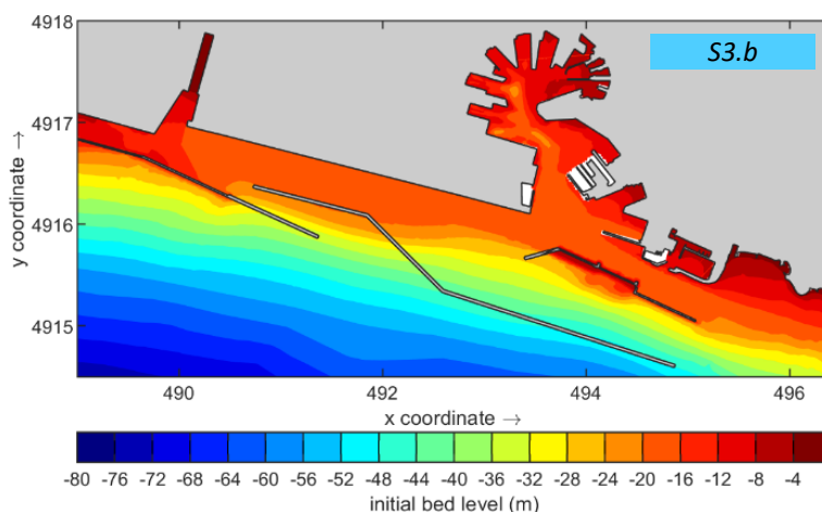
FIGURA 3-28. DOMINIO DI CALCOLO PER LA SOLUZIONE S3 - FASE B.
