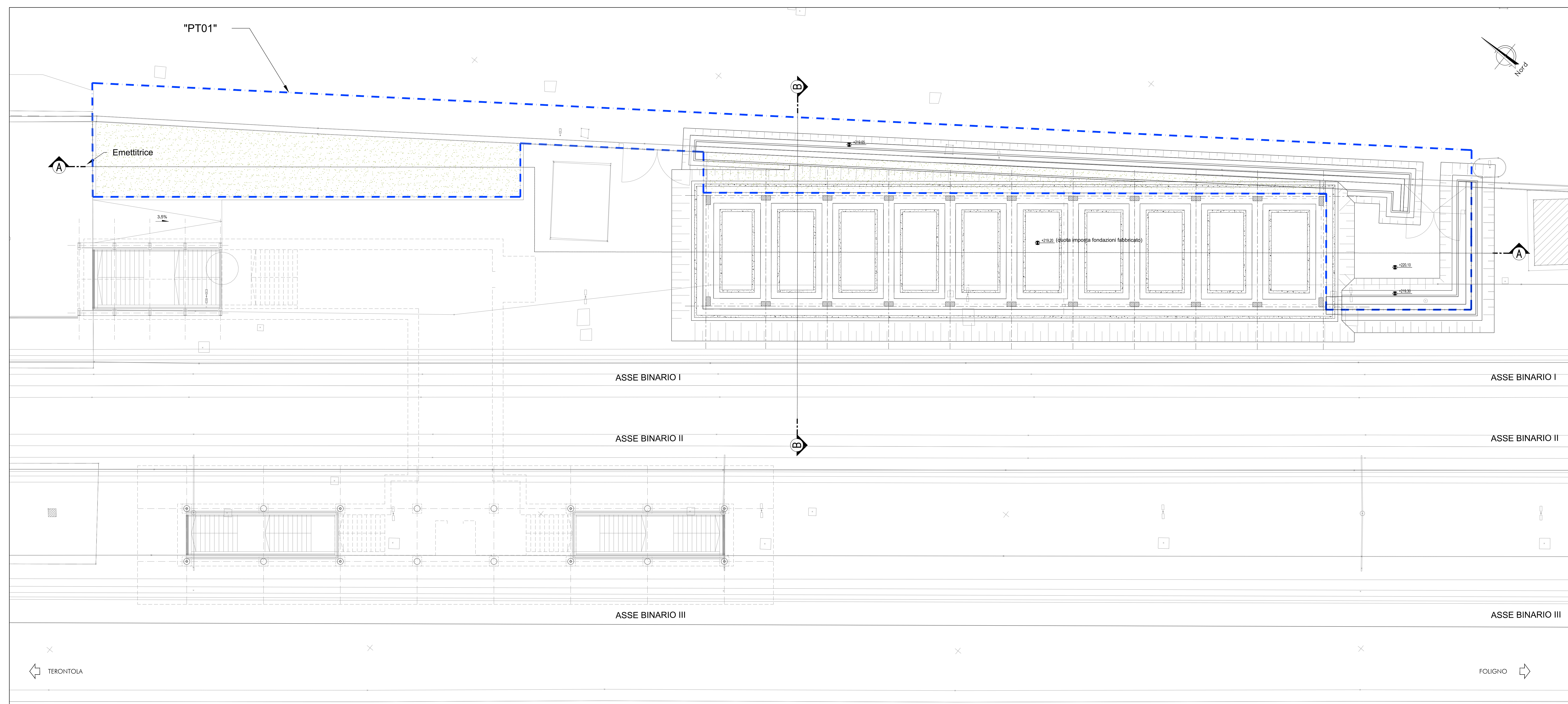
PIAZZALE PLANIMETRIA Scala 1:100
