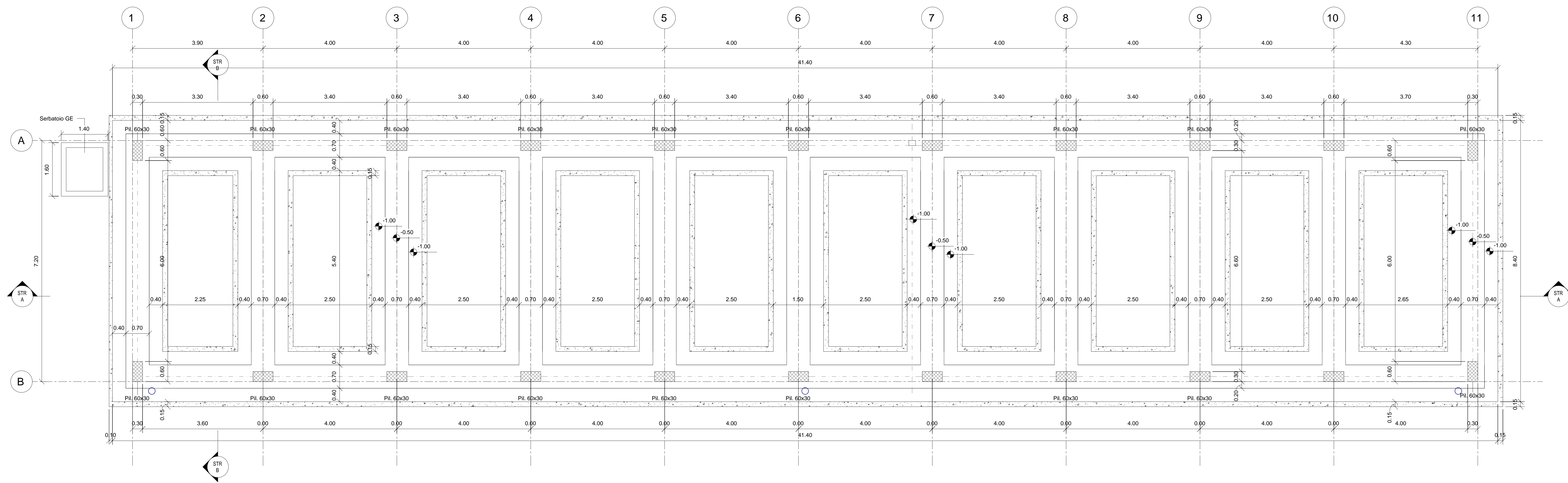
Carpenteria Fondazione 1 : 50
