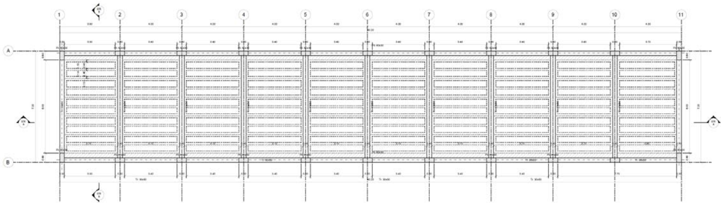
Figura 1 – Carpenteria della copertura
