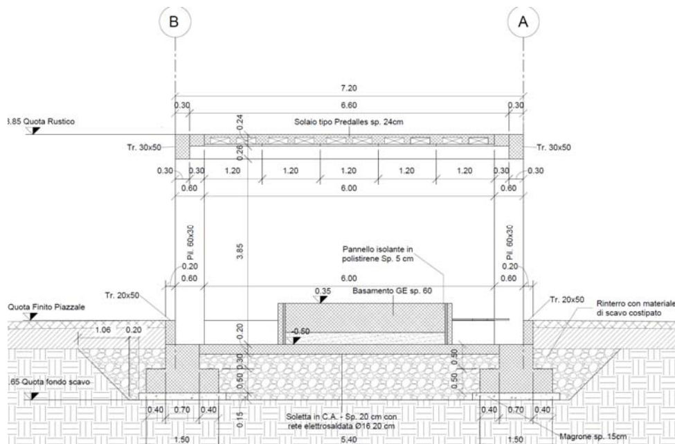
Figura 4 – Sezione trasversale
