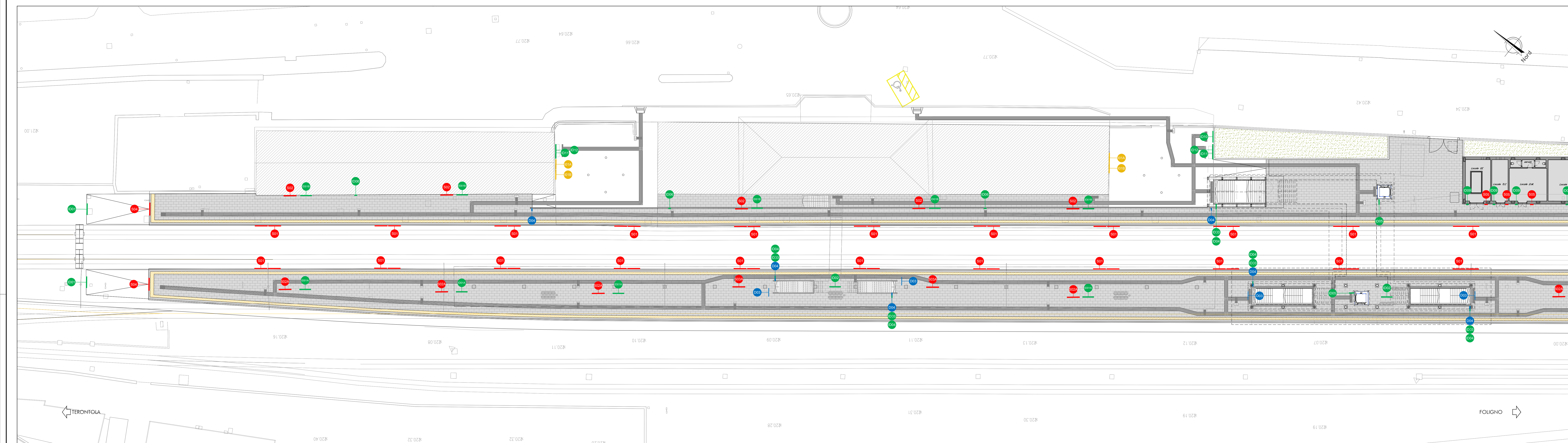
PIANTA QUOTA BANCHINA CON SEGNALETICA A MESSAGGIO FISSO Scala 1:200
