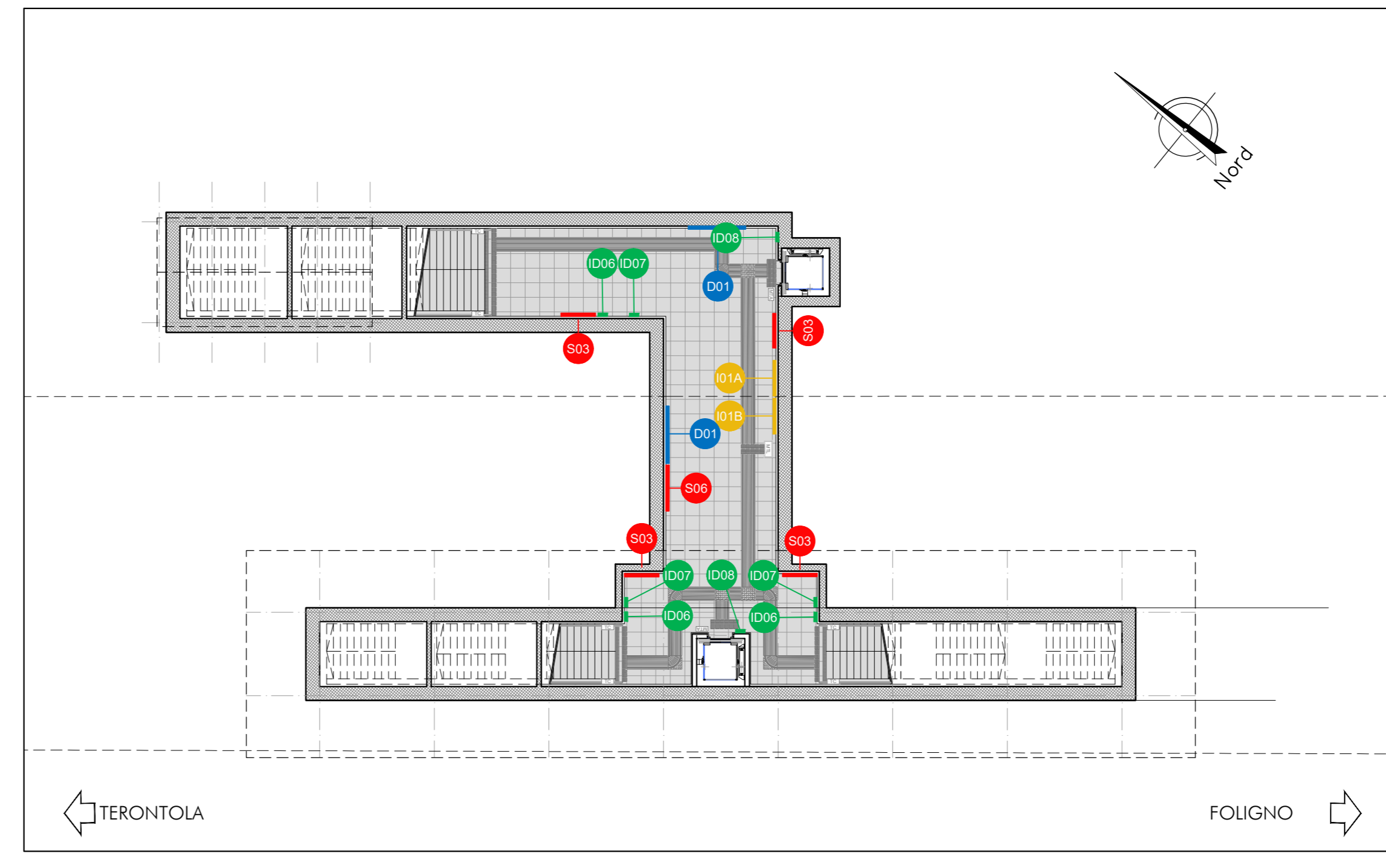
PIANTA QUOTA SOTTOPASSO CON SEGNALETICA A MESSAGGIO FISSO Scala 1:200
