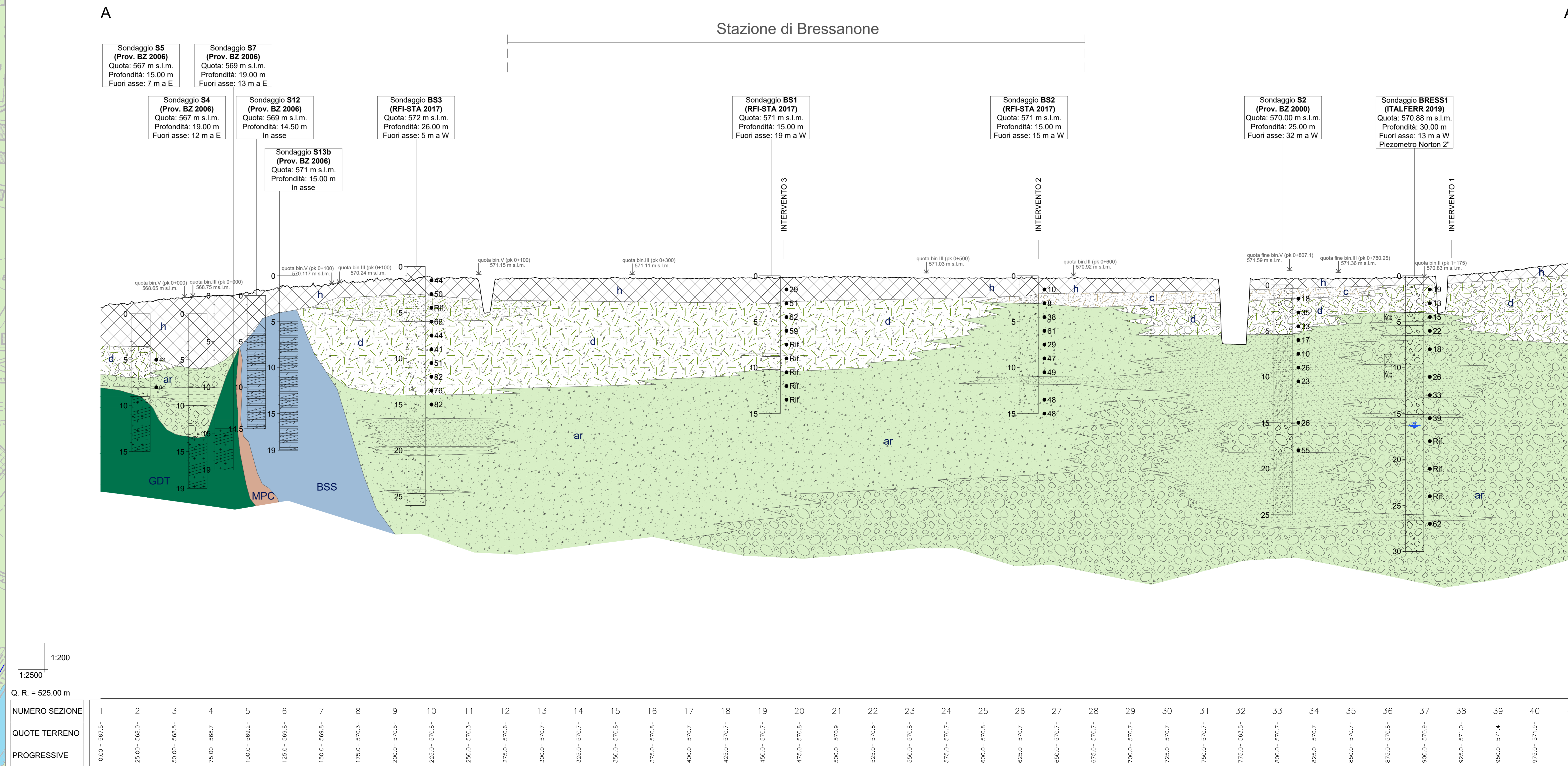
PROFILO GEOLOGICO LONGITUDINALE ALLA STAZIONE FERROVIARIA (SCALA 1:2.500/200)
