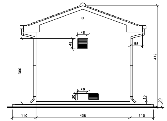
PROSPETTO B
