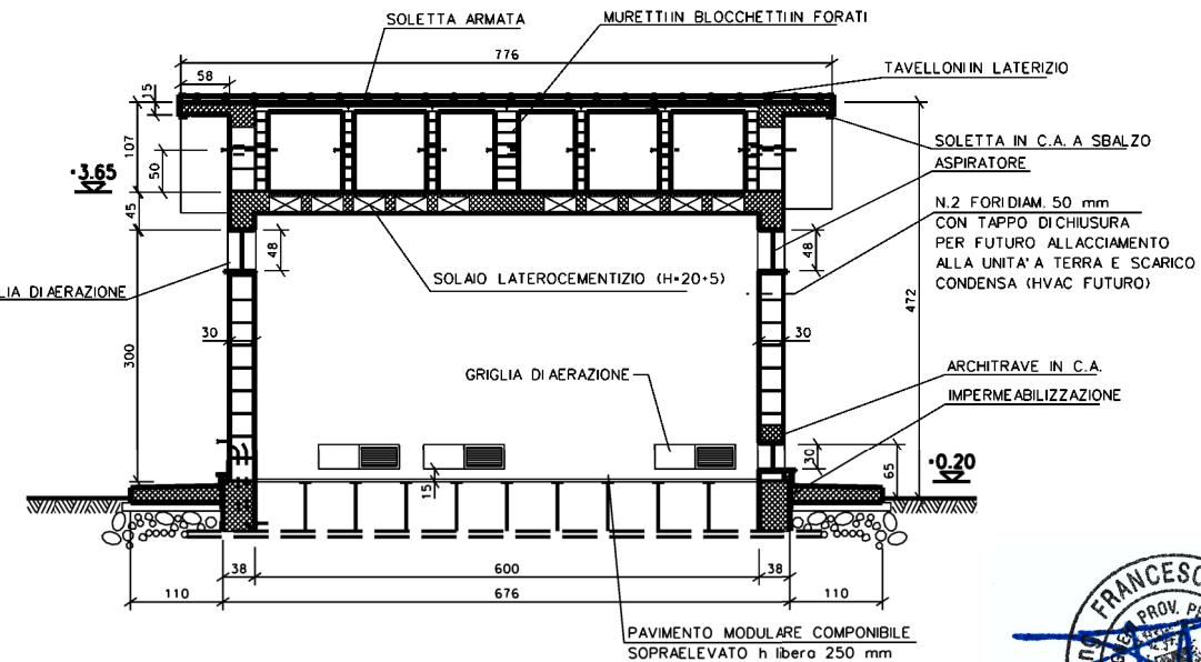
SEZIONE A-A
