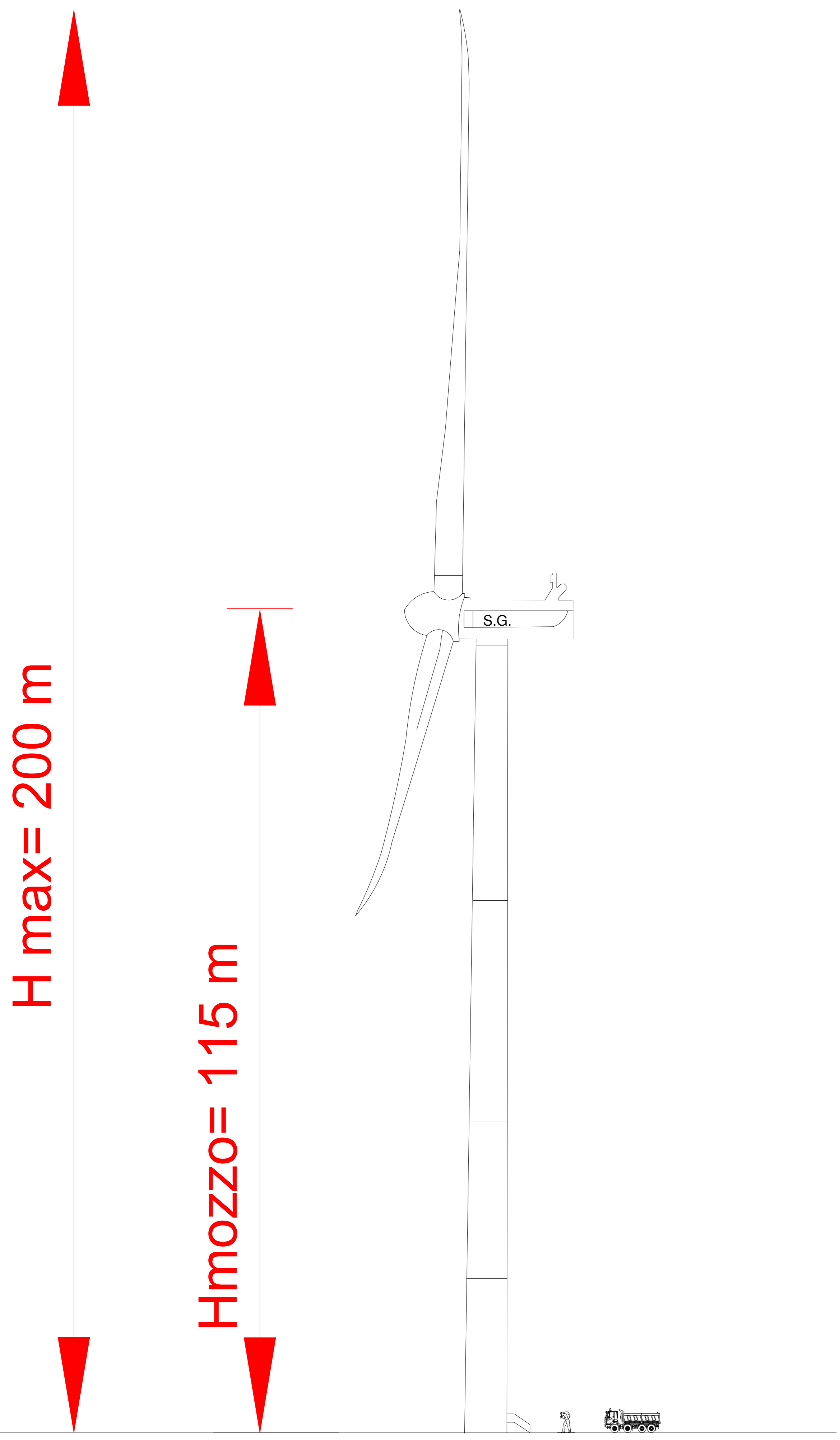
VISTA LATERALE
