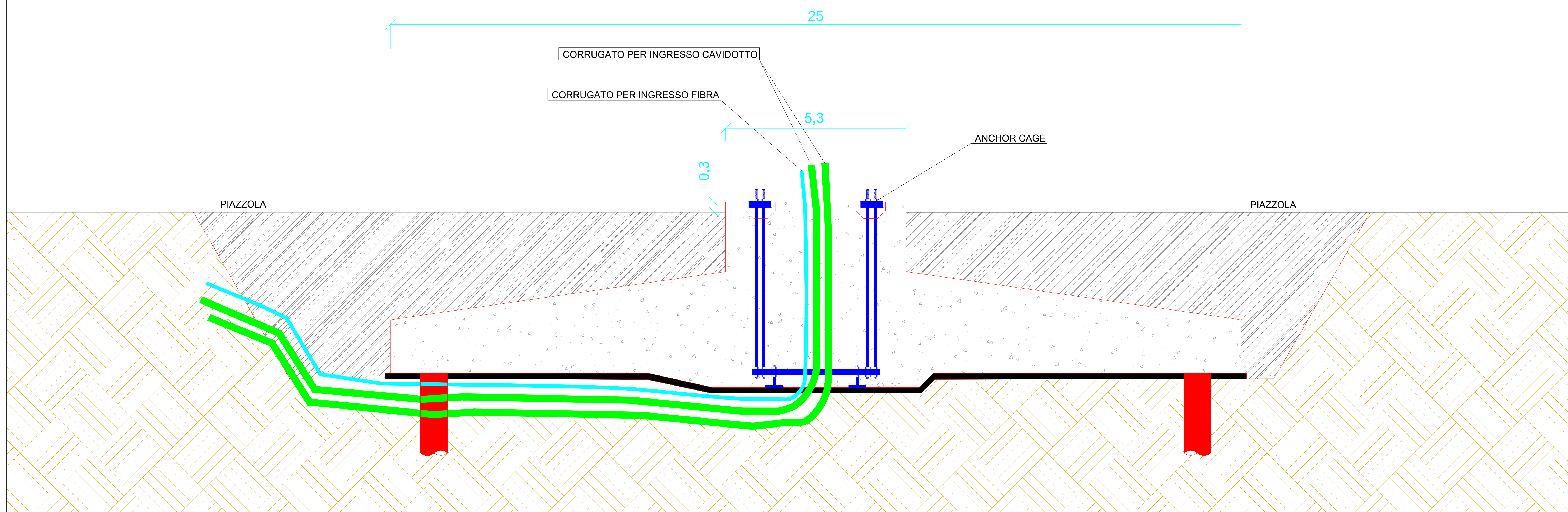
SEZIONE PLINTO DI FONDAZIONE SU PALI
